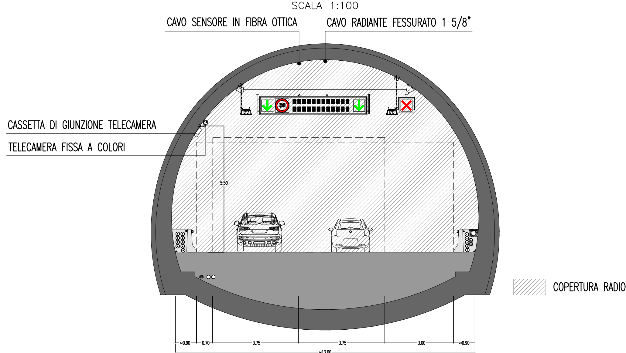
SEZIONE TIPO GALLERIA
