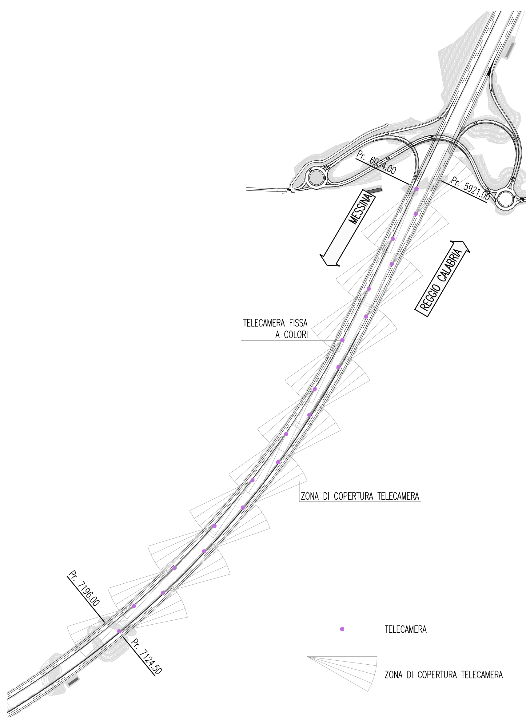
PARTICOLARE ZONA DI COPERTURA E DISPOSIZIONE TELECAMERE
