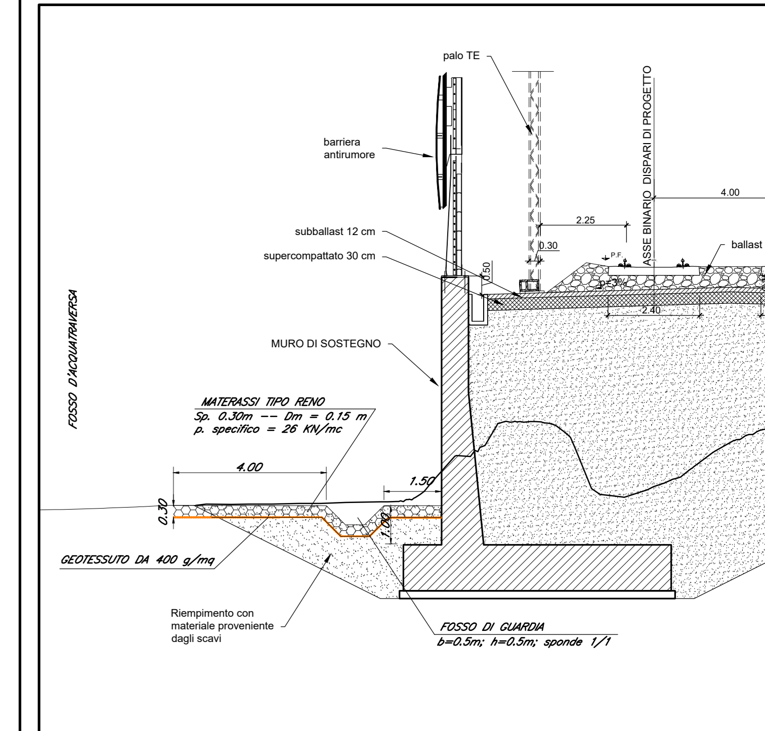
SEZIONE TIPO OPERE DI PROTEZIONE RILEVATO (scala 1:100)
