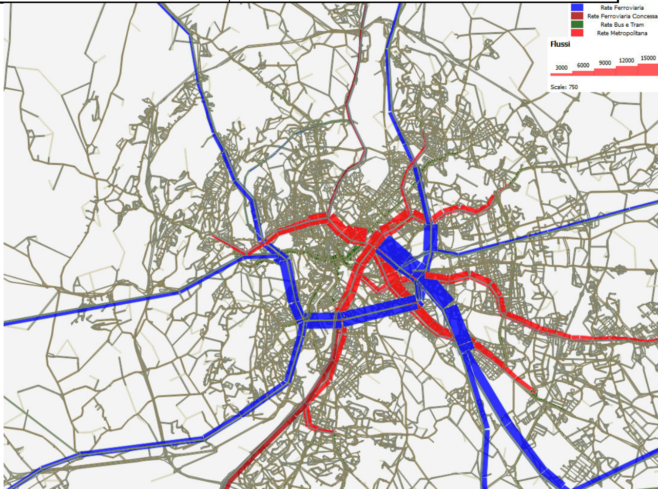
Figura 17. - Tavola 5 - Flussogramma Scenario di Progetto anno 2027
