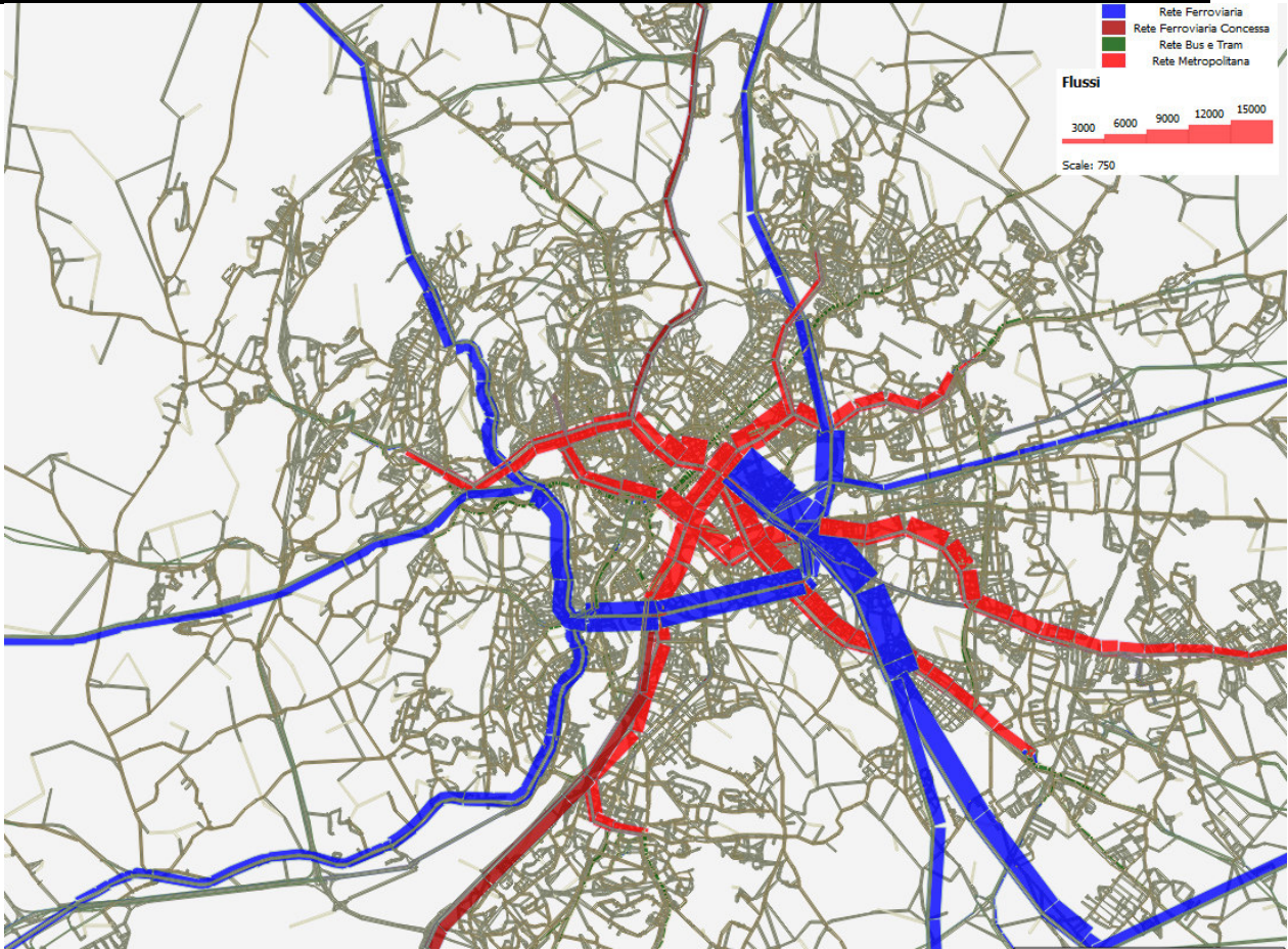
Figura 27. Tavola 10 - Flussogramma scenario di riferimento anno 2051
