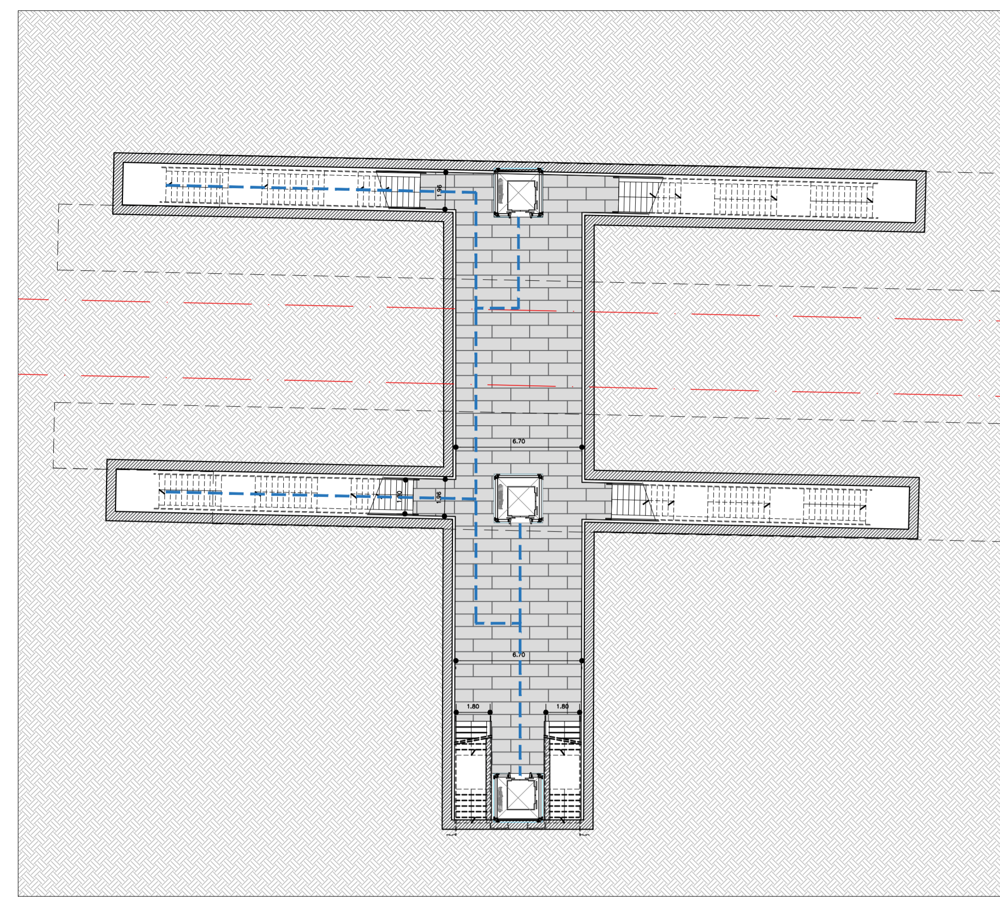
PIANTA SOTTOPASSO ASTRAL scala 1:200
