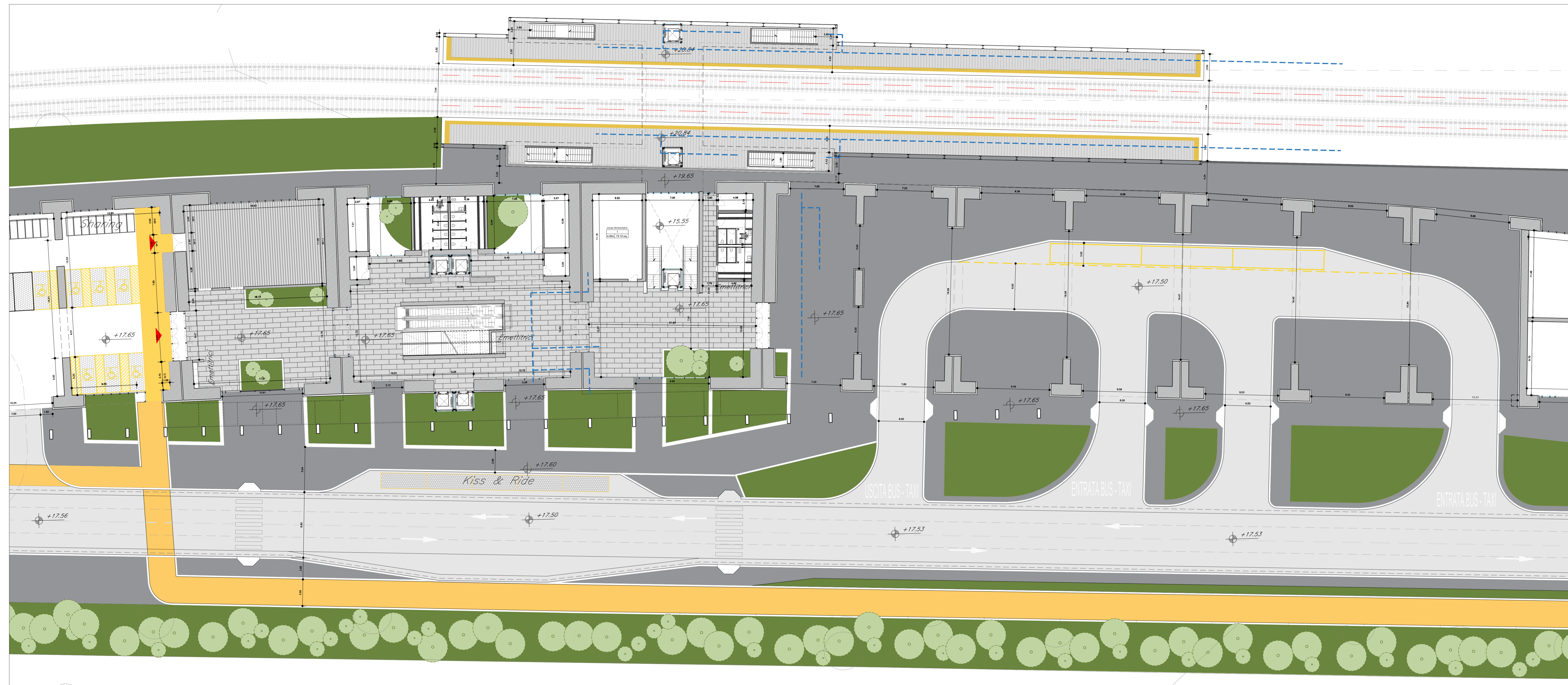
PLANIMETRIA ATRIO RFI - ASTRAL scala 1:200
