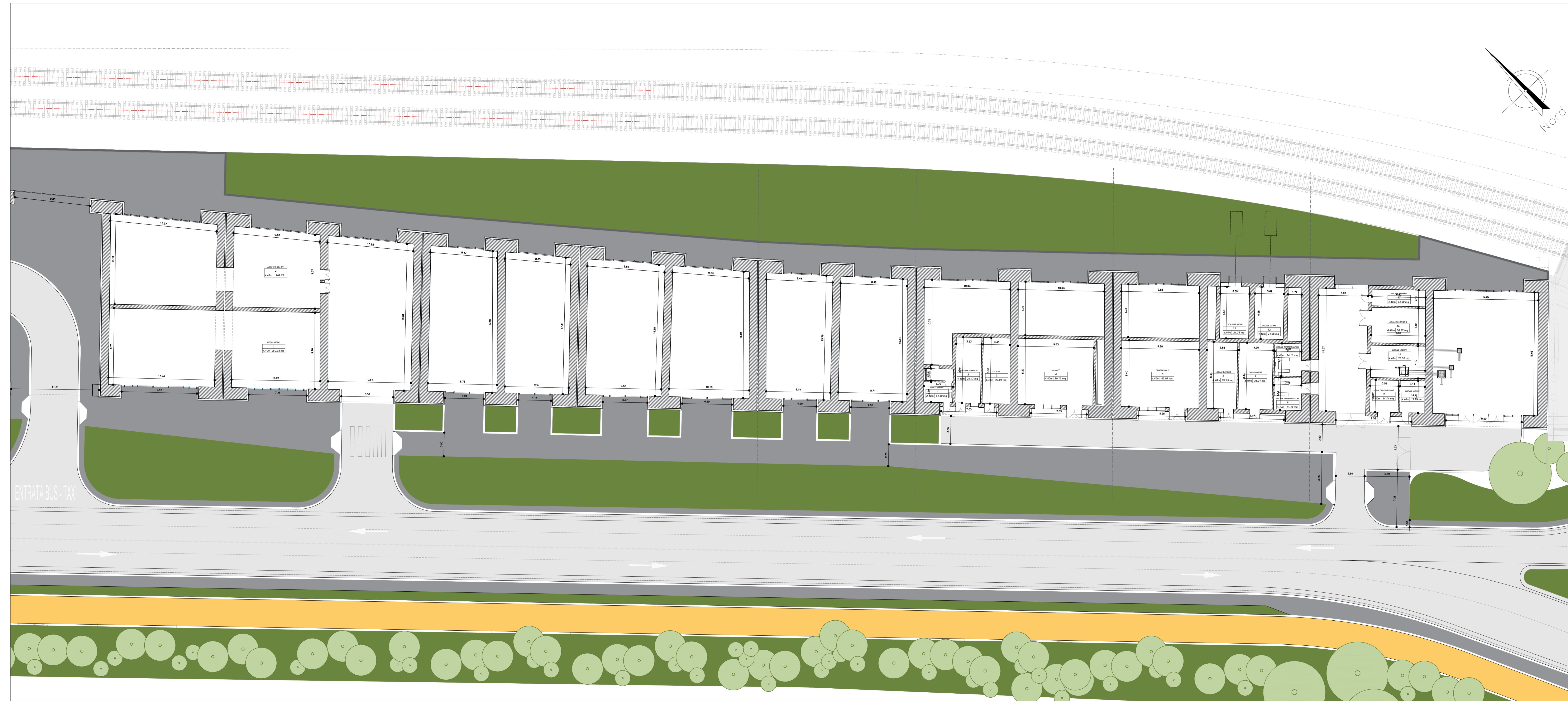
PIANTA AREA TECNOLOGICA scala 1:200
