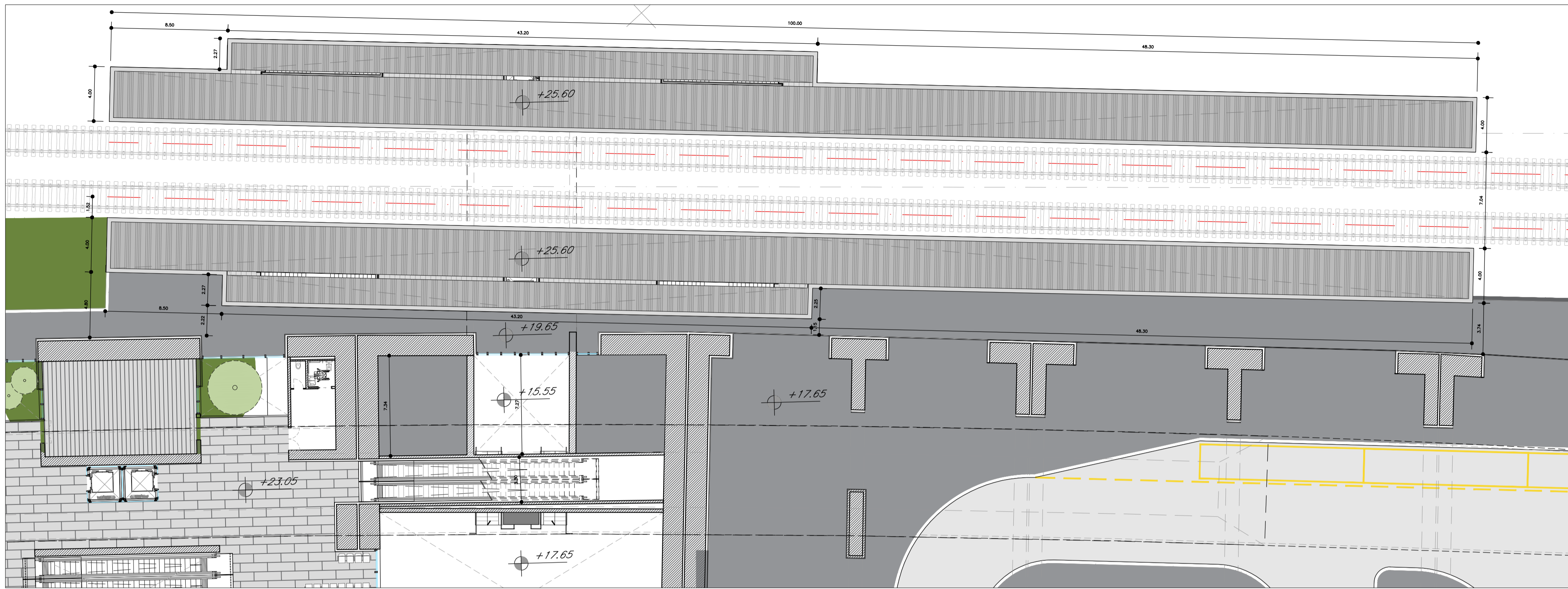
COPERTURA PENSILINA ASTRAL scala 1:200
