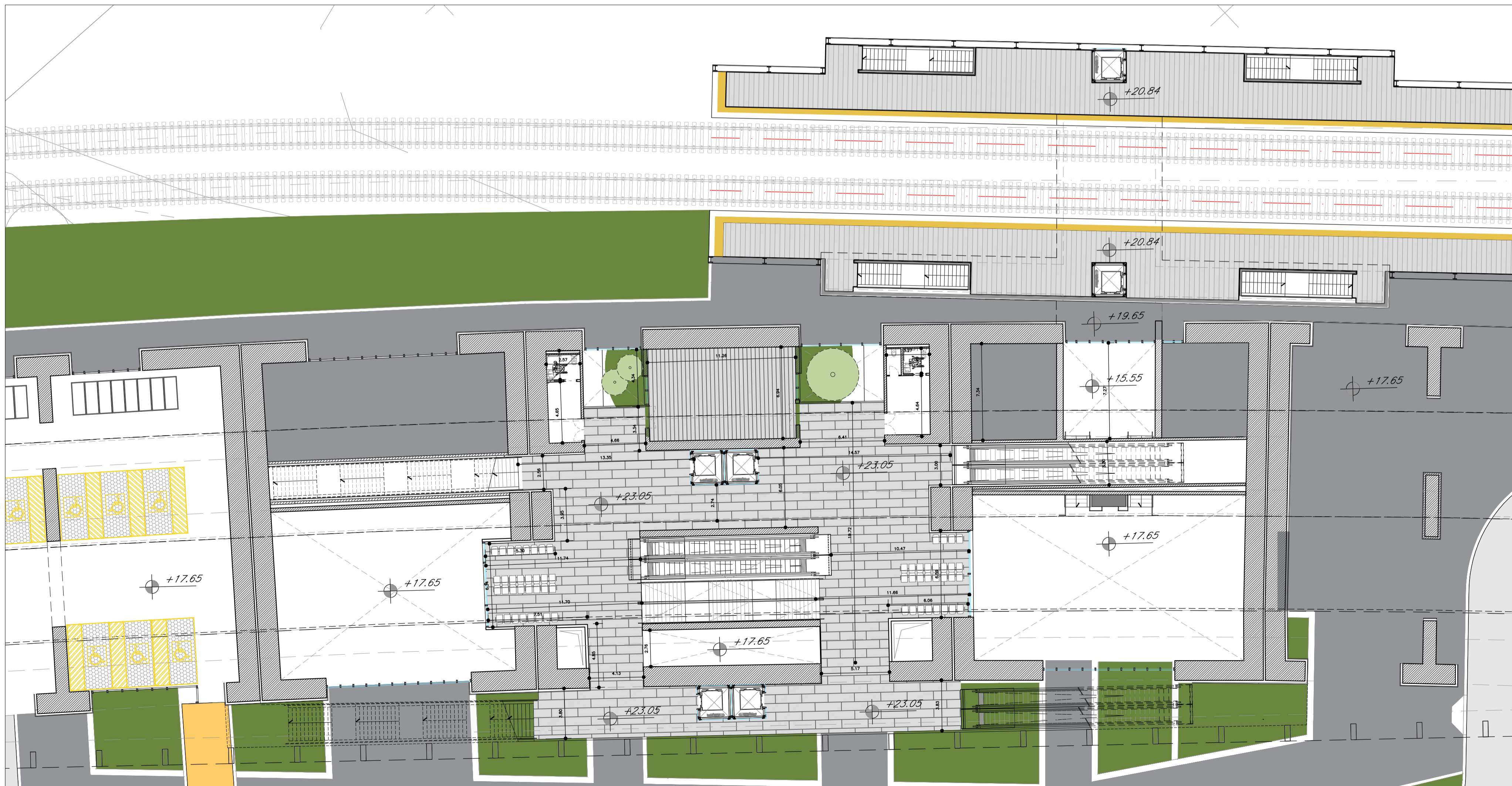
PLANIMETRIA QUOTA MEZZANINO FS scala 1:200
