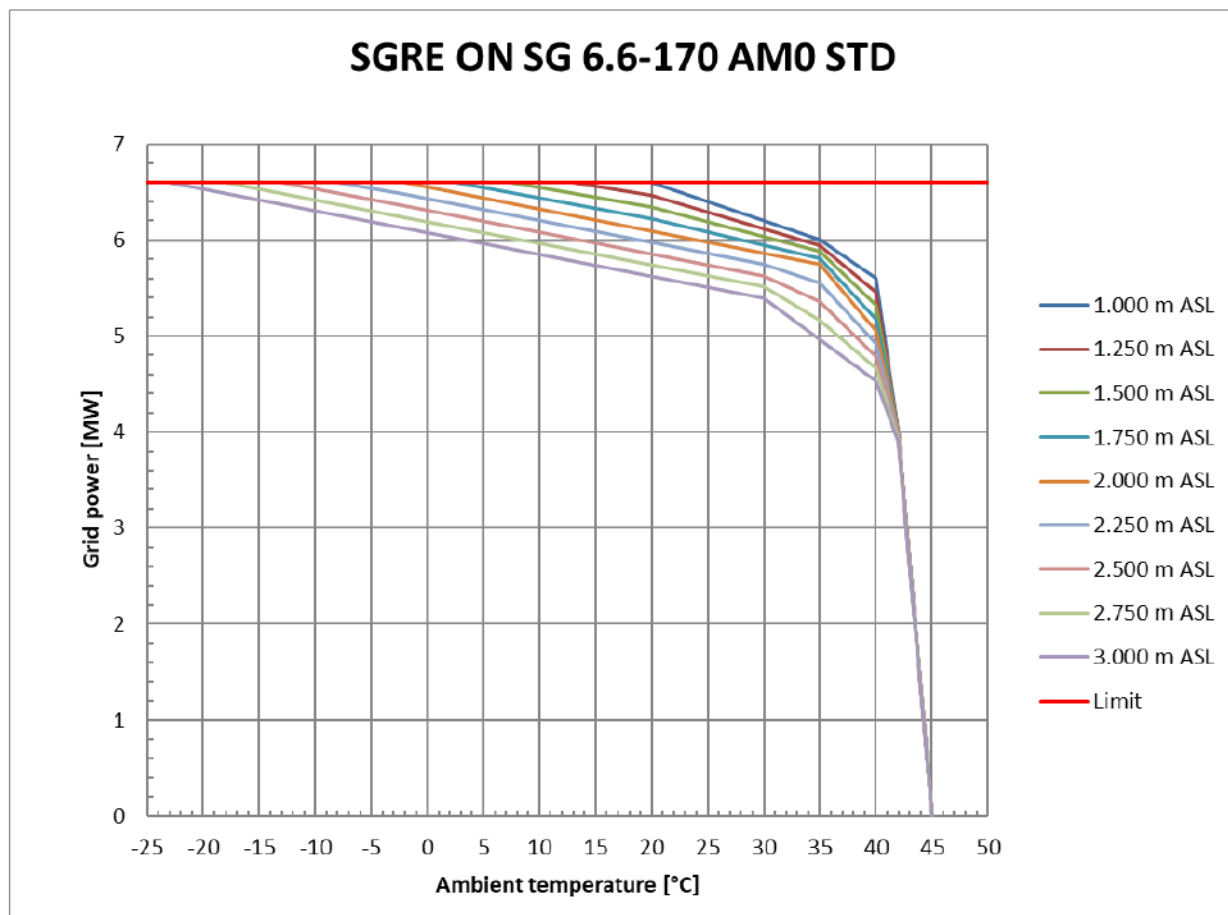
Figura 4 – Funzionamento dipendente dalla temperatura.
