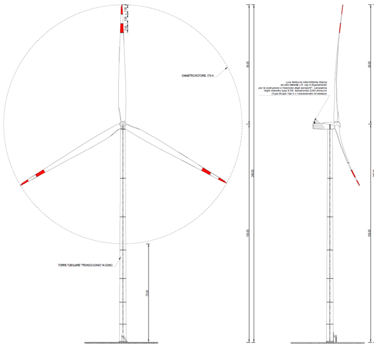
Figura 2 – Vista prospettica e laterale dell'aerogeneratore SIEMENS GAMESA SG 6.6 - 170 da 6,6 MW.
