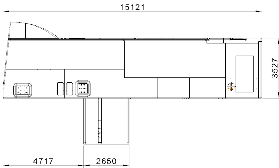
Figura 3 – Dettaglio della navicella dell'aerogeneratore SIEMENS GAMESA SG 6.6 - 170 da 6,6 MW.
