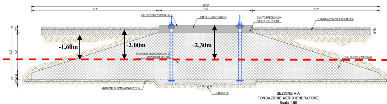
Figura 2 – Schema della dismissione del plinto della fondazione, fino a - 2,0 m dal piano campagna finale di progetto.
