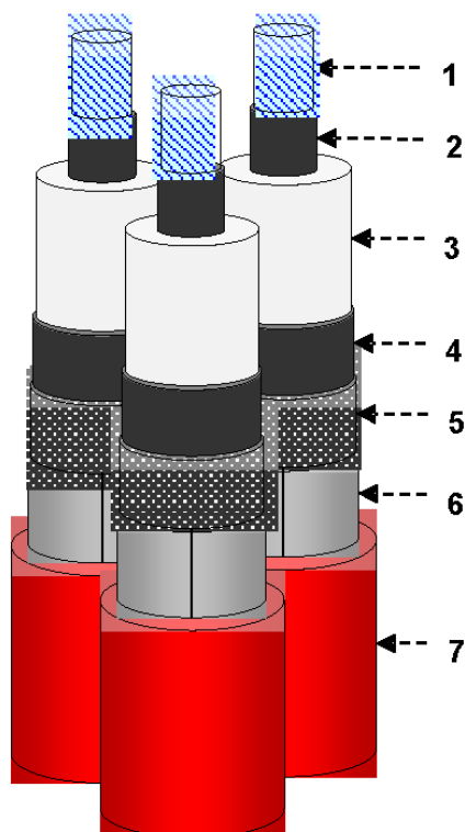
Figura 1 Particolare cavo MT
