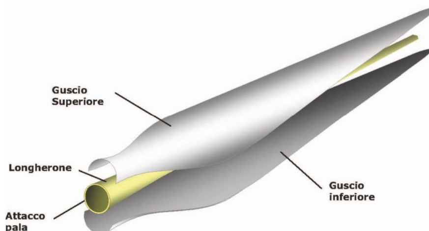
Figura 1 - Schema strutturale di una pala eolica.
