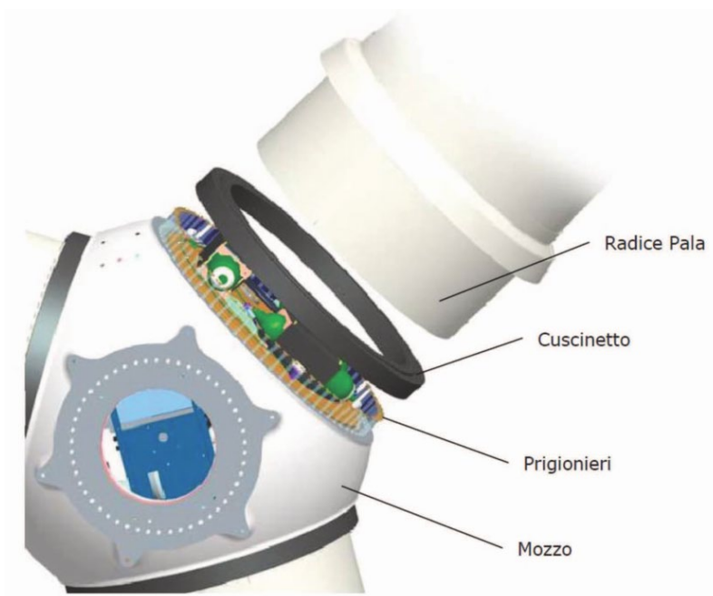
Figura 2 - Schema strutturale di collegamento elemento pala – mozzo.
