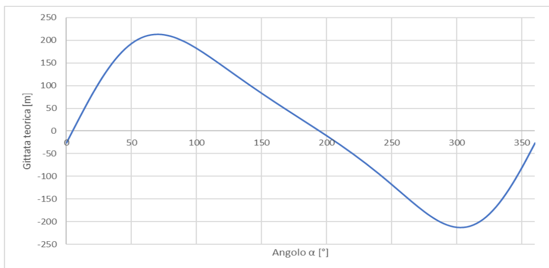
Figura 4 – Calcolo della gittata in funzione dell'angolo \alpha sotteso dalla pala (posizione della pala al momento della rottura).
