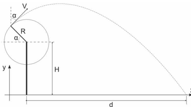
Figura 3 – Schema della traiettoria della pala in caduta.
