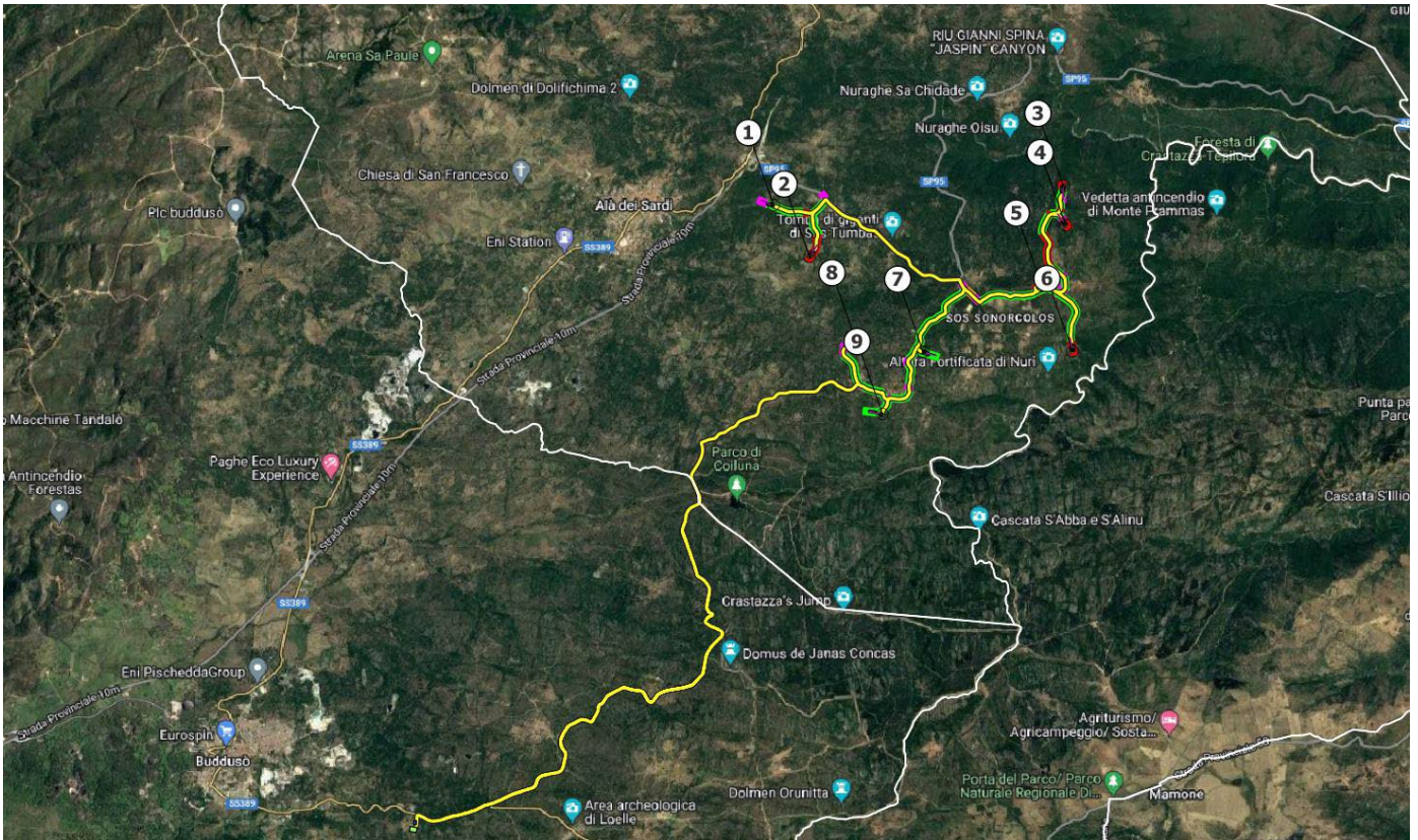
Figura 1 Layout di Impianto su ortofoto
