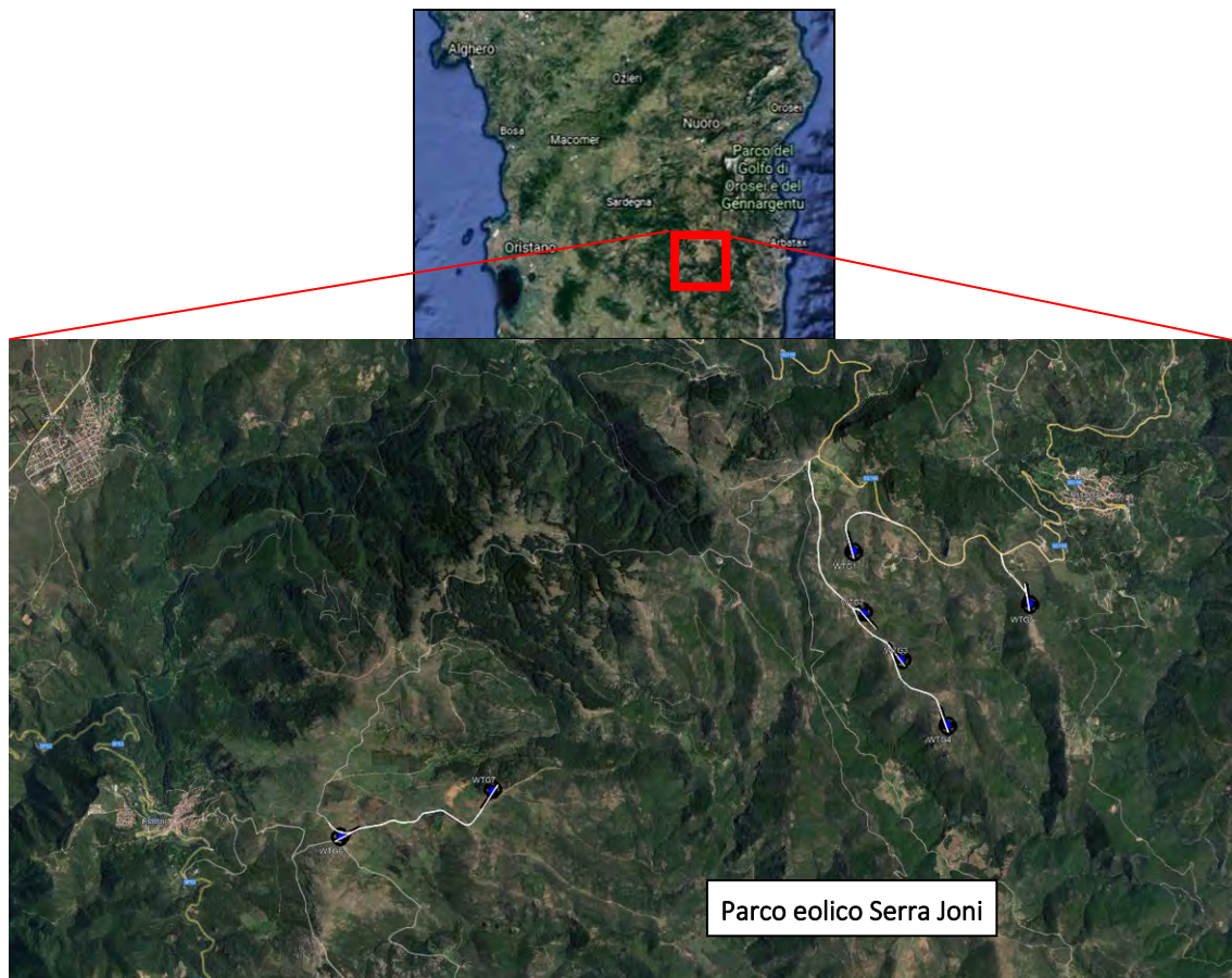
Figura 1 – Inquadramento territoriale generale e vista aerea delle posizioni degli aerogeneratori del parco eolico "Serra Joni" nei comuni di Ussassai e Esterzili e viabilità interna al parco.
