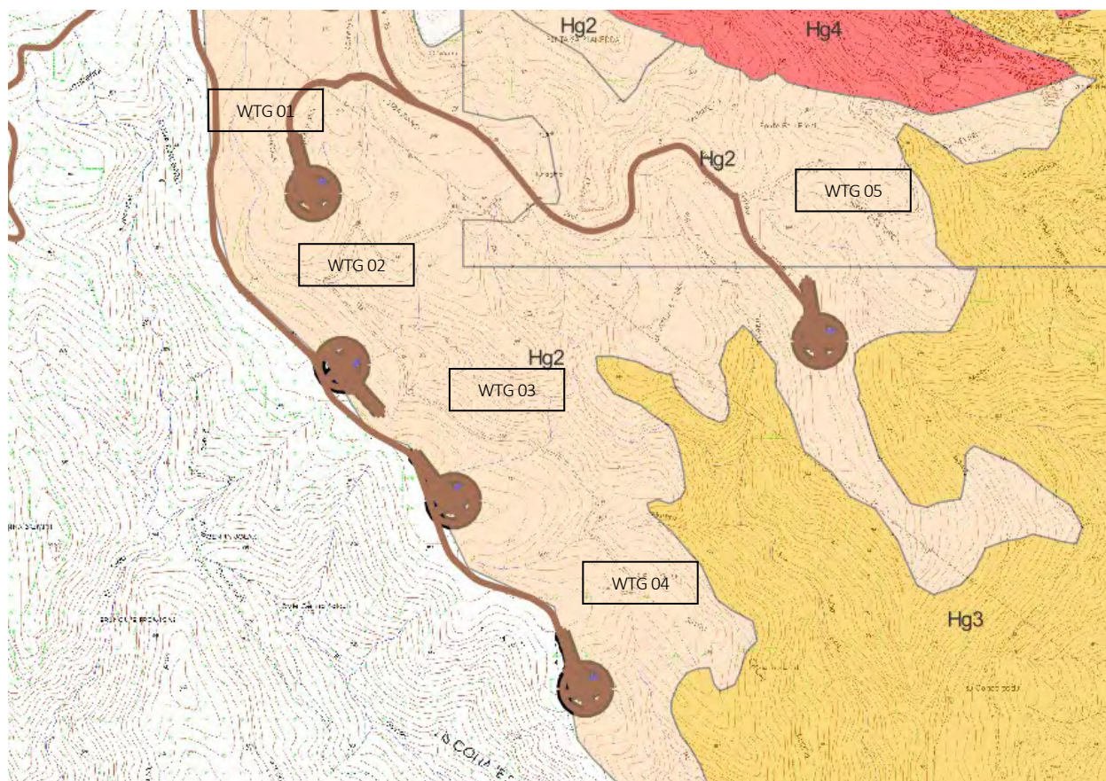
Figura 2 – Particolare dell'ubicazione degli aerogeneratori WTG 1, 2, 3, 4 e 5 su planimetria PAI frana, ricadenti in area Hg 2.
