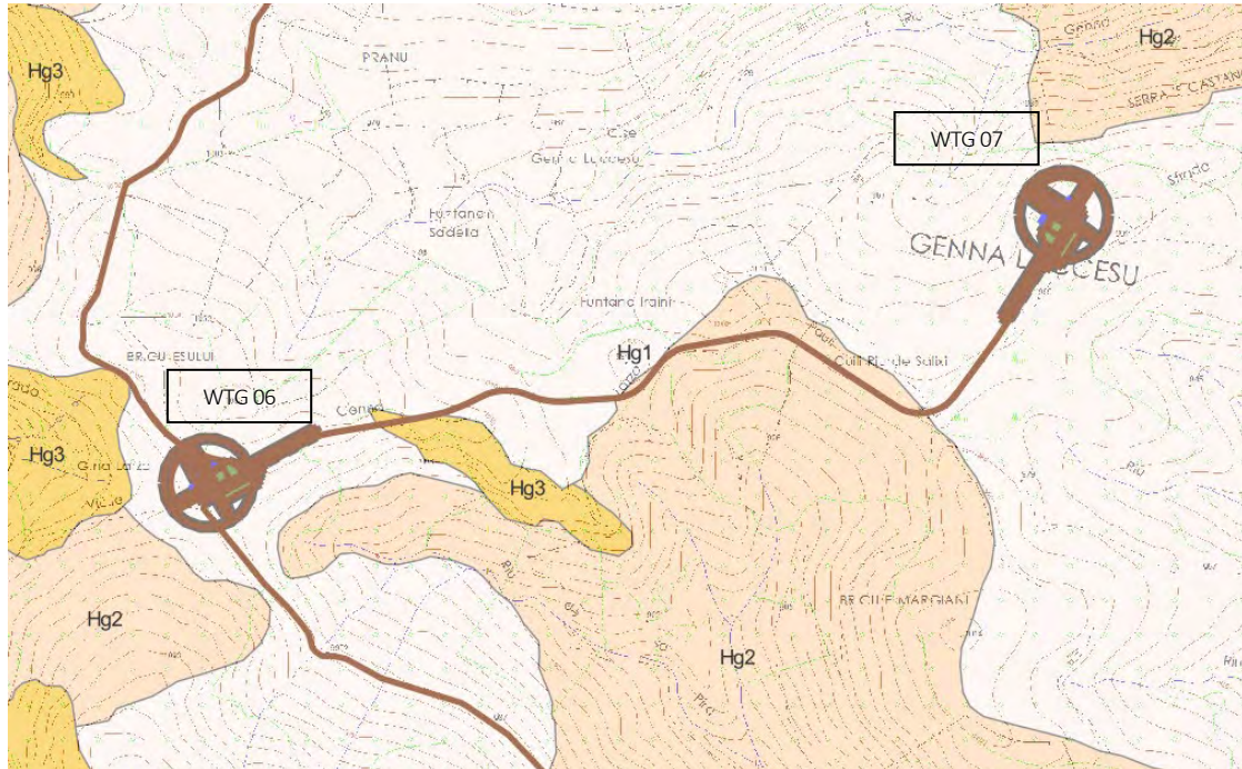
Figura 3 - Particolare dell'ubicazione degli aerogeneratori WTG 6 e 7 su planimetria PAI frana, ricadenti in area Hg 1.
