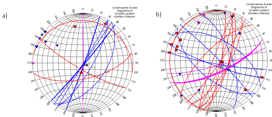
Figura 6 – Proiezioni stereografiche dei piani di frattura rilevati nel settore est (a - Comune di Ussassai) e ovest (b - Comune di Esterzili) del parco.
