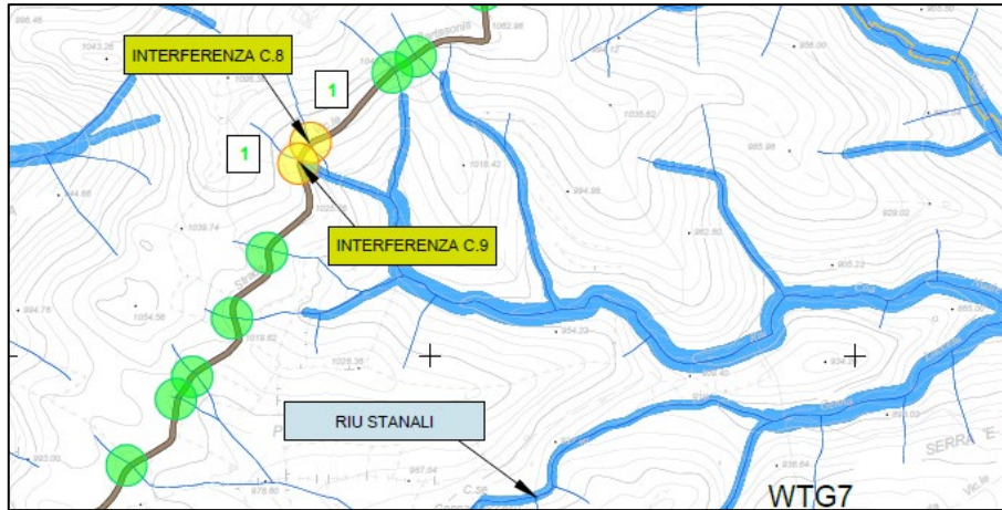
Figura 8 - Interferenze con la rete idrografica lungo il tracciato del cavidotto in progetto.
