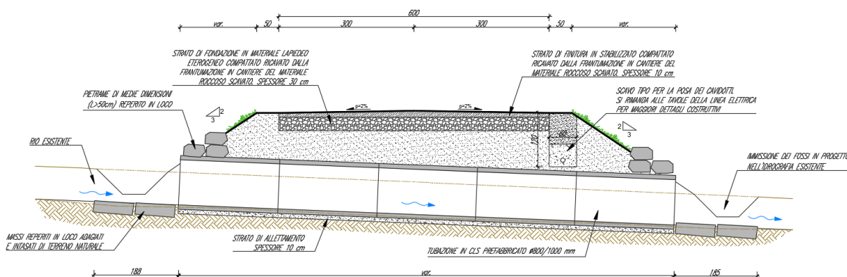
Figura 16 – Sezione tipologica relativa agli interventi di realizzazione di nuova viabilità.
