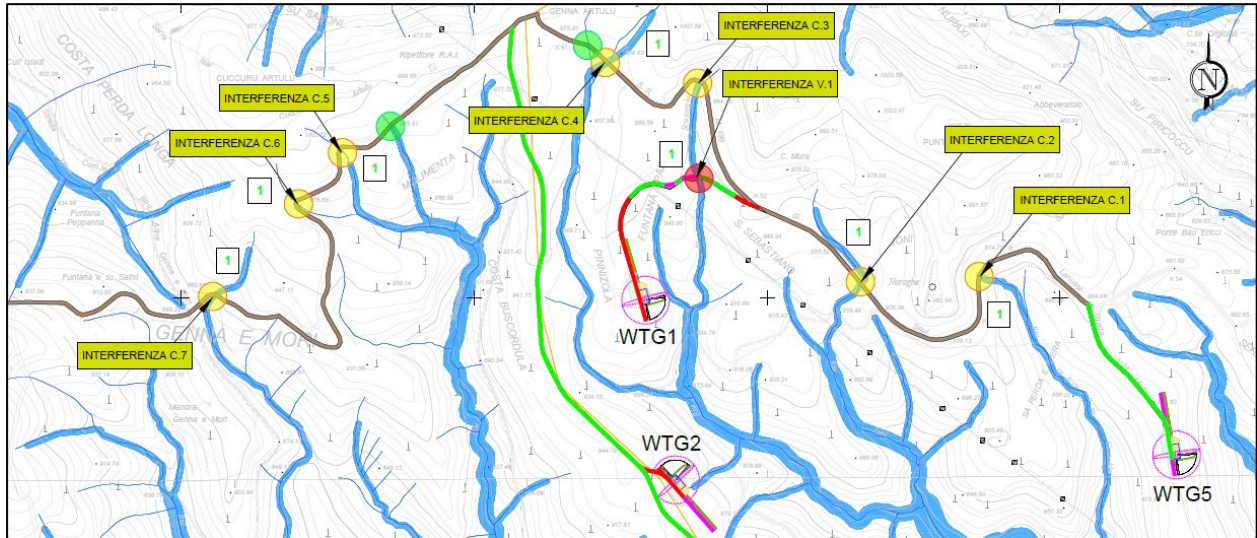
Figura 7 – Interferenze con la rete idrografica lungo il tracciato del cavidotto e la viabilità in progetto.
