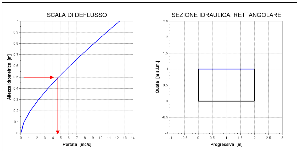
Figura 17 – Scale di deflusso di moto uniforme per gli elementi scatolari di dimensioni 2,5 x 1,5 m e 5,0 x 1,5 m.
