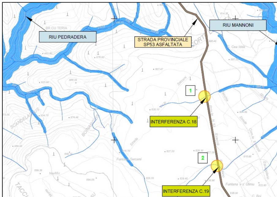
Figura 11 - Interferenze con la rete idrografica lungo il tracciato del cavidotto in progetto.
