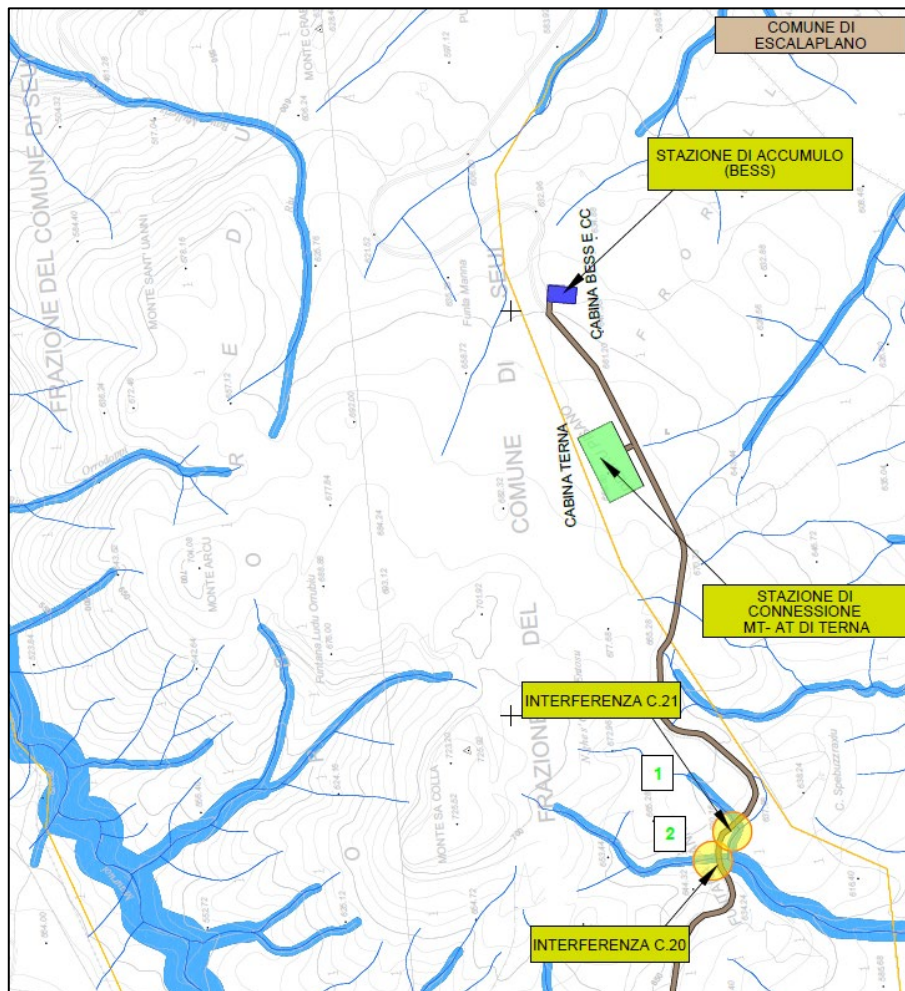
Figura 12 – Interferenze con la rete idrografica lungo il tracciato del cavidotto in progetto.
