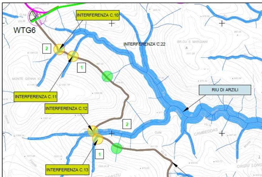
Figura 9 - Interferenze con la rete idrografica lungo il tracciato del cavidotto in progetto.
