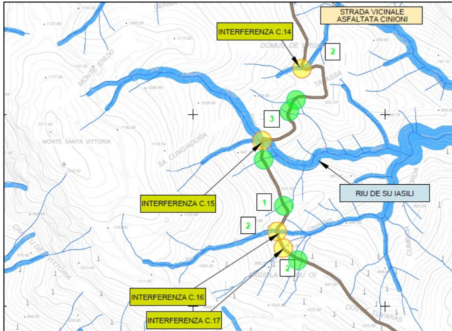
Figura 10 - Interferenze con la rete idrografica lungo il tracciato del cavidotto in progetto.
