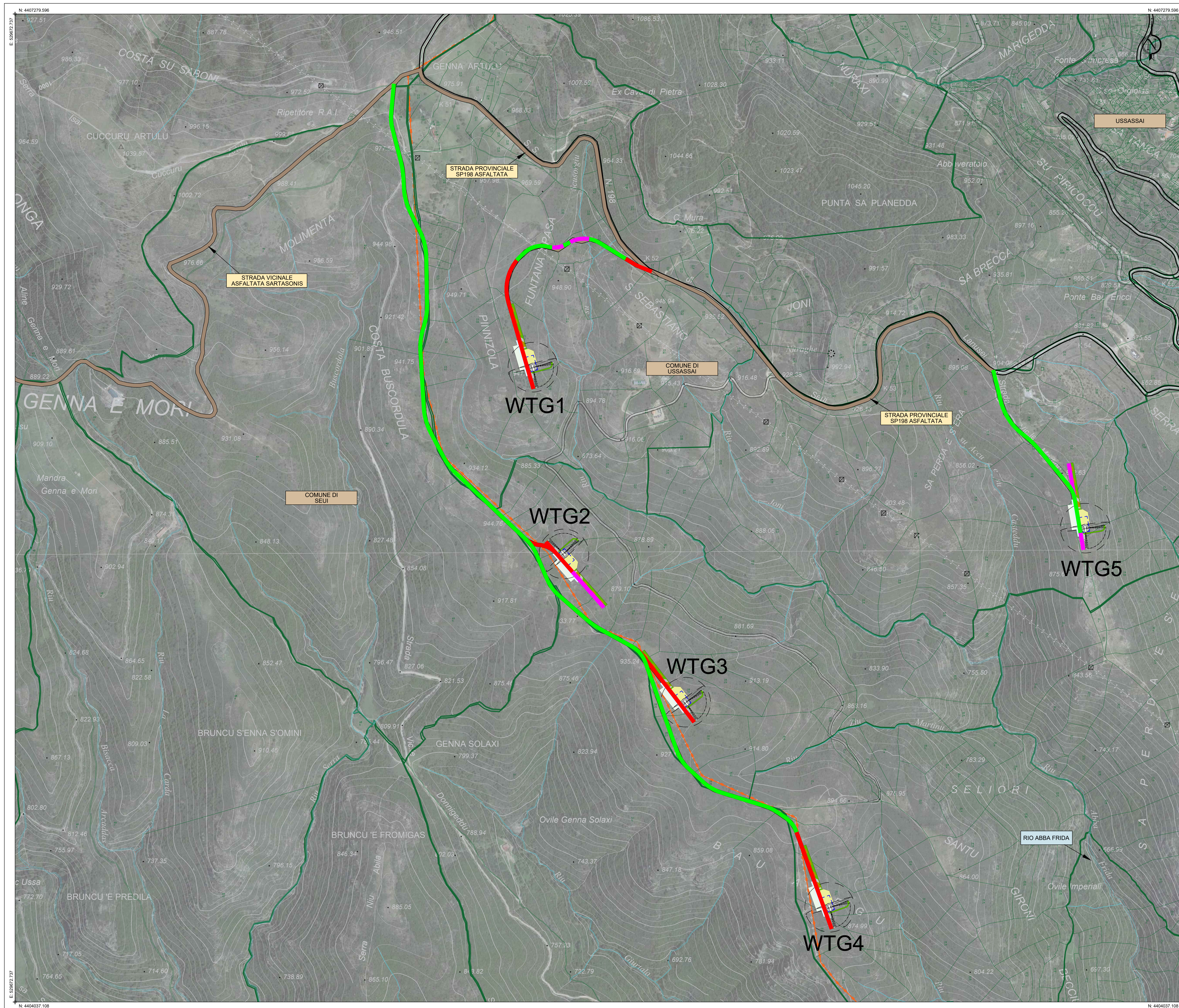
PLANIMETRIA SU BASE C.T.R. VETTORIALE E CATASTALE: TAVOLA A Base carta: Carta Tecnica Regionale 1:10.000 e Ortofoto Google Map
