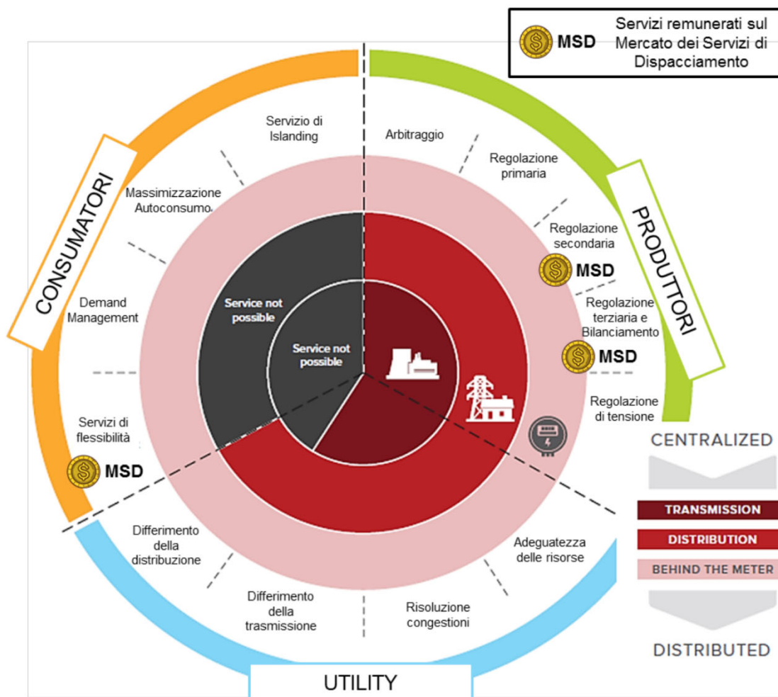
Figura 2 | diversi servizi erogabili dai sistemi Storage
