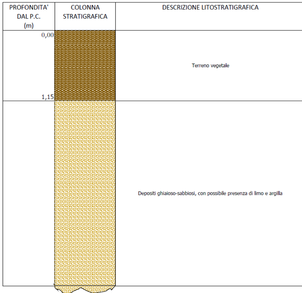
Fig. 6 - COLONNA STRATIGRAFICA
