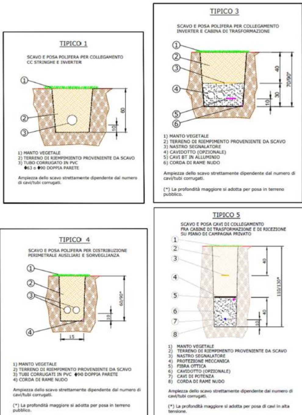
Fig. 7 – Tipici scavi e posa cavi
