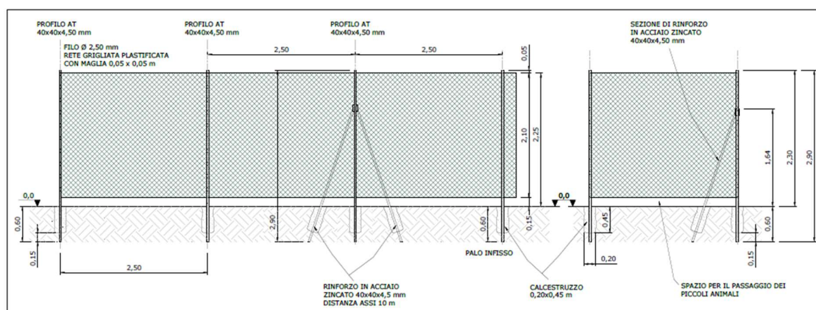
Fig. 14 – Recinzione perimetrale
