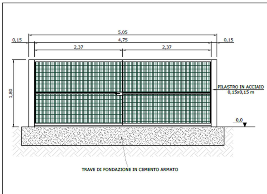
Fig. 15 – Cancello a doppia anta
