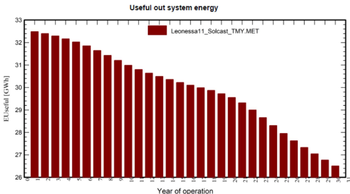
Fig. 28 – Producibilità dell’impianto con degrado moduli (30 anni)
