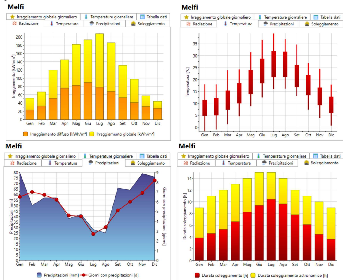
Fig. 23 – Dati di radiazione, temperatura, precipitazioni e soleggiamento
