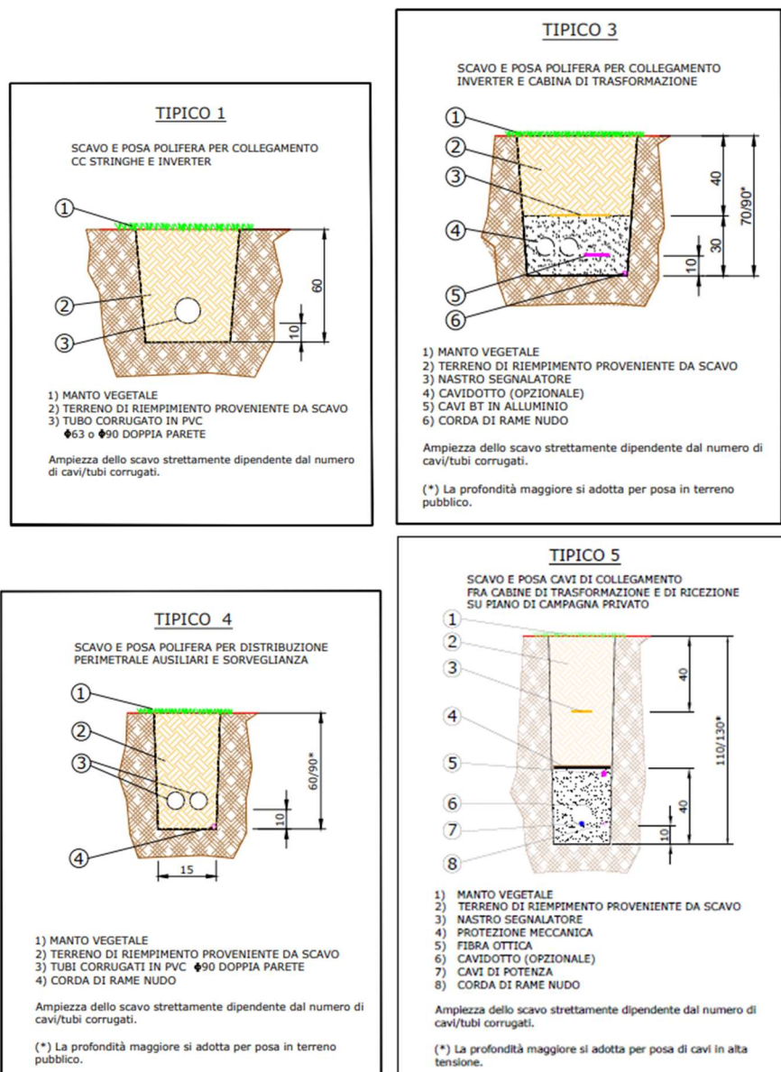
Fig. 17 – Tipici scavi e posa cavi
