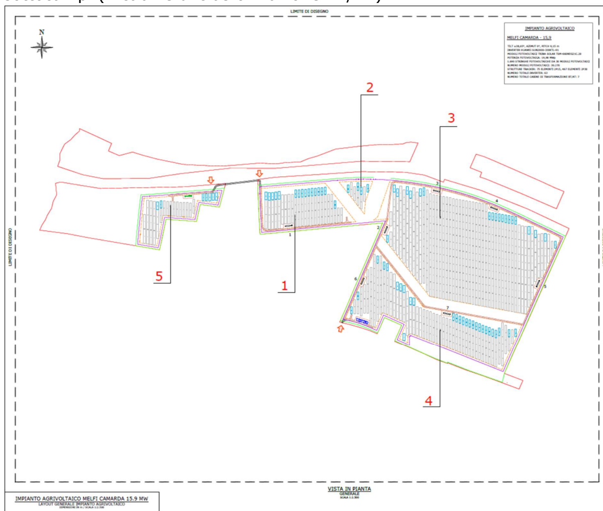
Fig. 6 - Layout di impianto
