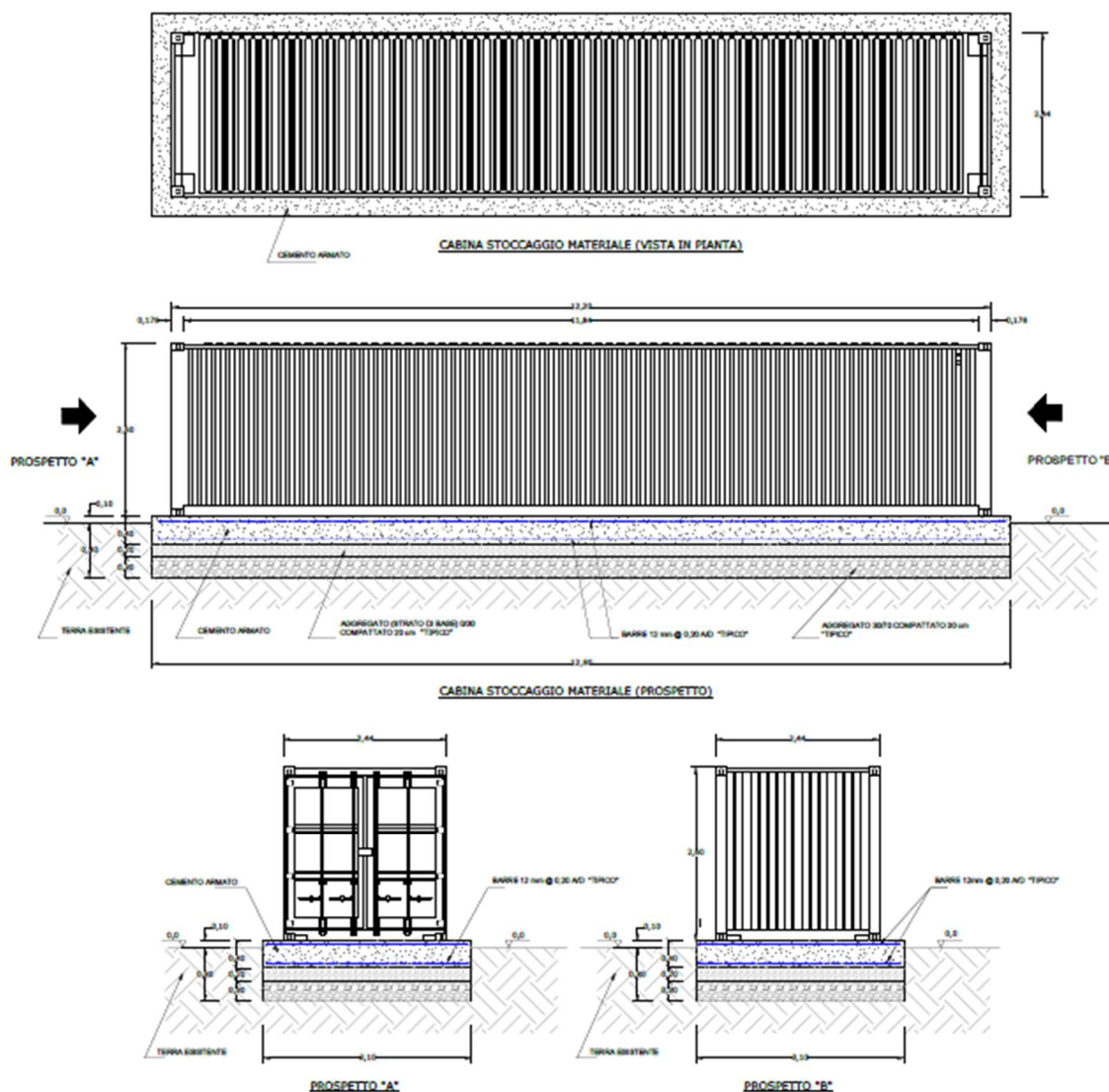
Fig. 20 - Cabina stoccaggio materiale
