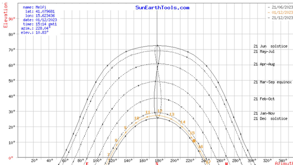
Fig. 25 - Diagramma Solare Polare (Melfi Camarda 15.9)
