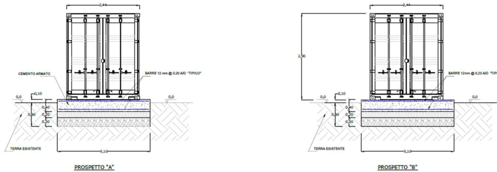
Fig. 18 - Cabina di trasformazione BT/AT
