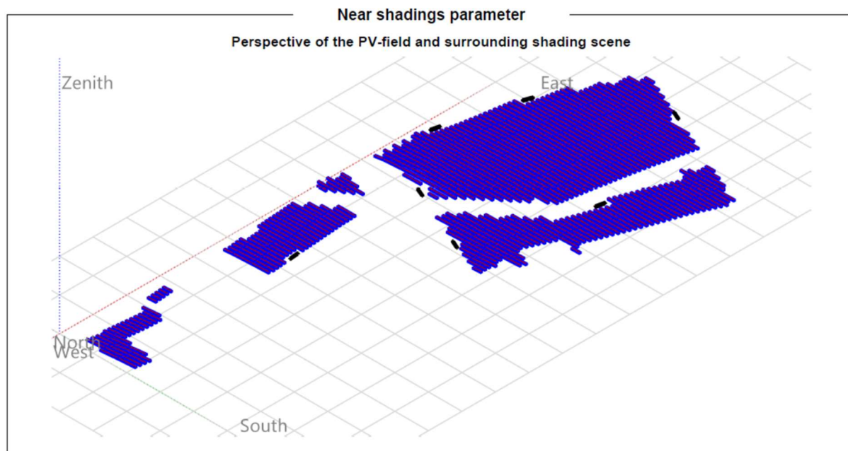
Fig. 26 – Modello 3D dell’impianto
