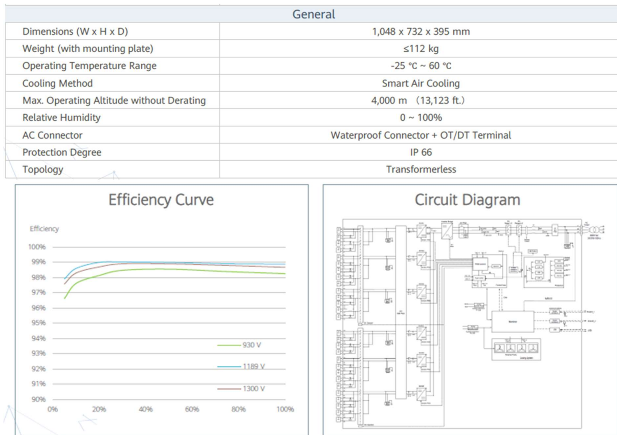
Fig. 12 - Dimensioni, specifiche tecniche e prestazionali dell'inverter
