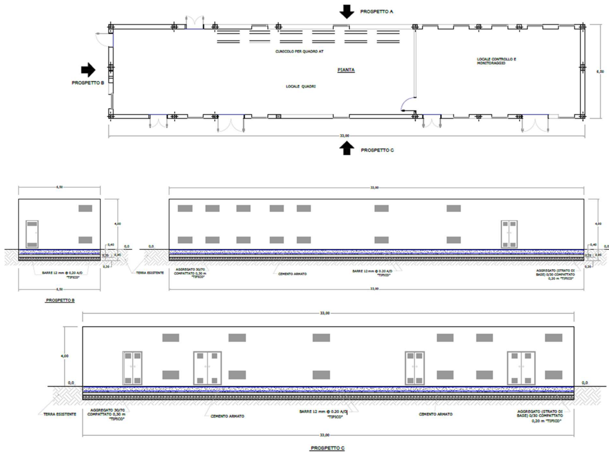
Fig. 19 - Cabina di ricezione, sezionamento e controllo
