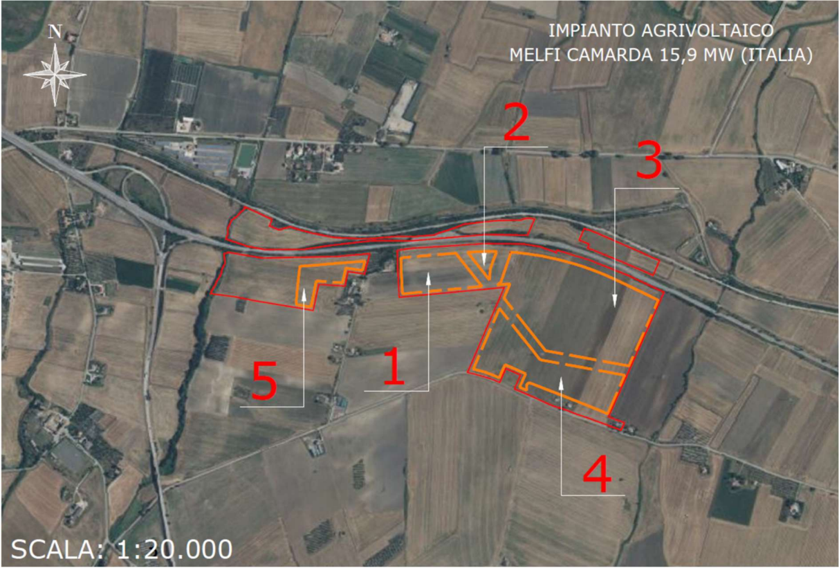
Fig. 5 – Individuazione dell’area di intervento su foto satellitare
