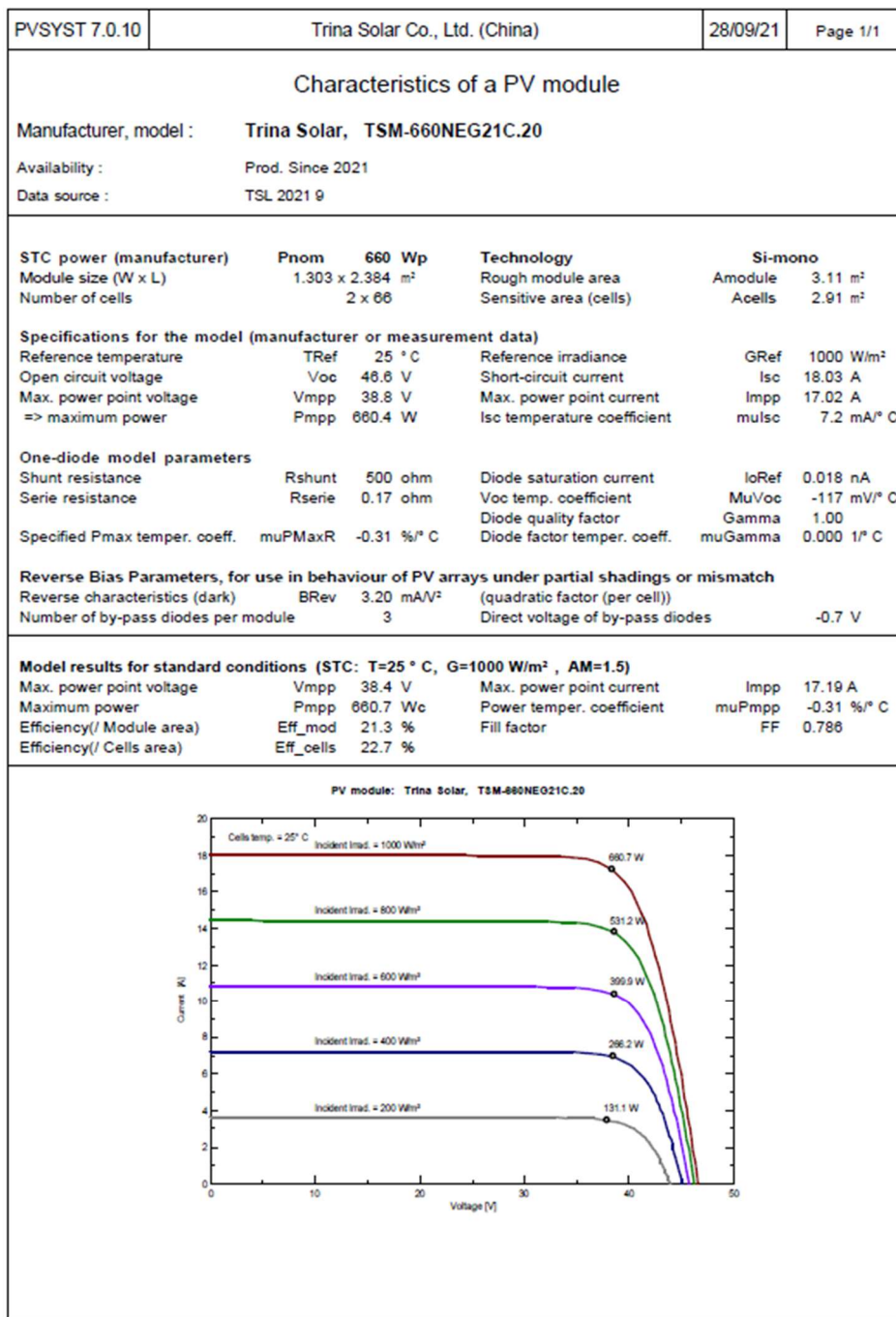
Fig. 7 - Dimensioni, specifiche tecniche e prestazionali pannelli fotovoltaici Trina Solar
