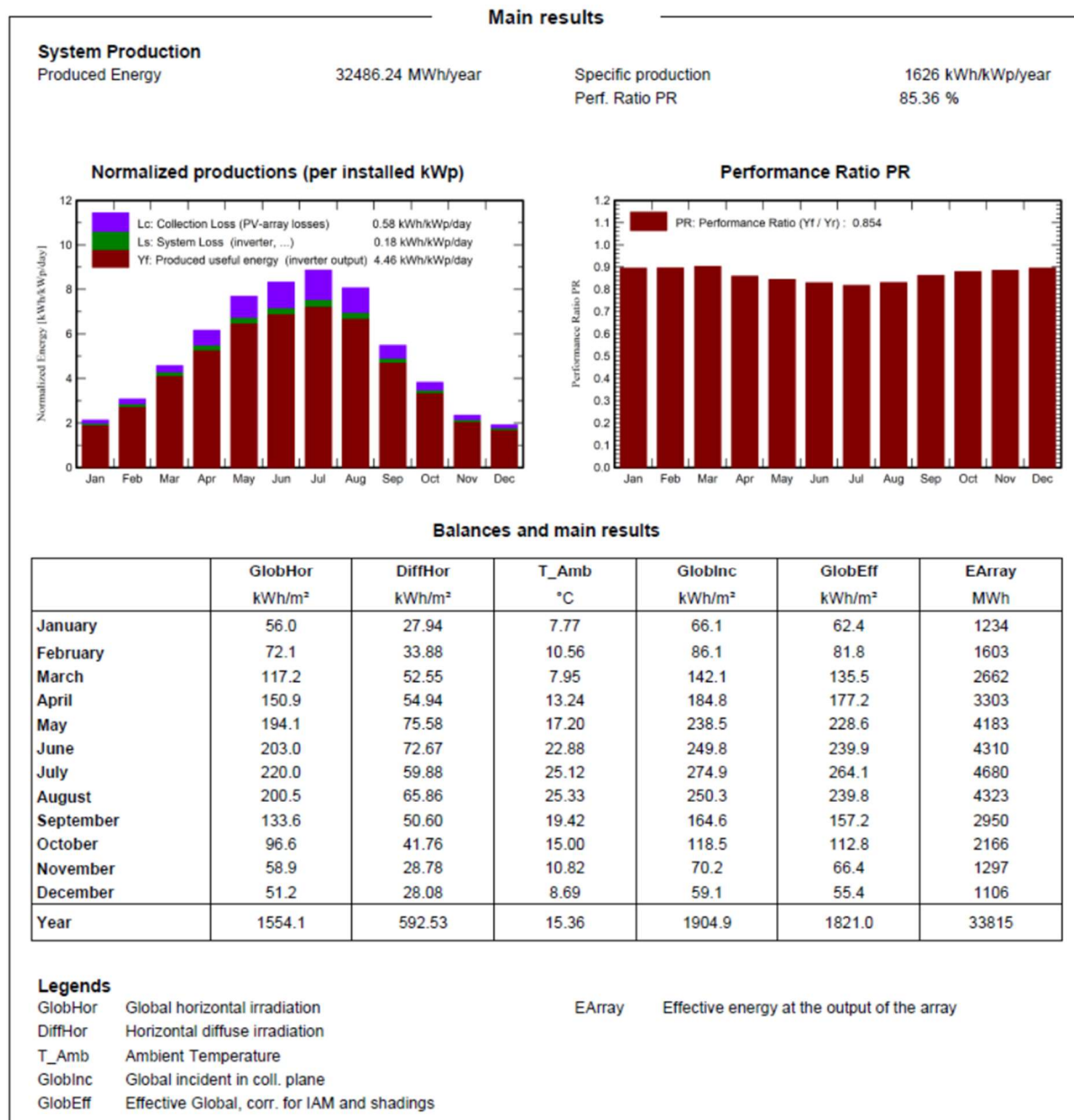
Fig. 27 - Risultati di calcolo (Fonte: PVsyst - Solcast)
