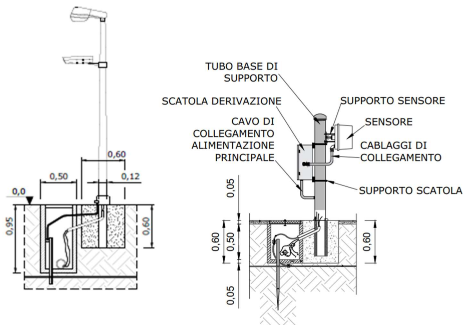
Fig. 21 – Sistema antintrusione
