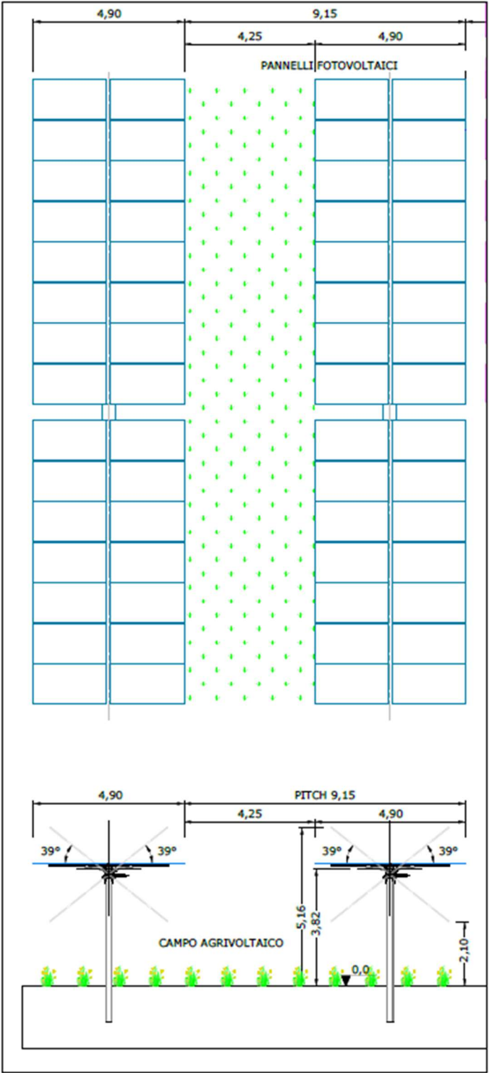
Fig. 2 – Piantumazione tra le file di tracker
