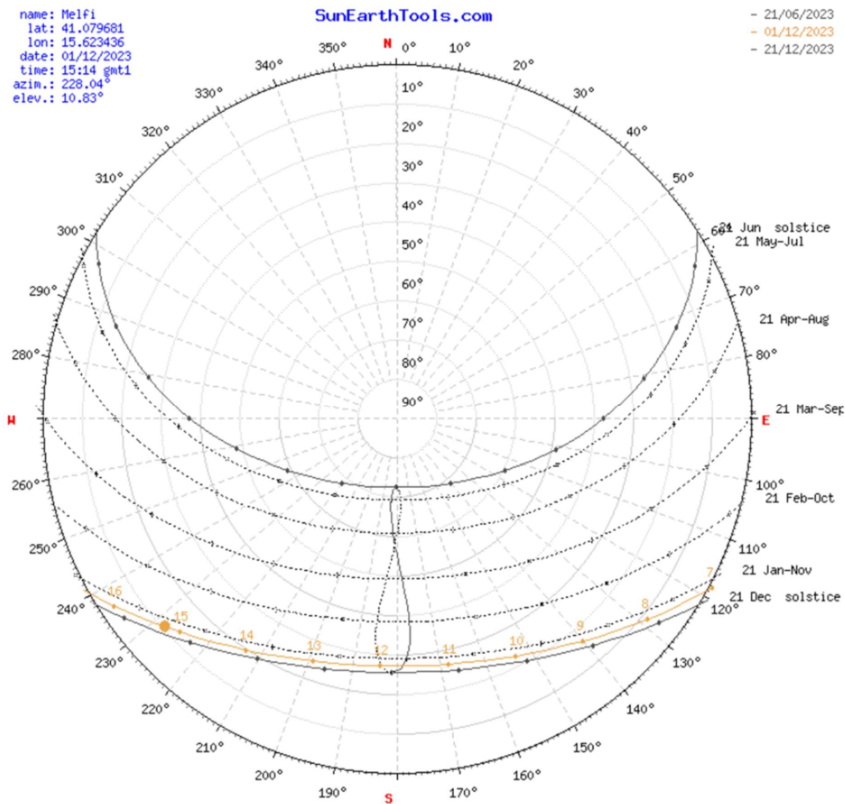
Fig. 24 - Diagramma Solare Polare (Melfi Camarda 15.9)
