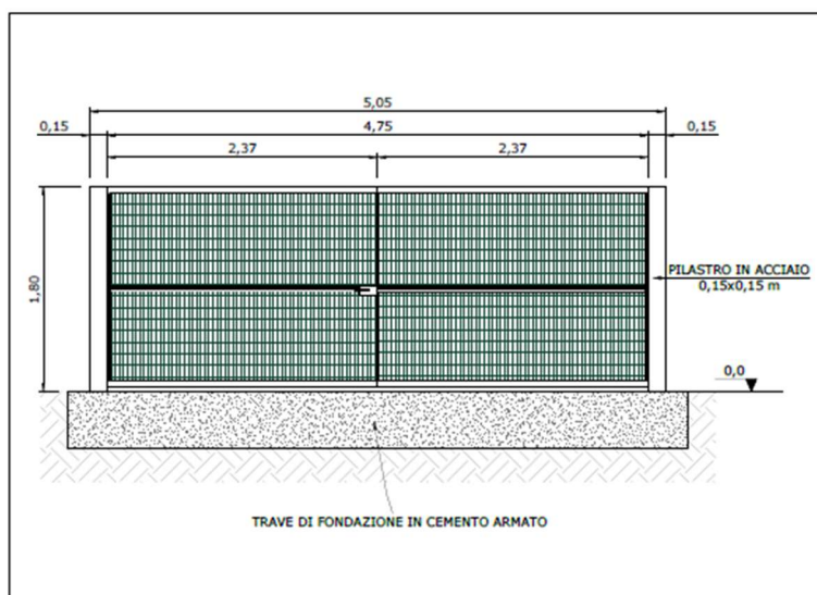
Fig. 16 – Cannello carrabile
