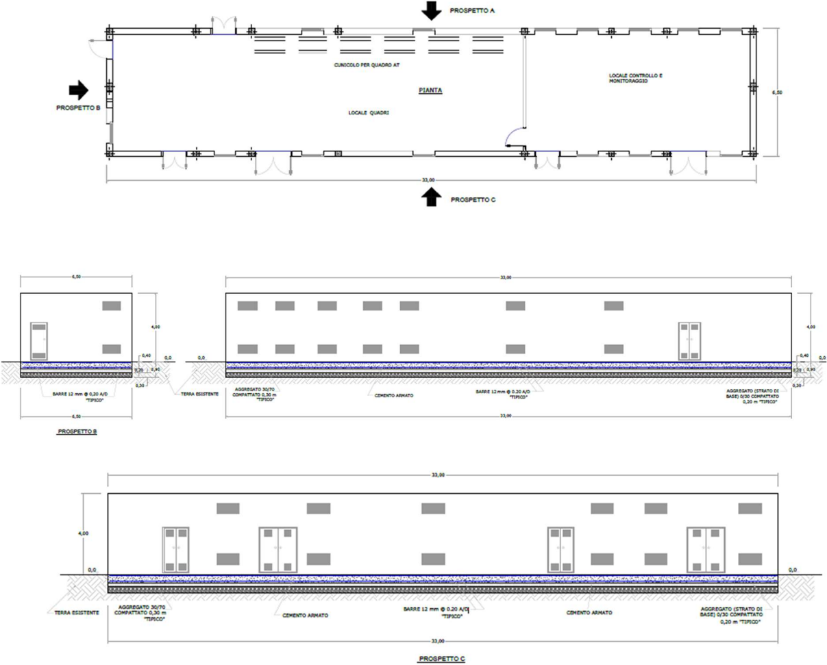
Fig. 13 - Cabina di ricezione, sezionamento e controllo
