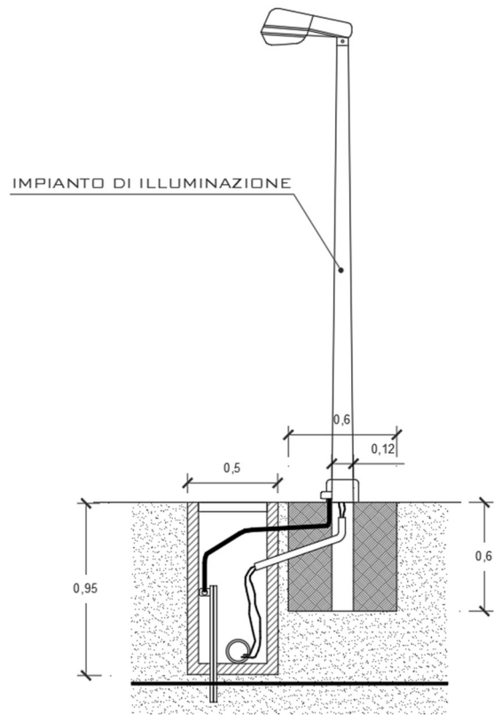
Fig. 19 – Sistema di illuminazione
