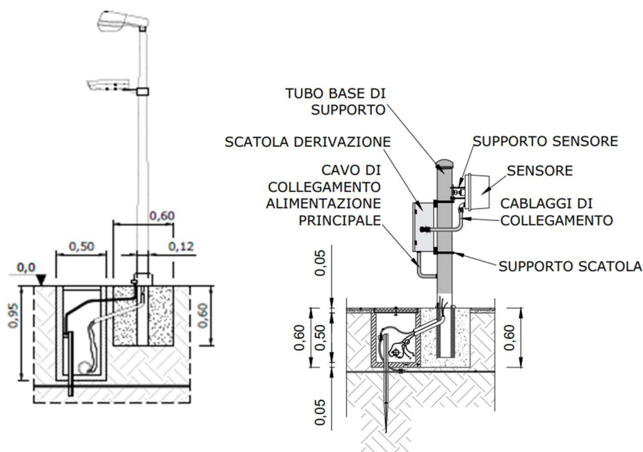
Fig. 18 – Sistema antintrusione
