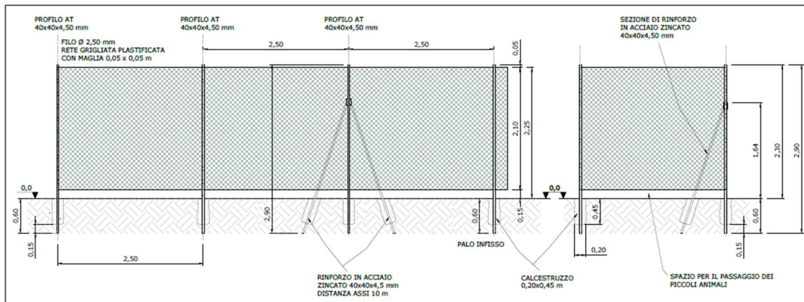
Fig. 15 – Particolare della recinzione
