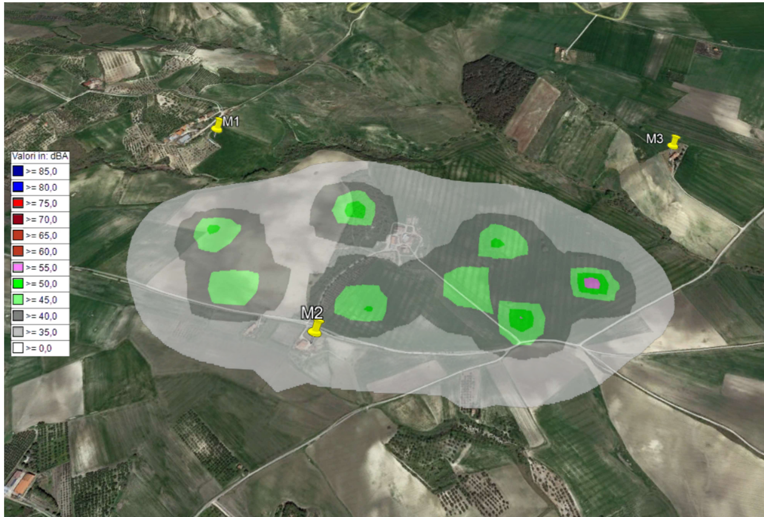
Risultato dello studio modellistico in fase di cantiere
