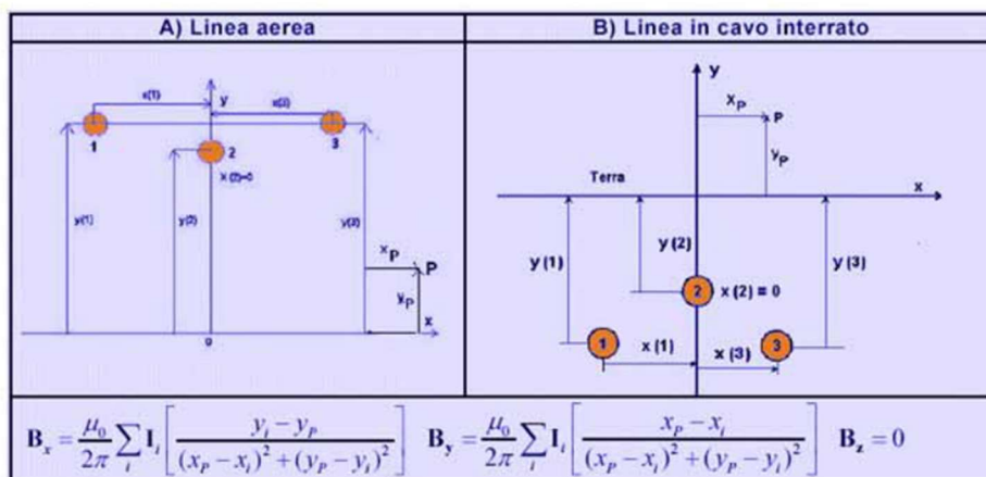
Fig.3 – Formule per la determinazione delle componenti sugli assi dell'induzione magnetica B (C.932)
