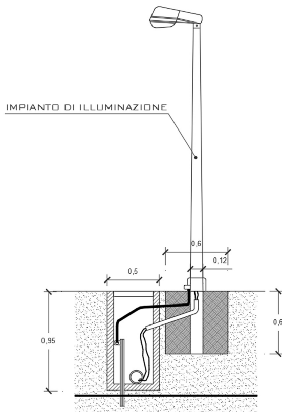
Fig. 18 – Sistema di illuminazione
