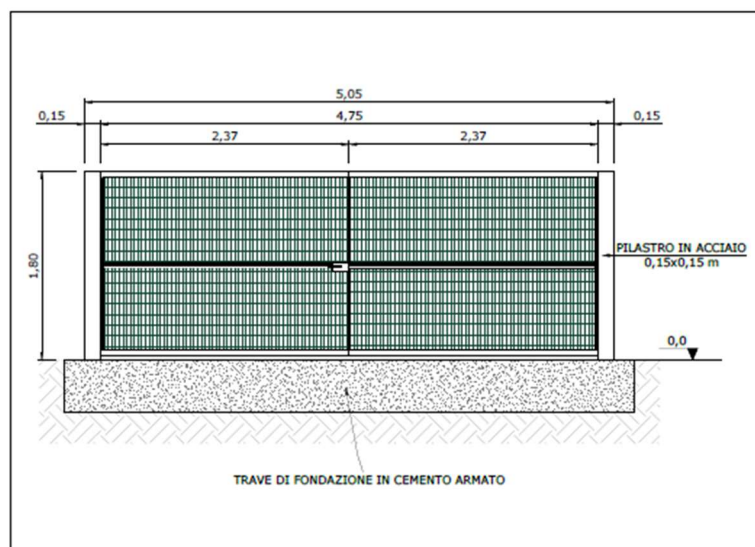
Fig. 15 – Cannello carrabile
