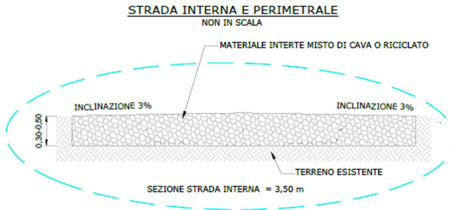
Fig. 16 – Sezione strada perimetrale
