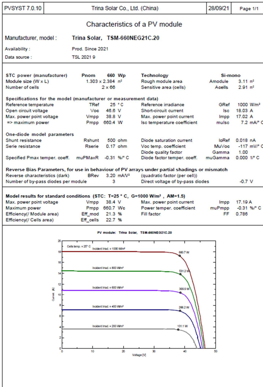
Fig. 1 - Dimensioni, specifiche tecniche e prestazionali pannelli fotovoltaici Trina Solar
