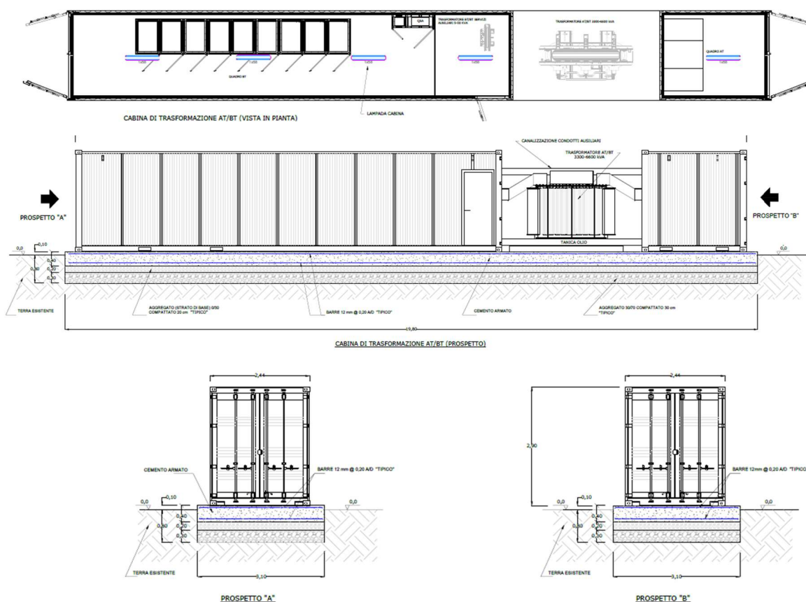
Fig. 12 - Cabina di trasformazione BT/AT
