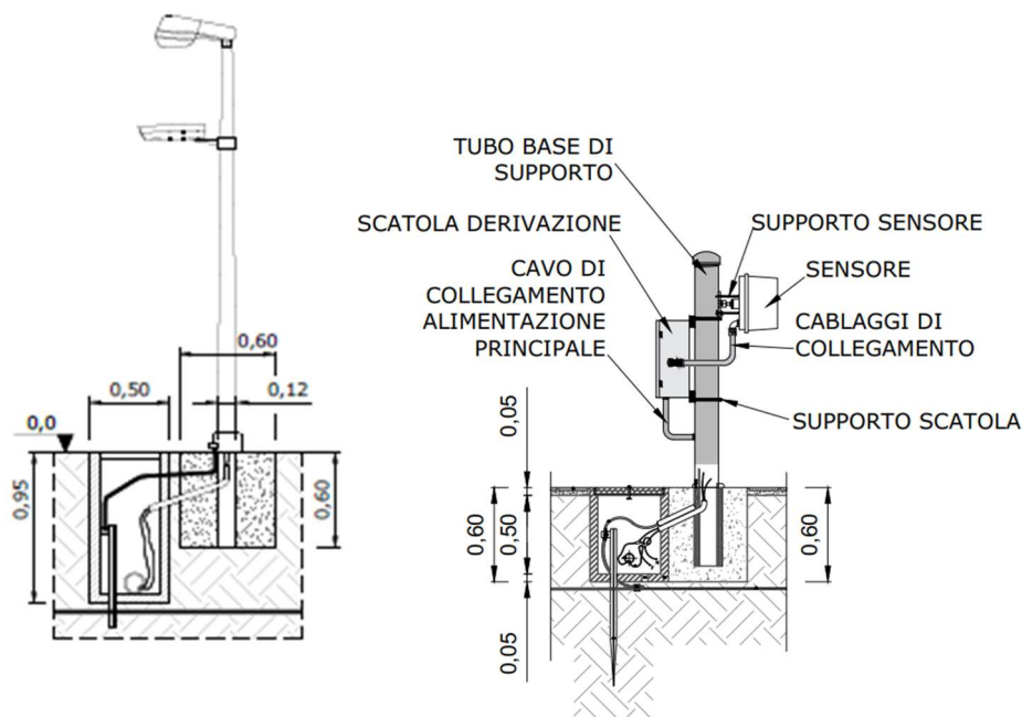
Fig. 17 – Sistema antintrusione
