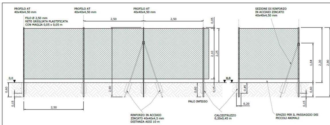
Fig. 14 – Particolare della recinzione
