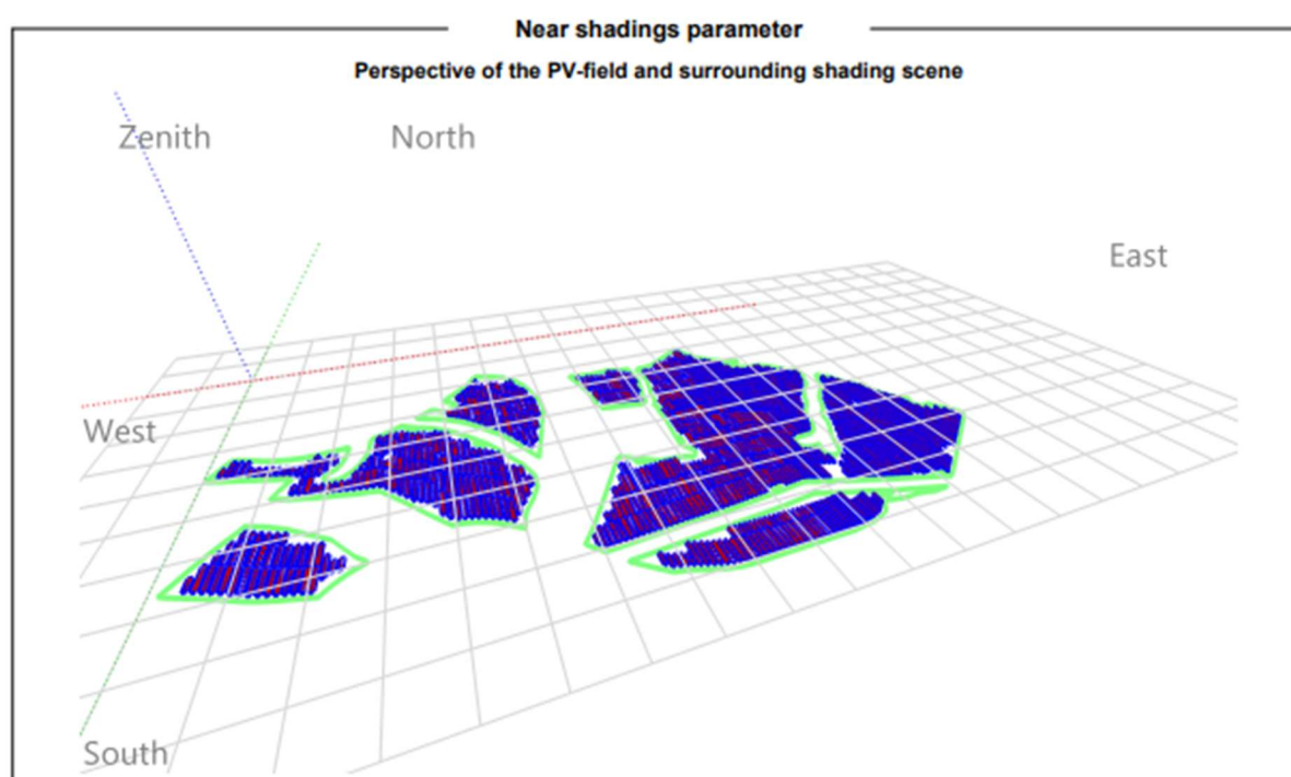
Fig. 30 – Modello 3D dell’impianto
