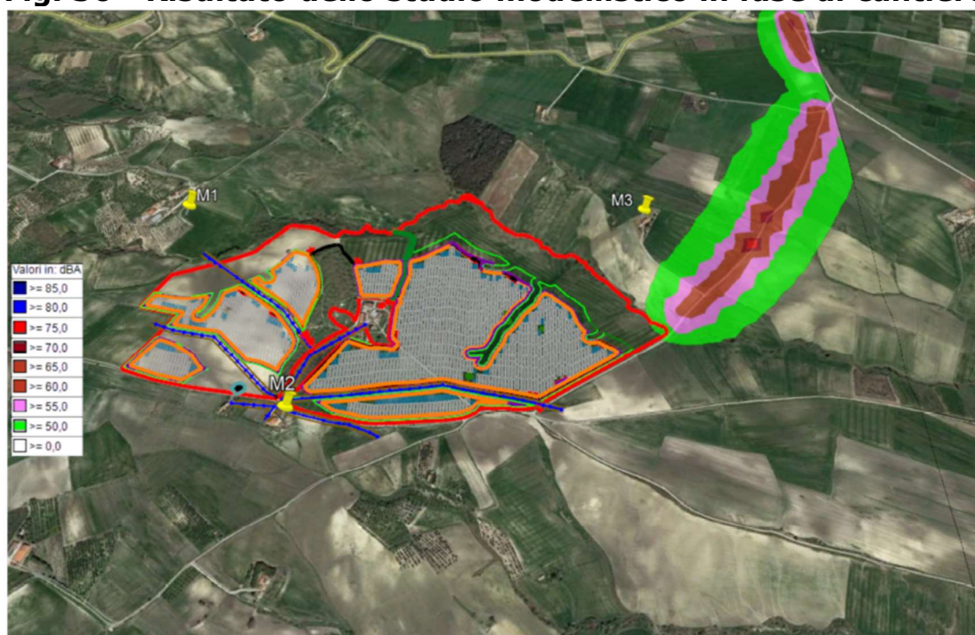
Fig. 37 - Risultato dello studio modellistico in fase di cantiere per il cavidotto
