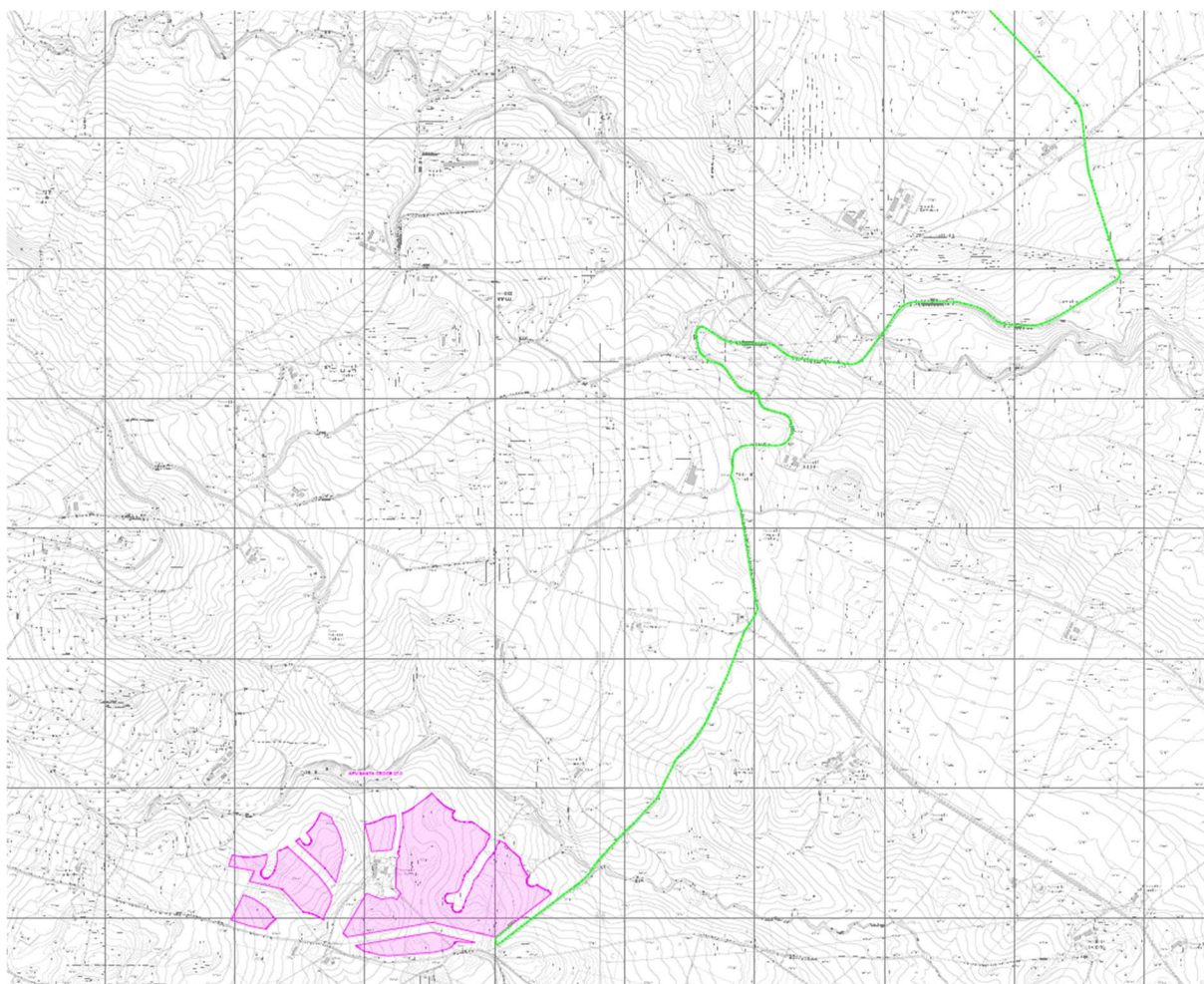
Fig. 25 – Cavidotto AT di collegamento verso la SE
