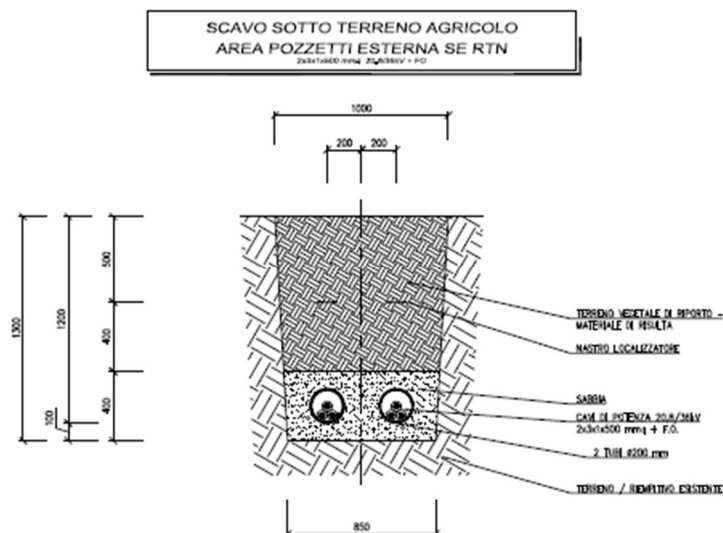
Fig. 26 – Dettagli sezioni di posa
