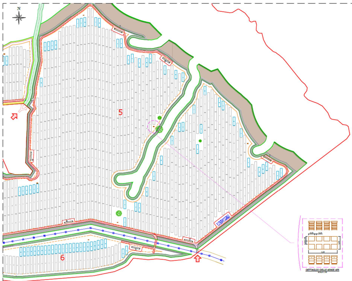
Fig. 3 – Esempio di “area di impianto” agrivoltaico
