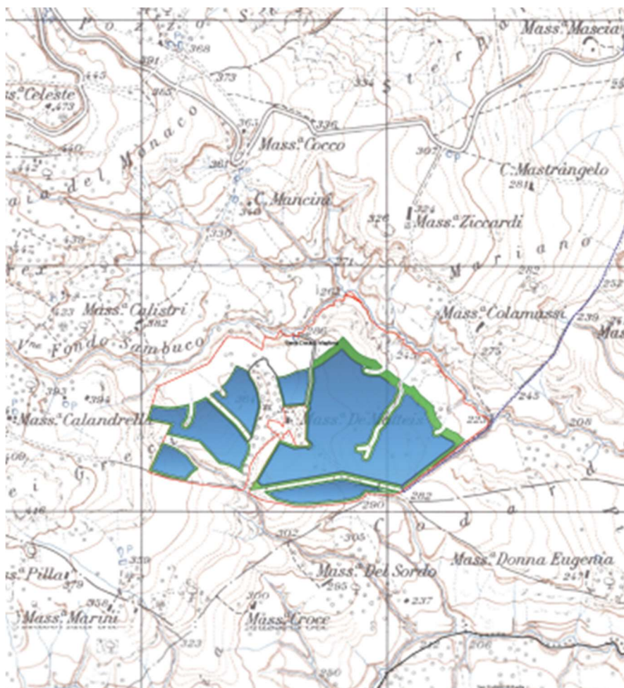
Fig.6 – Inquadramento dell’impianto su IGM
