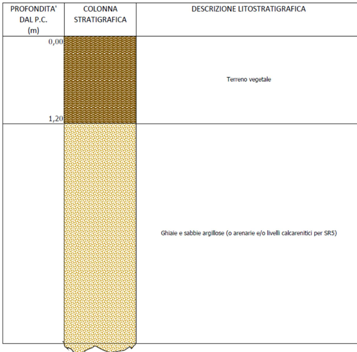
Fig. 10 – Colonna stratigrafica – profili sismici SR1, SR2, SR3, SR4, SR5, SR6
