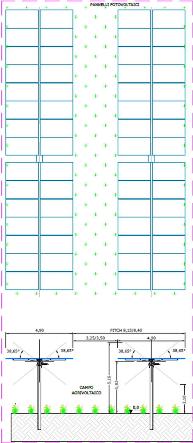
Fig. 2 – Piantumazione tra le file di tracker
