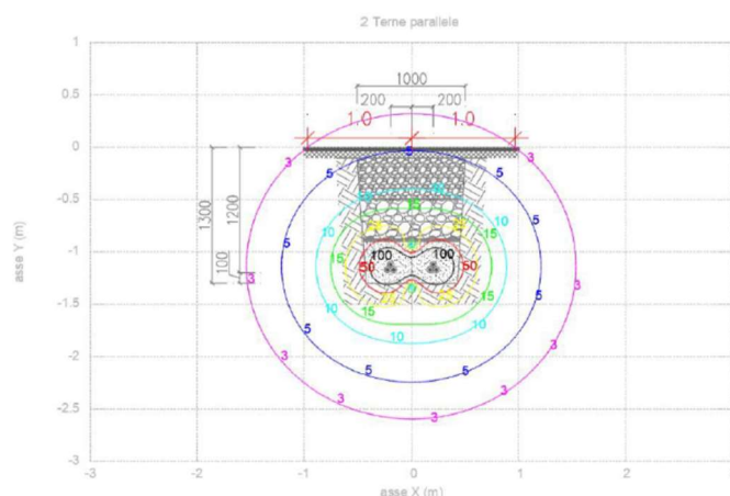
Fig. 39 – Valori di campo magnetico generati dal cavidotto
