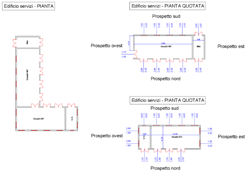
Pianta edificio in ampliamento locali tecnici
