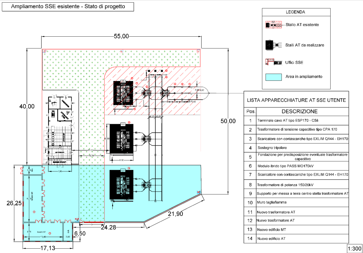
Planimetria SSE esistente – Stato di Progetto
