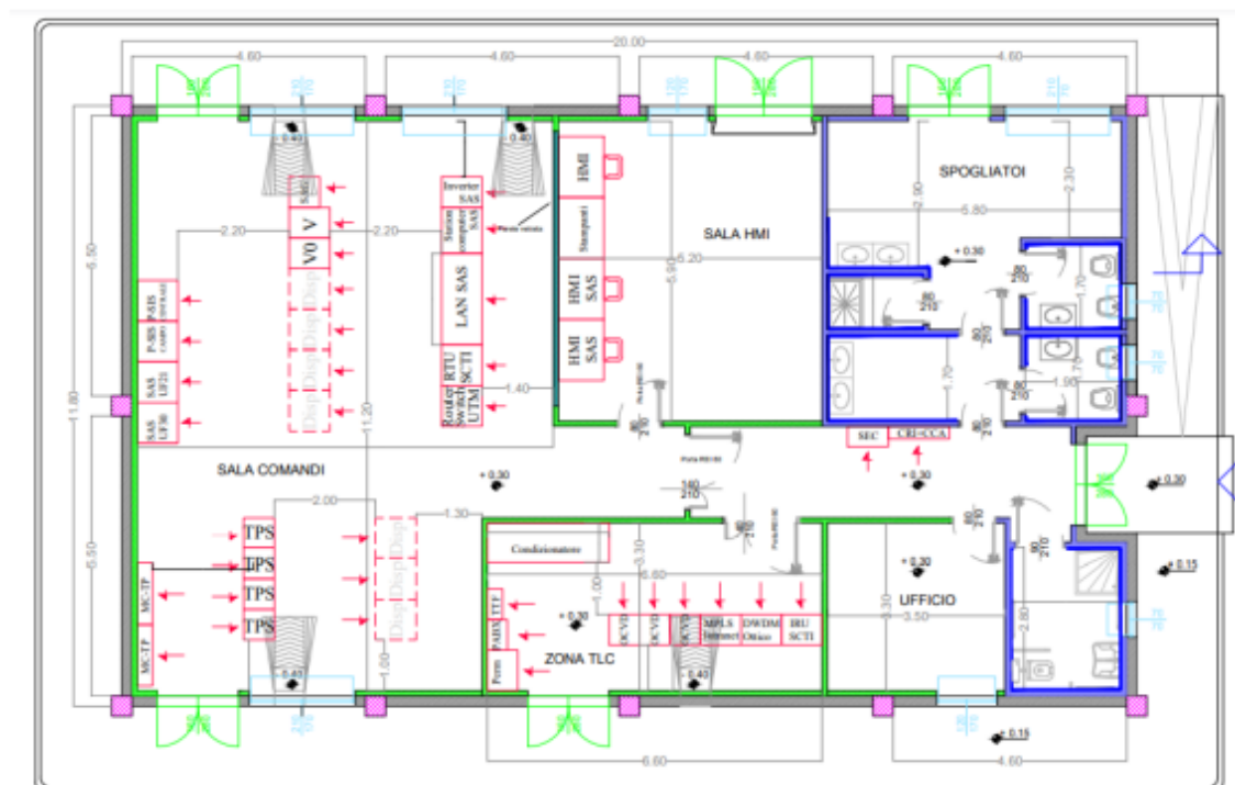
Figura 2-11: Pianta edificio comandi
