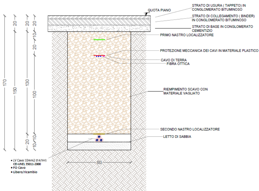
Figura 2-8: Sezione scavo su strada asfaltata
