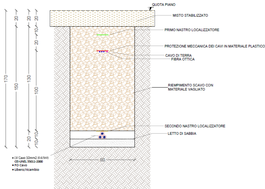
Figura 2-7: Sezione scavo su strada sterrata
