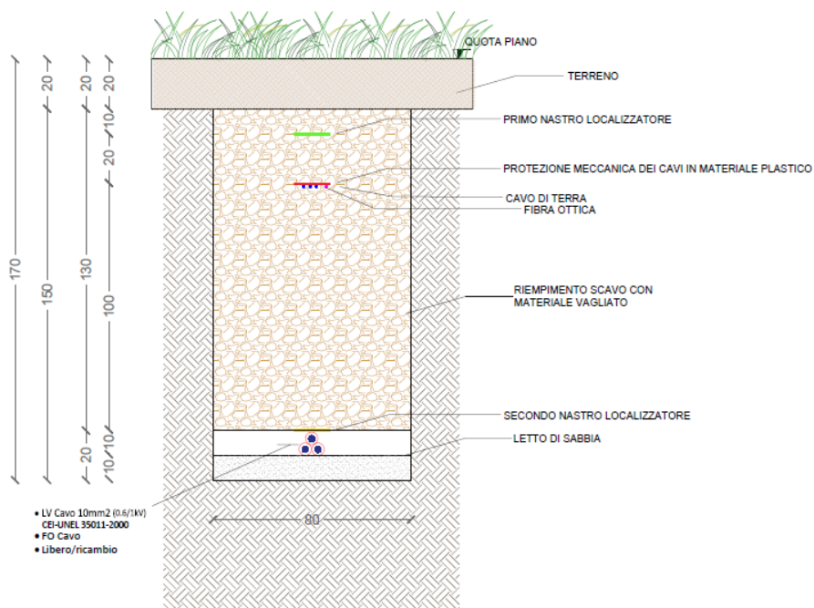
Figura 2-9: Sezione scavo su terreno agricolo
