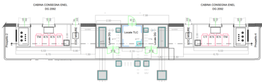
Figura 2-14: Pianta edifici consegna MT e TLC
