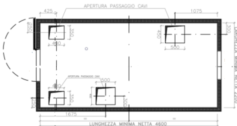
Figura 2-15: Pianta chioschi
