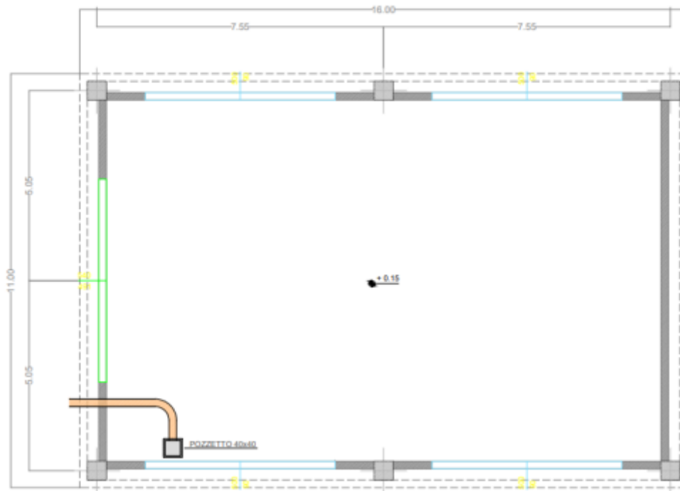
Figura 2-13: Pianta edificio magazzino
