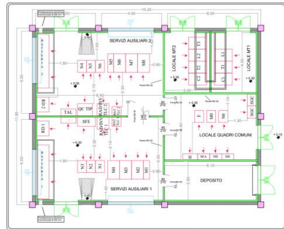
Figura 2-12: Pianta edificio servizi ausiliari
