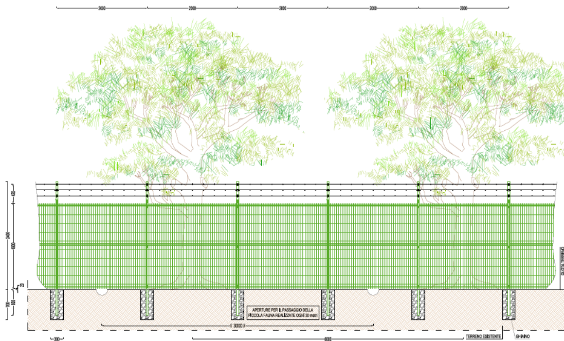
Figura 2-5: Prospetto recinzione con fascia di mitigazione
