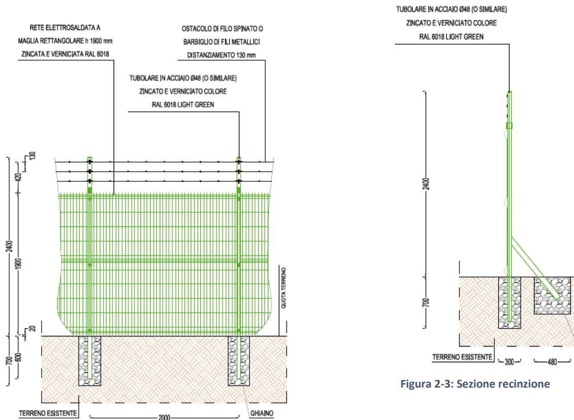
Figura 2-2: Prospetto recinzione
