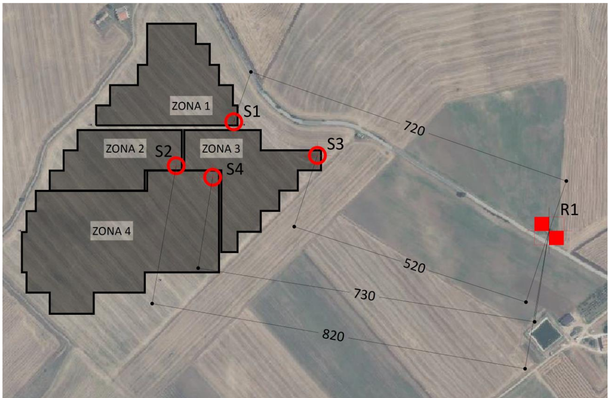
Fig. 29 – Scenario ipotizzato per verifica livello assoluto al recettore R1
