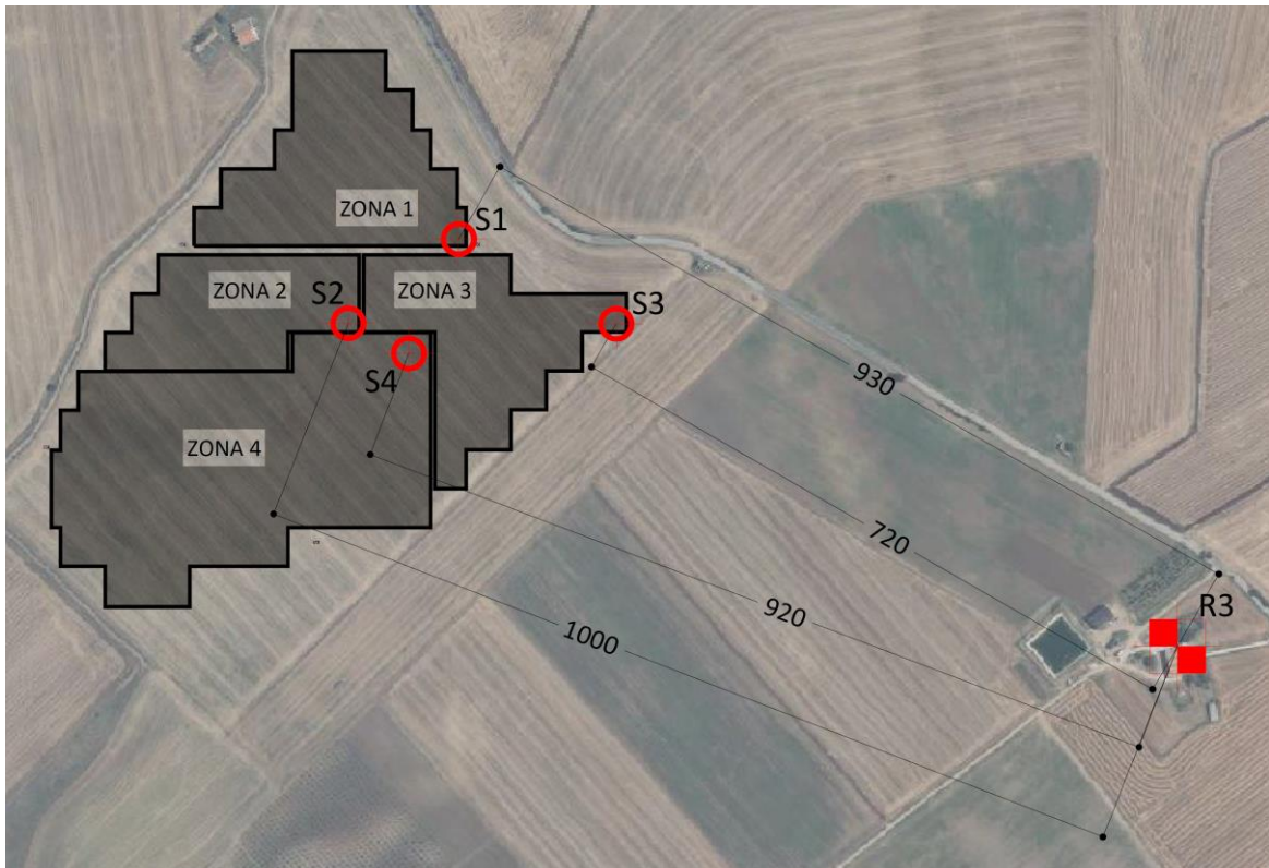
Fig. 31 – Scenario ipotizzato per verifica livello assoluto al recettore R3
