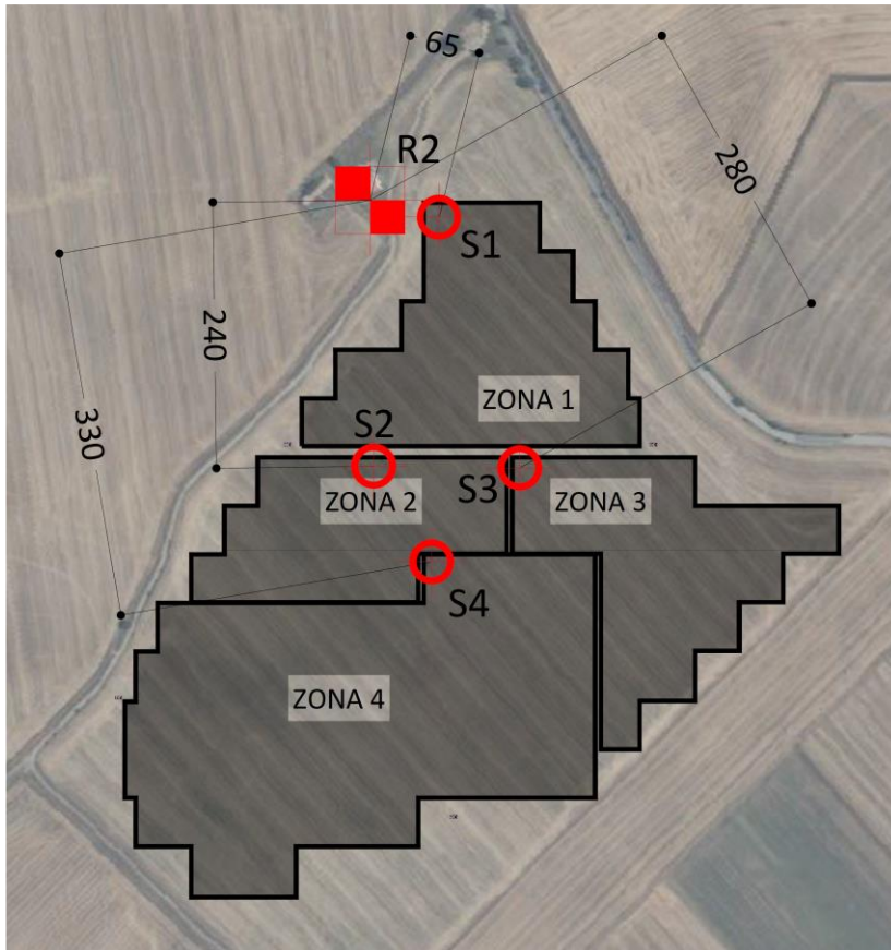
Fig. 30 – Scenario ipotizzato per verifica livello assoluto al recettore R2
