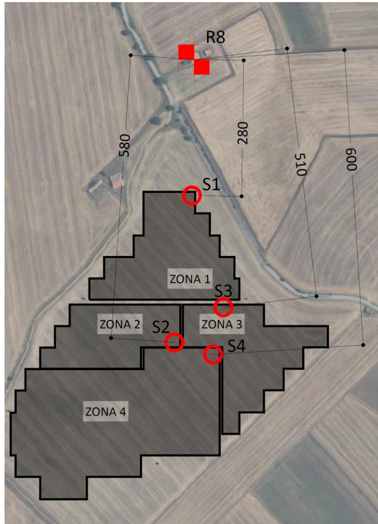
Fig. 32 – Scenario ipotizzato per verifica livello assoluto al recettore R8
