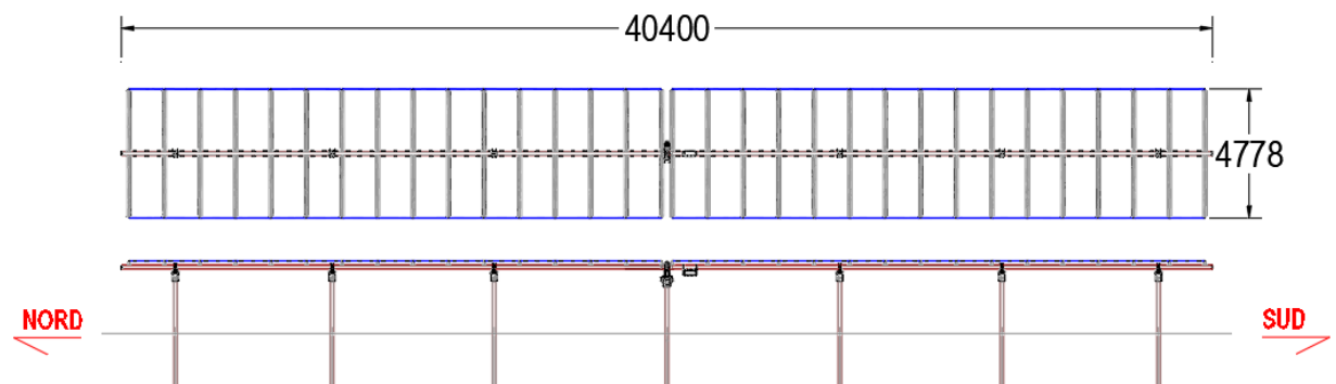
Fig. 5 – Vista laterale e vista dall'alto traker tipo
