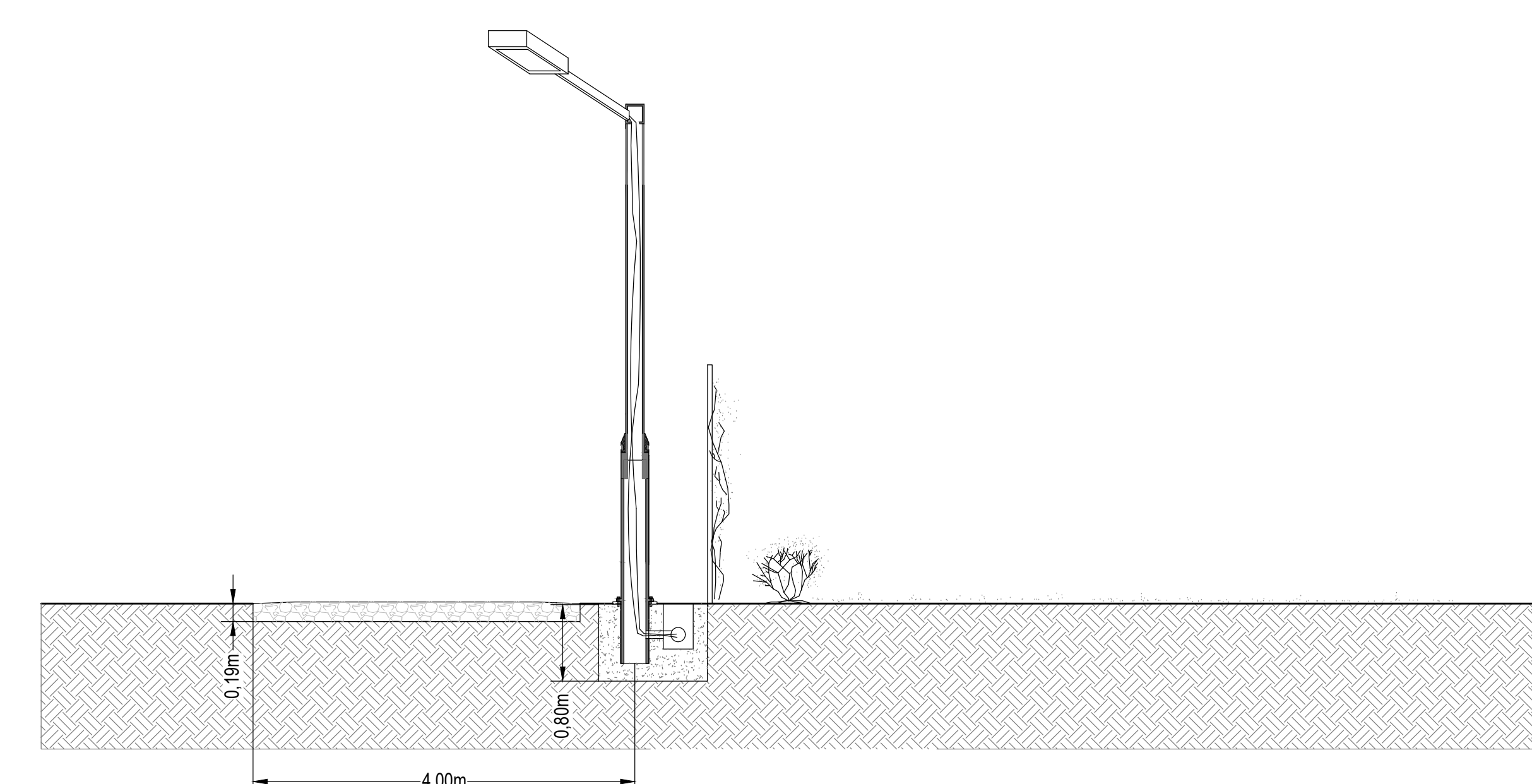
PARTICOLARE VIABILITA' E RECINZIONE LATERALE scala 1:50
