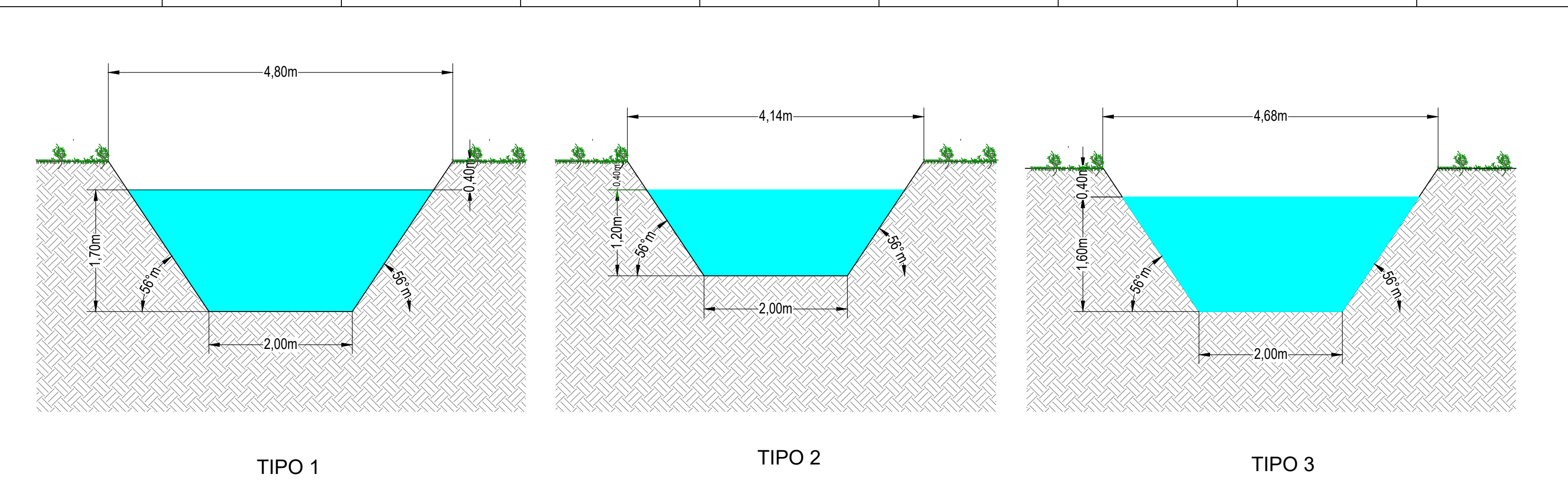
PARTICOLARE SEZIONI TRASVERSALI FOSSI DI SCOLO scala 1:50
