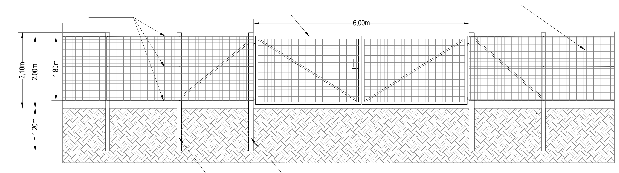
PARTICOLARE RECINZIONE E CANCELLO DI ACCESSO scala 1:50
