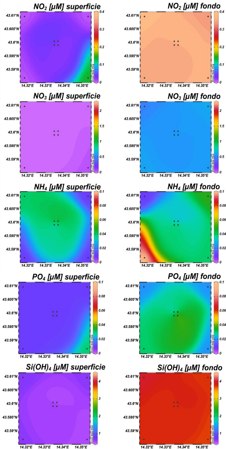
Fig. 3.21 - Mappe areali in superficie e al fondo rappresentanti le concentrazioni di fosfati (PO 4 ), silicati (Si(OH) 4 ), nitrati (NO 3 ), nitriti (NO 2 ) e ammonio (NH 4 ) espresse in μM. Luglio 2022 . Grafico realizzato mediante il software Ocean Data View – ODV (© 2016 Reiner Schlitzer).
