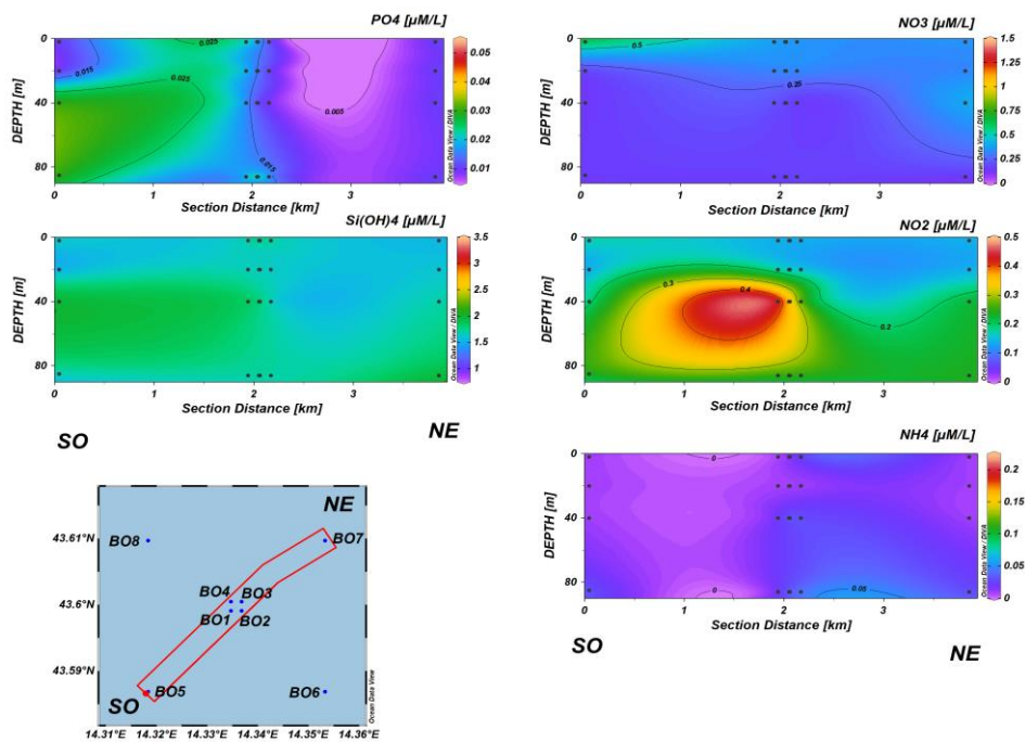
Fig. 3.16b - Sezioni SO-NE delle stazioni BO5, BO1, BO2, BO4, BO3 e BO7 rappresentanti le concentrazioni di fosfati ( PO_4 ), silicati ( Si(OH)_4 ), nitrati ( NO_3 ), nitriti ( NO_2 ) e ammonio ( NH_4 ) espresse in \mu M . Marzo 2022.
