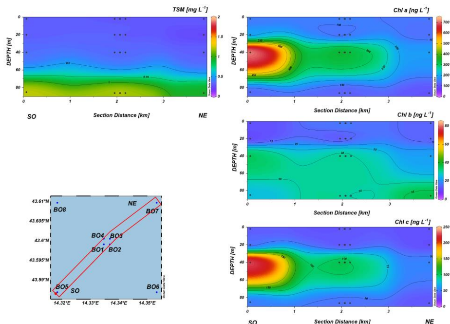
Fig. 3.32b - Sezioni SO-NE delle stazioni BO5, BO1, BO2, BO4, BO3 e BO7 rappresentanti le concentrazioni di particolato sospeso (TSM) espresso in \text{mg L}^{-1} , clorofilla a (Chl a), clorofilla b (Chl b), clorofilla c (Chl c), espresse in \text{ng L}^{-1} . Novembre 2022 . Grafico realizzato mediante il software Ocean Data View – ODV (© 2016 Reiner Schlitzer).
