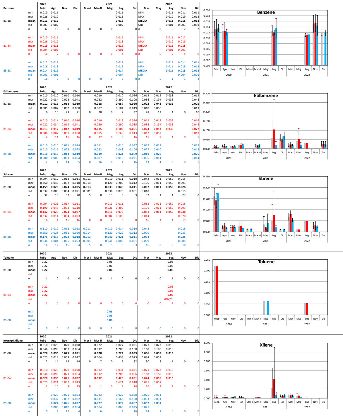
Fig. 3.39 - Andamento dei BTEX relativo al 2022 e confronto con gli anni 2020 e 2021. Nelle tabelle dei singoli composti sono riportati i valori minimo, massimo, media, deviazione standard ed il numero di campioni in cui i BTEX sono risultati rilevabili nell'intero areale (BO1 - BO8, in nero, in grigio nel grafico) nelle stazioni poste a 100 m dalla piattaforma Bonaccia NW (BO1 - BO4, in rosso nelle tabelle e nei grafici) e nelle stazioni di controllo poste a 2000 m dalla piattaforma (BO5 - BO8 in azzurro nelle tabelle e nei grafici). Tutte le misure sono espresse in \mu\text{g L}^{-1} .
