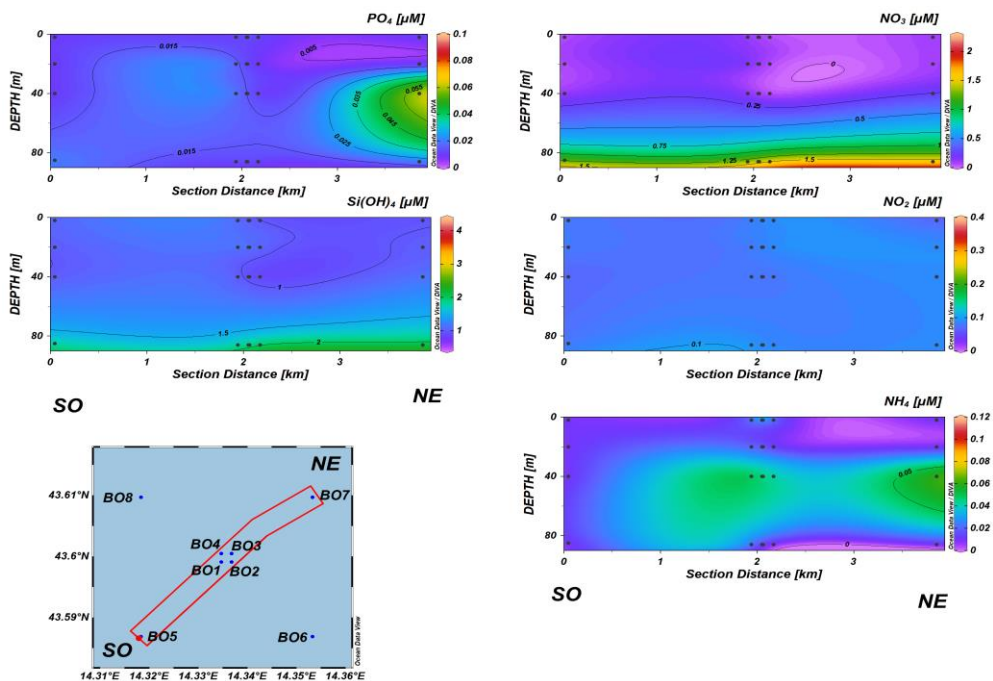
Fig. 3.24b - Sezioni SO-NE delle stazioni BO5, BO1, BO2, BO4, BO3 e BO7 rappresentanti le concentrazioni di fosfati ( PO_4 ), silicati ( Si(OH)_4 ), nitrati ( NO_3 ), nitriti ( NO_2 ) e ammonio ( NH_4 ) espresse in \mu M . Dicembre 2022 . Grafico realizzato mediante il software Ocean Data View – ODV (© 2016 Reiner Schlitzer).
