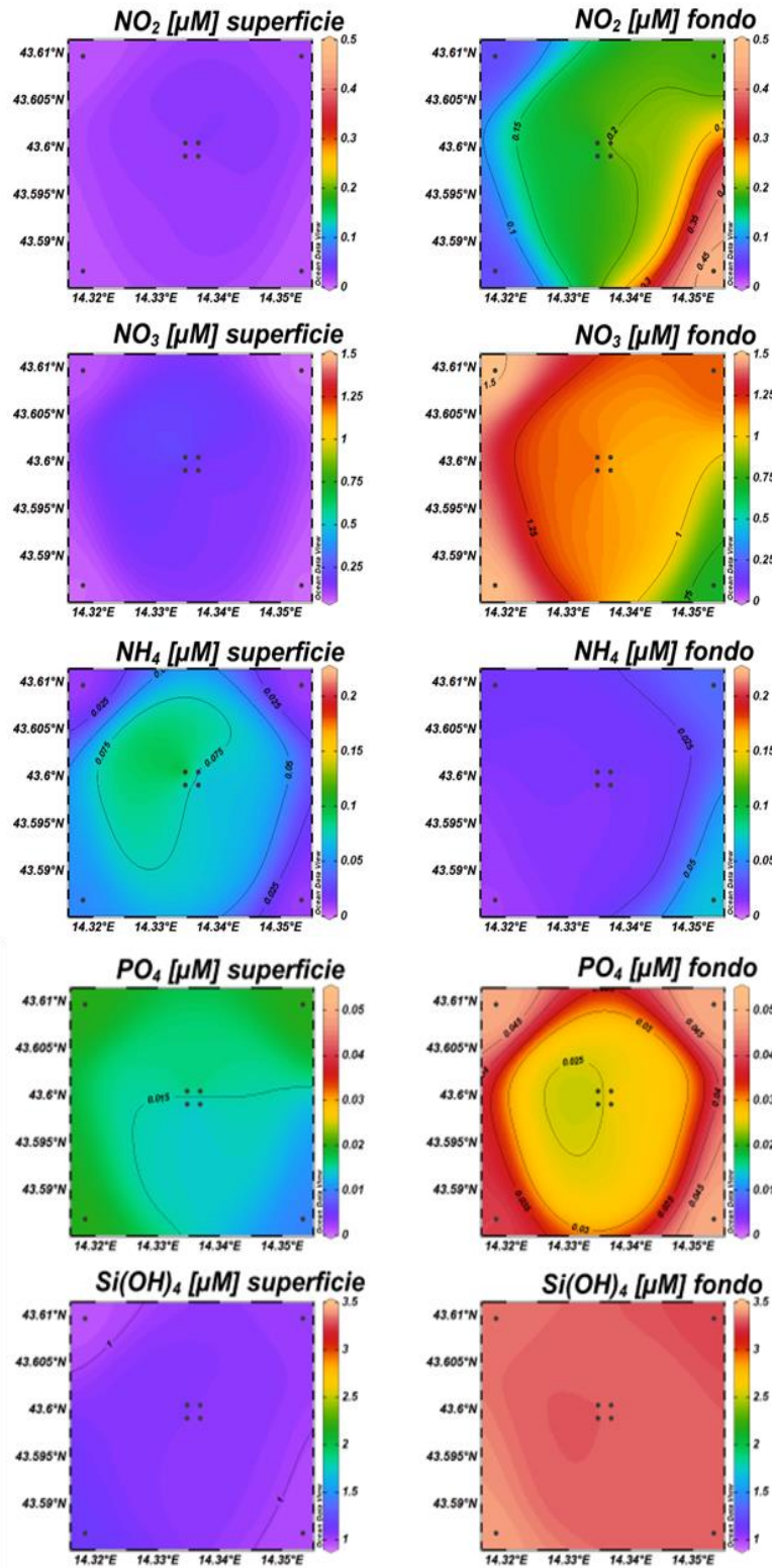
Fig. 3.19 - Mappe areali in superficie e al fondo rappresentanti le concentrazioni di fosfati (PO 4 ), silicati (Si(OH) 4 ), nitrati (NO 3 ), nitriti (NO 2 ) e ammonio (NH 4 ) espresse in μM. Maggio 2022.
