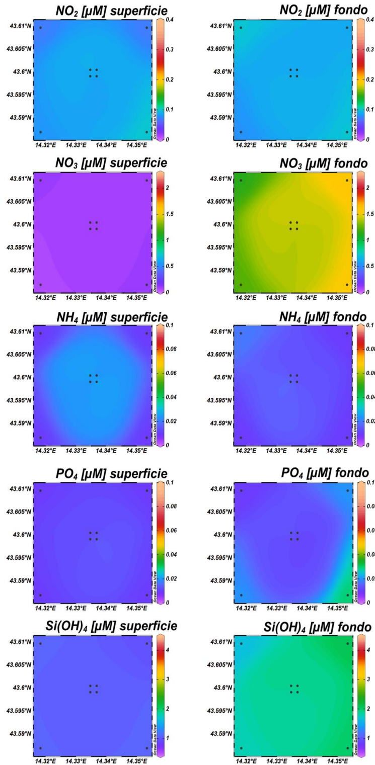
Fig. 3.25 - Mappe areali in superficie e al fondo rappresentanti le concentrazioni di fosfati (PO 4 ), silicati (Si(OH) 4 ), nitrati (NO 3 ), nitriti (NO 2 ) e ammonio (NH 4 ) espresse in \mu M. Dicembre 2022. Grafico realizzato mediante il software Ocean Data View – ODV (© 2016 Reiner Schlitzer).
