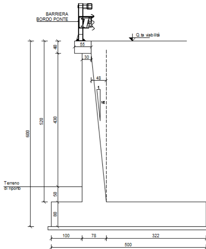
Figura 2.1 – Muro Tipo D1
