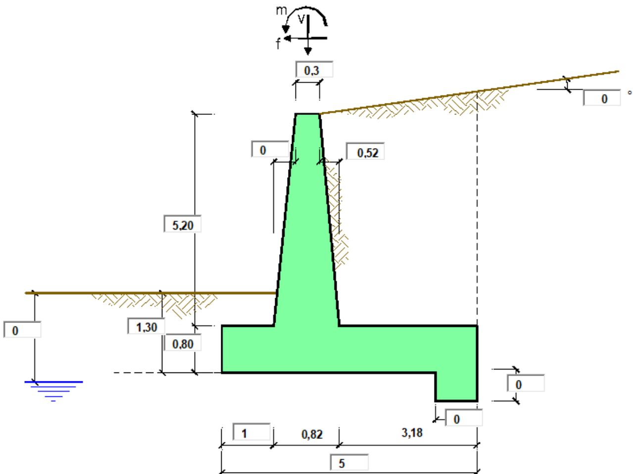
Figura 8.1 - Muro Tipo D1
