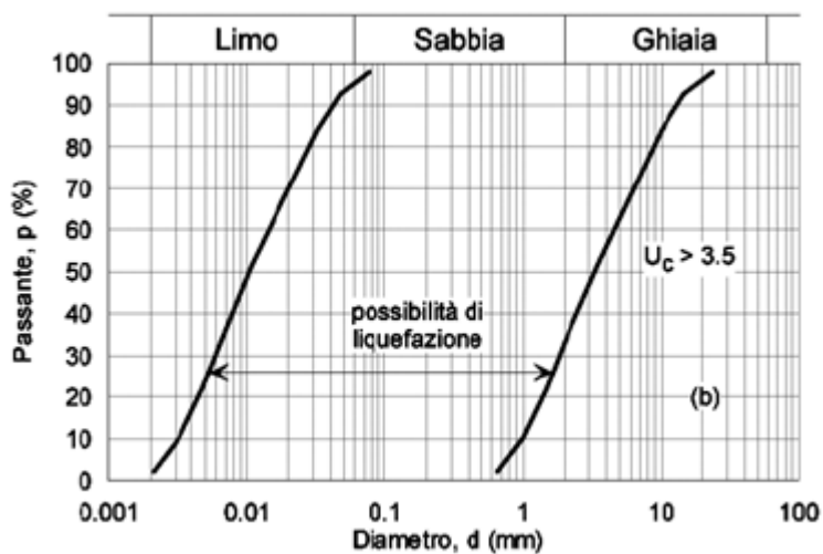
Figure 9-49 – Fusi granulometrici di terreni suscettibili alla liquefazione per U_c > 3.5
