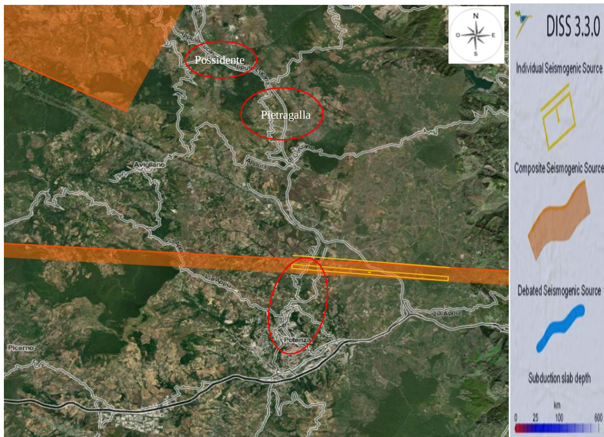
Figure 8-9 – Sorgenti sismogenetiche contenute nella nuova versione del “Database of Individual Seismogenic Sources” per l’area di Possidente, Pietragalla e Potenza (indicata in rosso)
