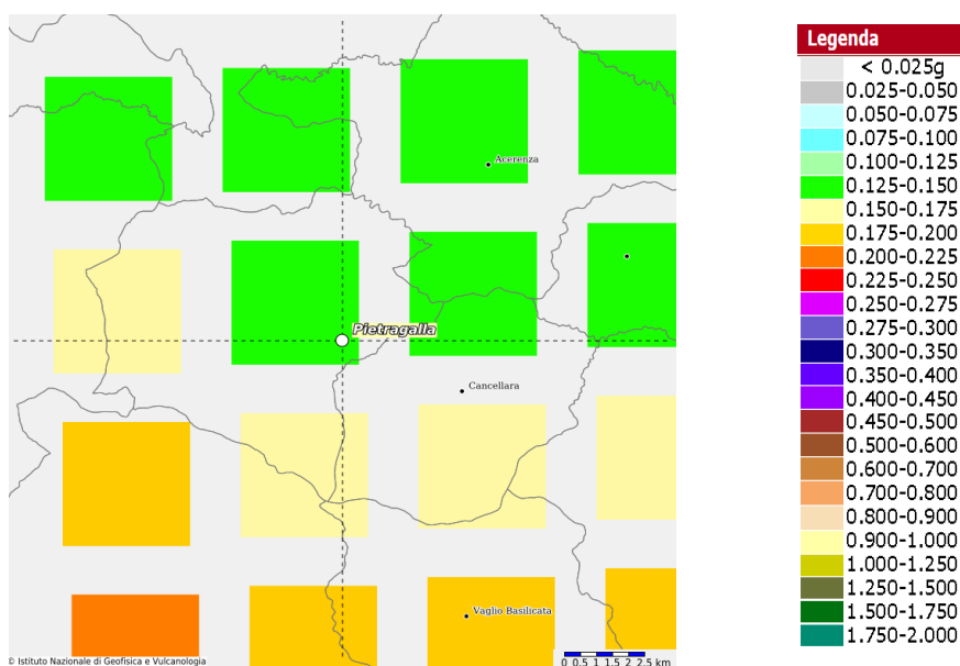
Figure 8-3– Mappa di pericolosità sismica espressa in termini di accelerazione massima del suolo ( a_{max} ) con probabilità di eccedenza del 10% in 50 anni riferita a suoli molto rigidi ( V_{s30} > 800 m/s) – da INGV
