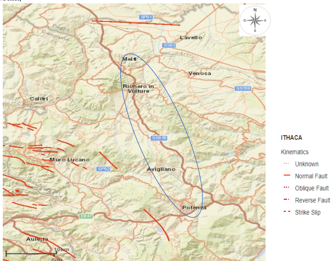
Figure 8-12 – Stralcio cartografico dell'area di Melfi a Potenza e faglie capaci (ITHACA, 2019)
