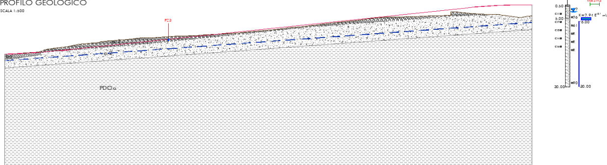
PROFILO GEOLOGICO SCALA 1:500
