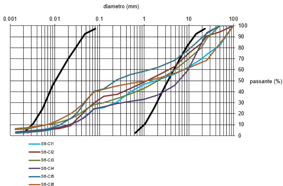
Figure 9-29 – Fusi granulometrici relativo al sondaggio S6
