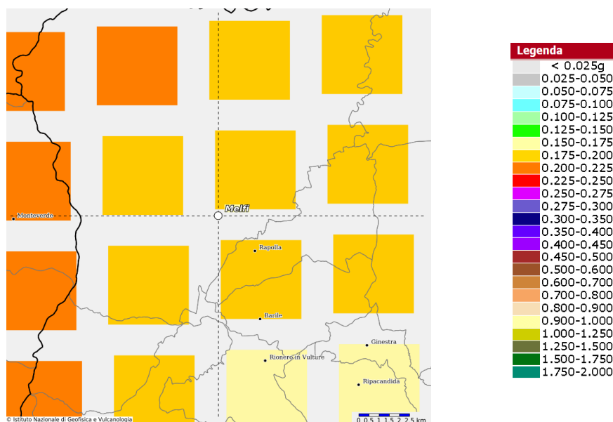
Figure 8-2 – Mappa di pericolosità sismica espressa in termini di accelerazione massima del suolo ( a_{max} ) con probabilità di eccedenza del 10% in 50 anni riferita a suoli molto rigidi ( V_{s30} > 800 m/s) – da INGV
