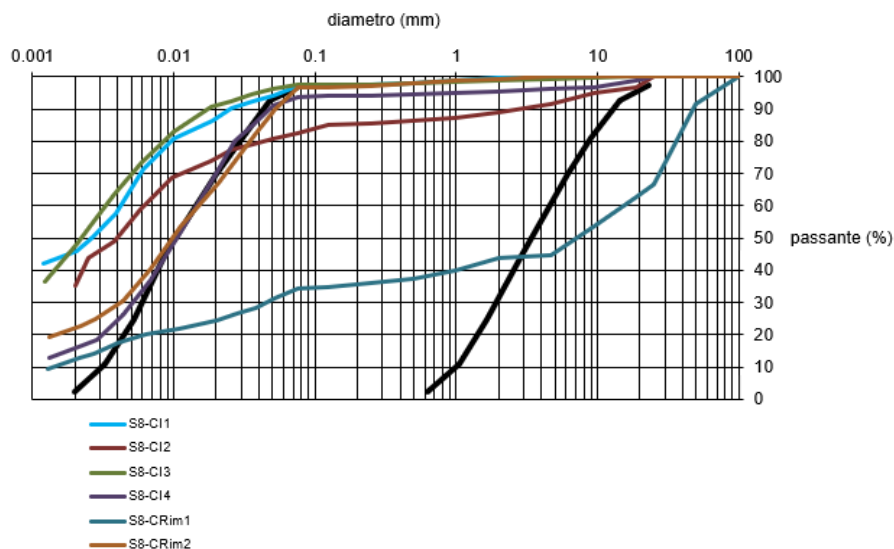
Figure 9-36 – Fusi granulometrici relativi al sondaggio S8
