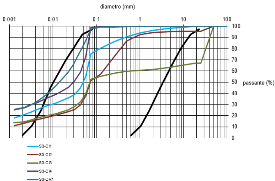
Figure 9-12 – fuso granulometrici relativo al sondaggio S3
