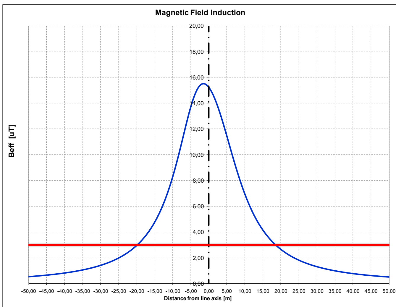
Fig. 1: andamento dell'induzione magnetica in una sezione perpendicolare all'asse linea, calcolata a 1,5 m dal suolo in caso di franco minimo (obiettivo di qualità pari a 3 \mu\text{T} )
