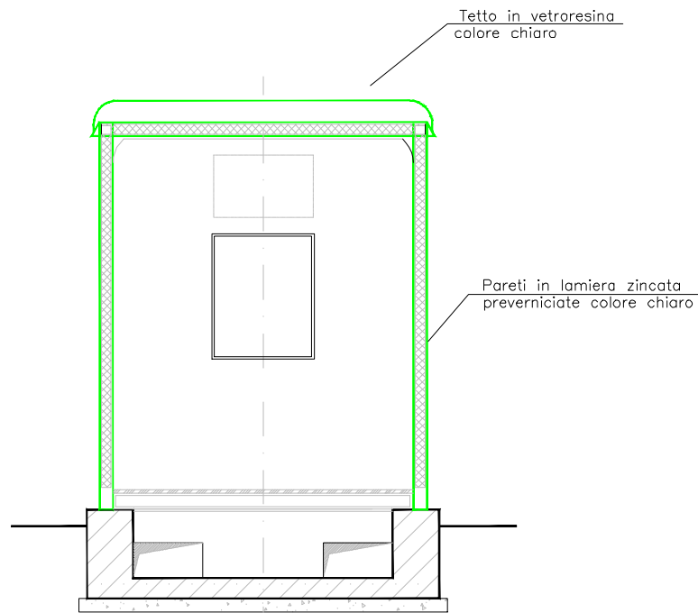
SEZIONE W-W
