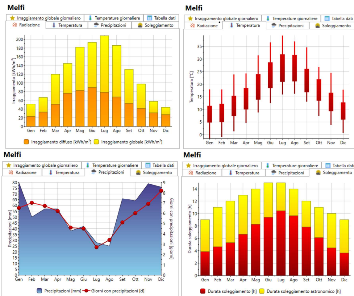
Fig. 26 – Dati di radiazione, temperatura, precipitazioni e soleggiamento (Riferiti al sito di Melfi)
