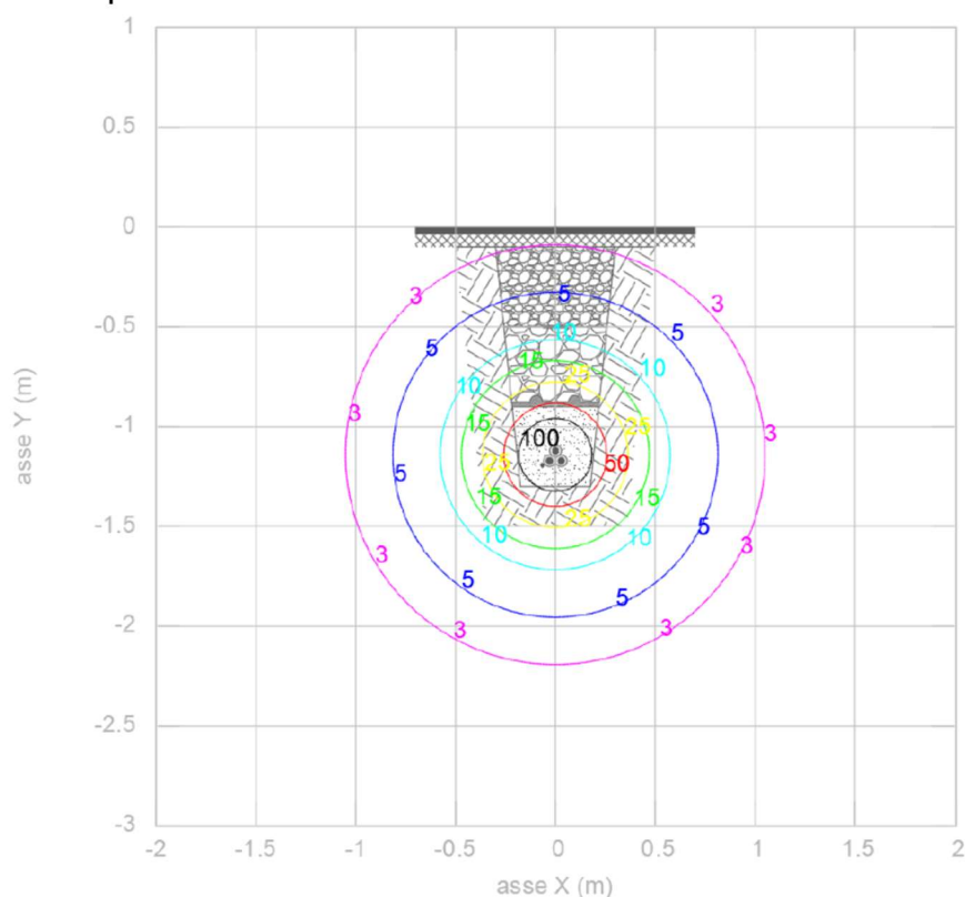
Fig. 39 – Valori di campo magnetico generati dal cavidotto
