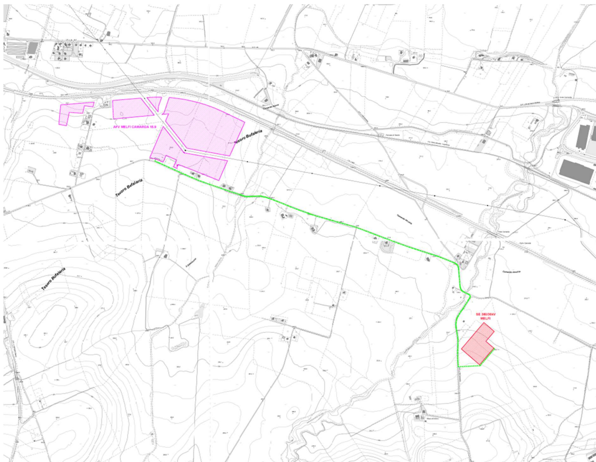
Fig. 24 – Cavidotto AT di collegamento verso la SE
