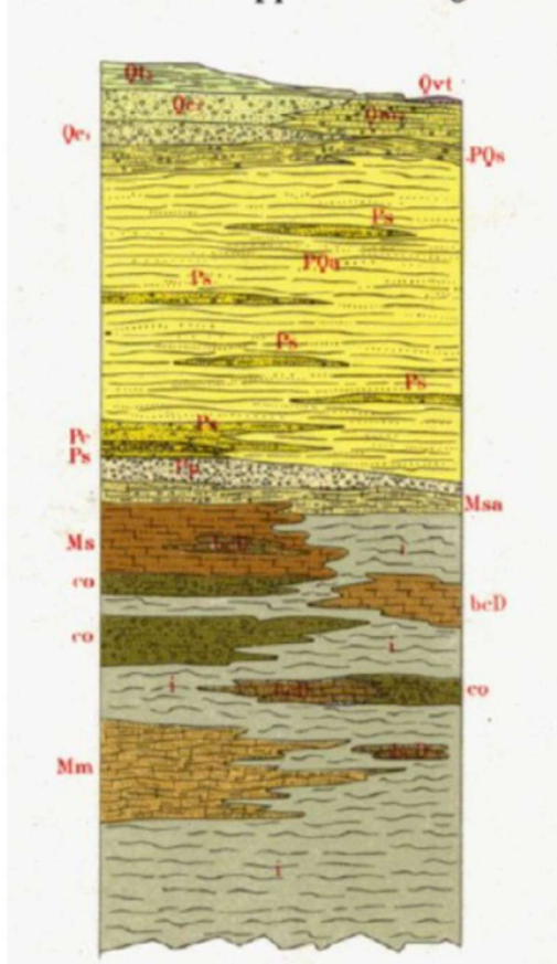
Fig. 9 – Carta geologica
