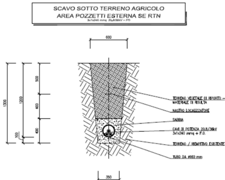
Fig. 25 – Dettagli sezioni di posa
