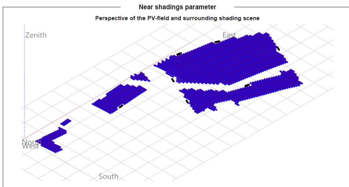
Fig. 29 – Modello 3D dell’impianto
