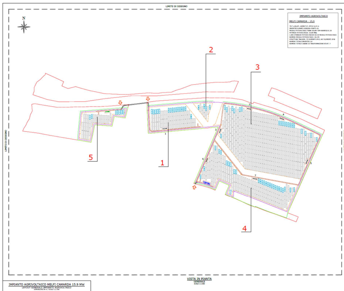
Fig. 23 - Layout di impianto
