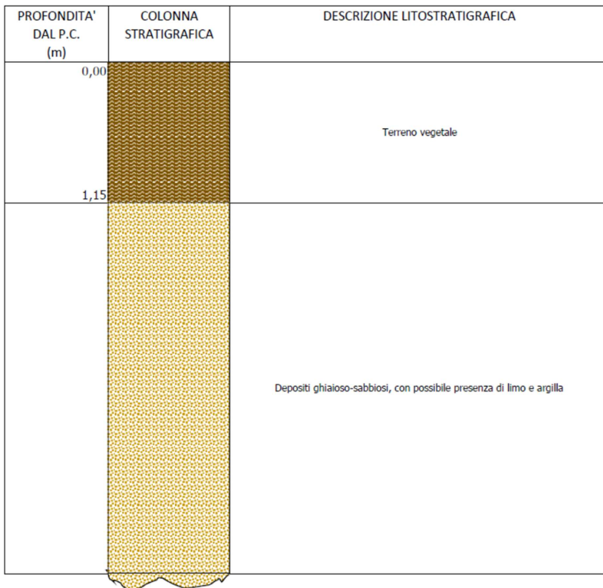
Fig. 10 – Colonna stratigrafica
