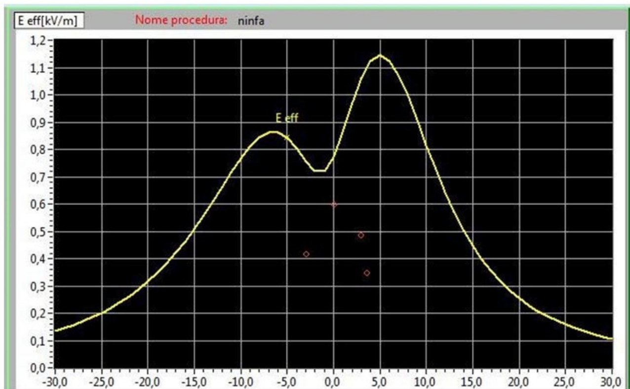
Figura 12 - Grafico dell'intensità del campo elettrico al suolo
