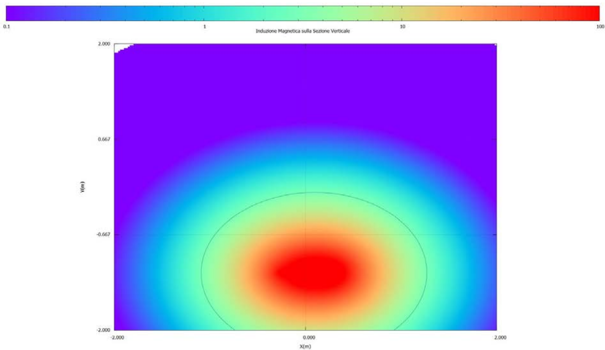
Figura 8 - Mappa a colori induzione magnetica con isolinea 3\mu T
