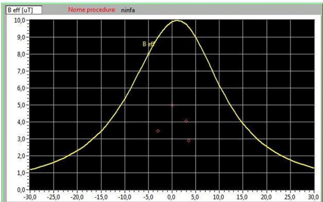
Figura 13 - Profili laterali del campo magnetico sulla sezione trasversale dell'asse della linea aerea
