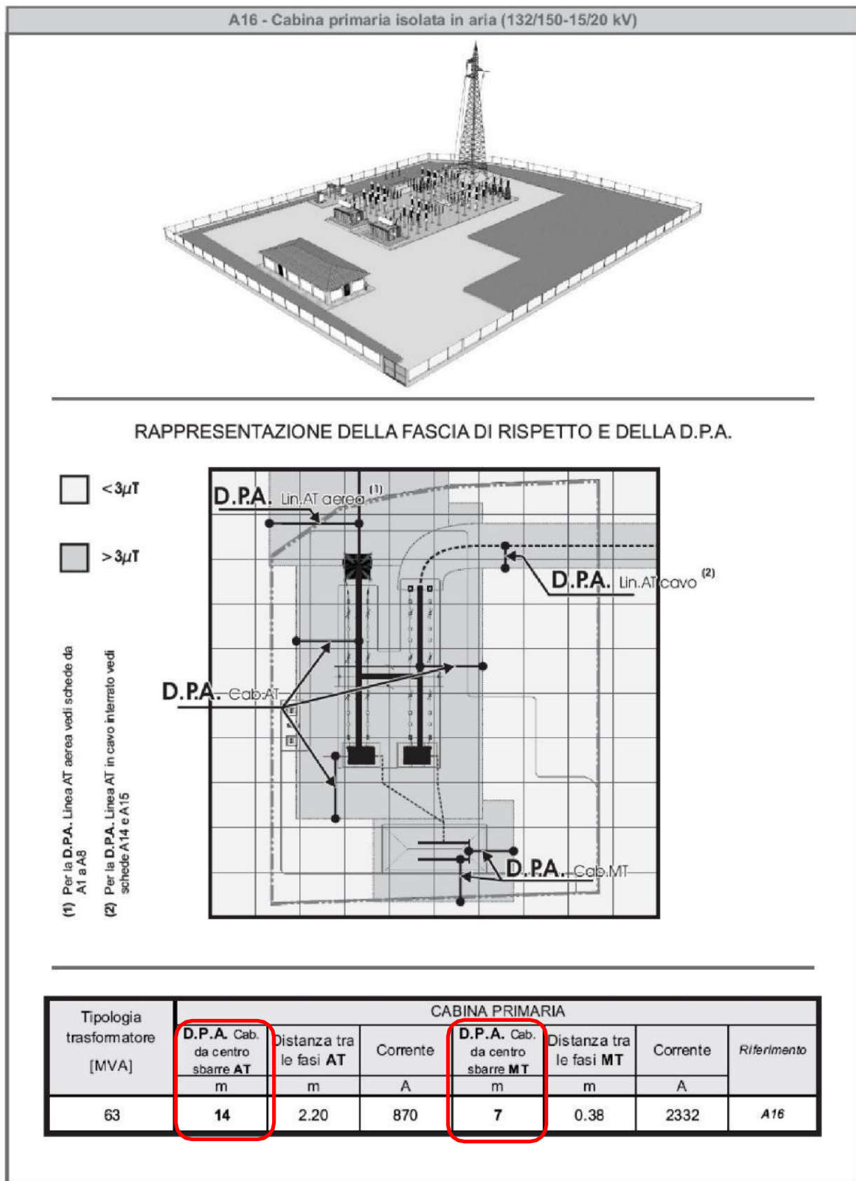
Figura 11 - Stralcio linee guida di Enel sul calcolo della DPA: sottostazioni di trasformazione in alta tensione
