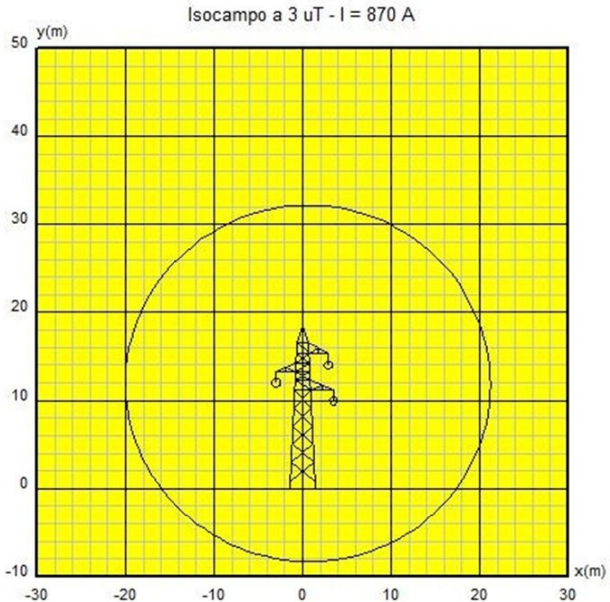
Figura 14 - Obiettivo di qualità valore di campo magnetico
