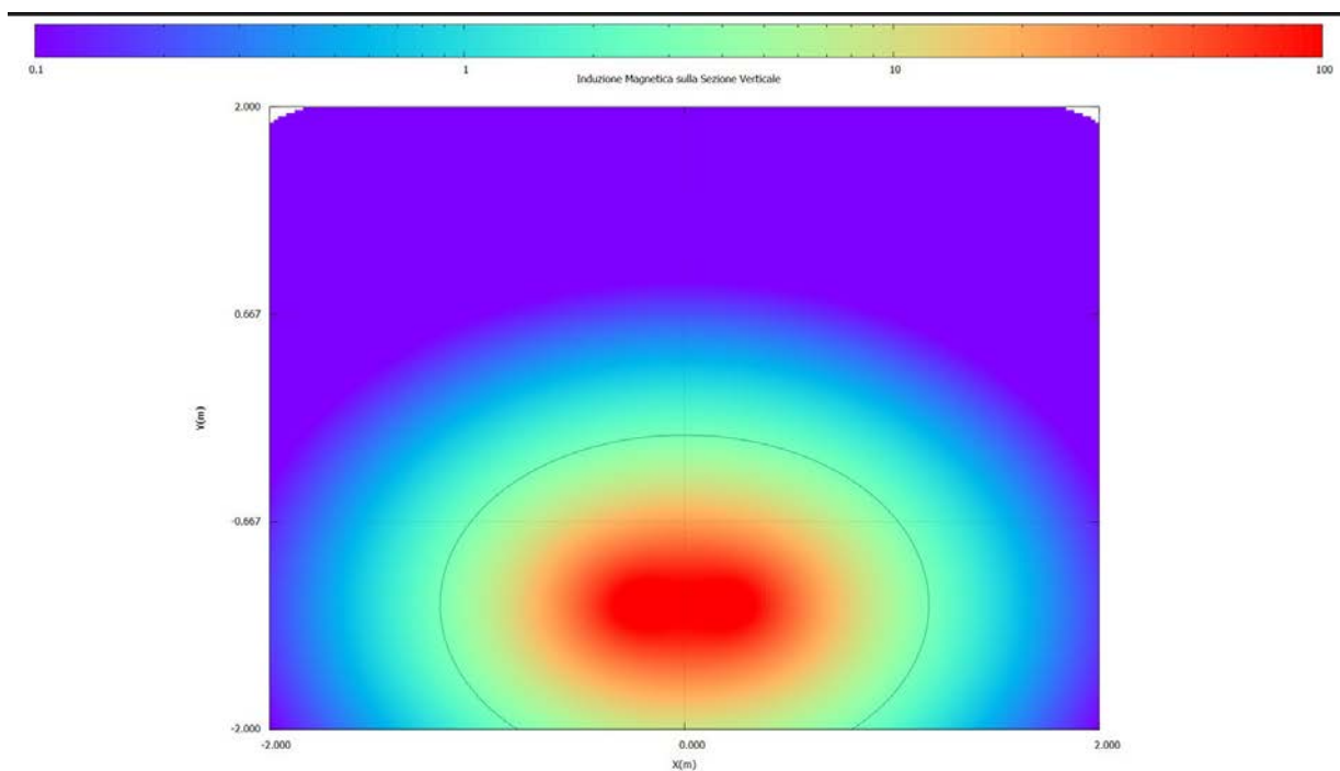
Figura 5 - Mappa a colori induzione magnetica con isocline 3 \mu T
