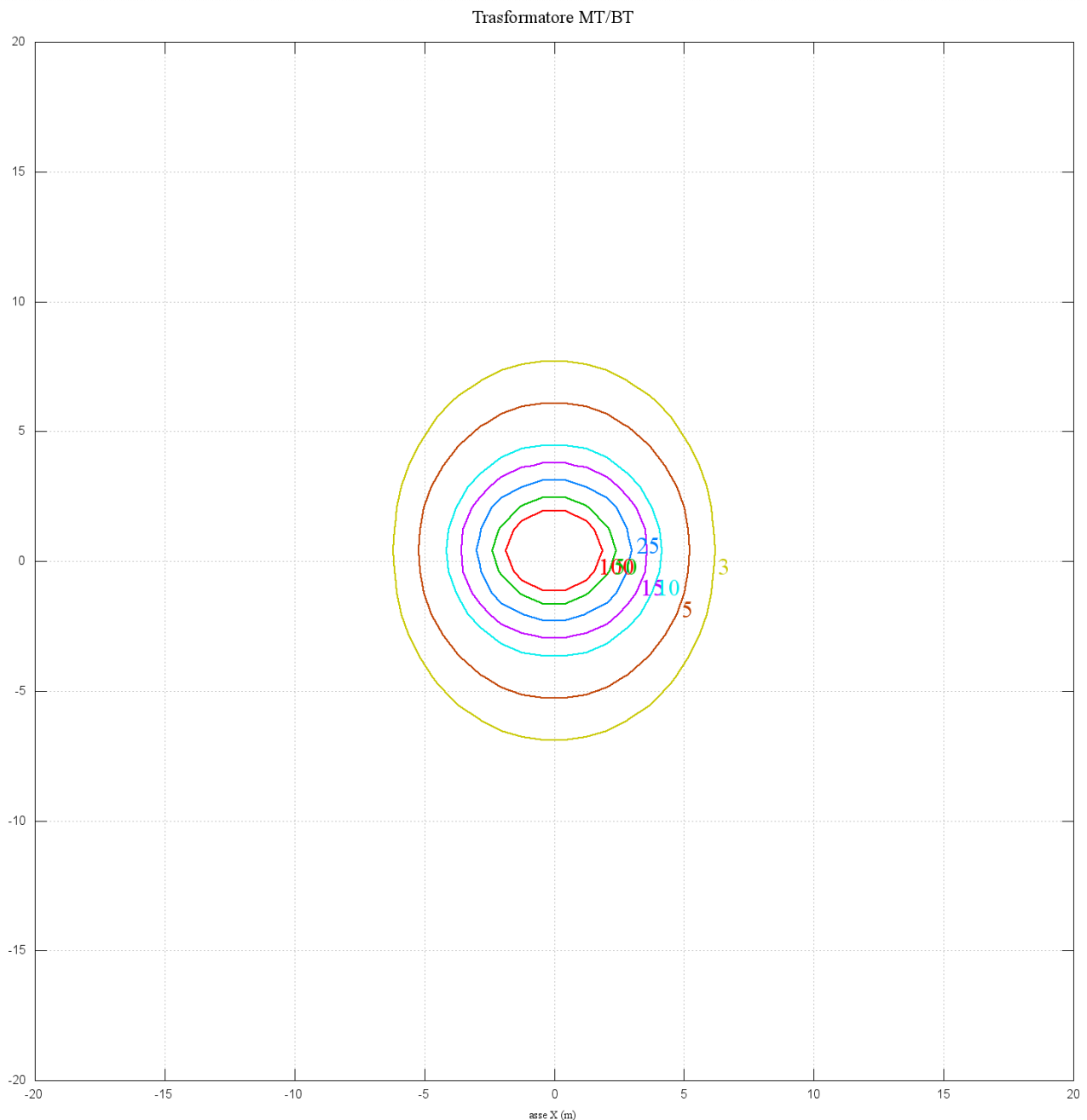
Figura 9 - valori dell'induzione magnetica
