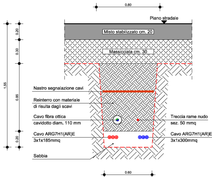
Figura 2 - Tipici cavi MT interrati
