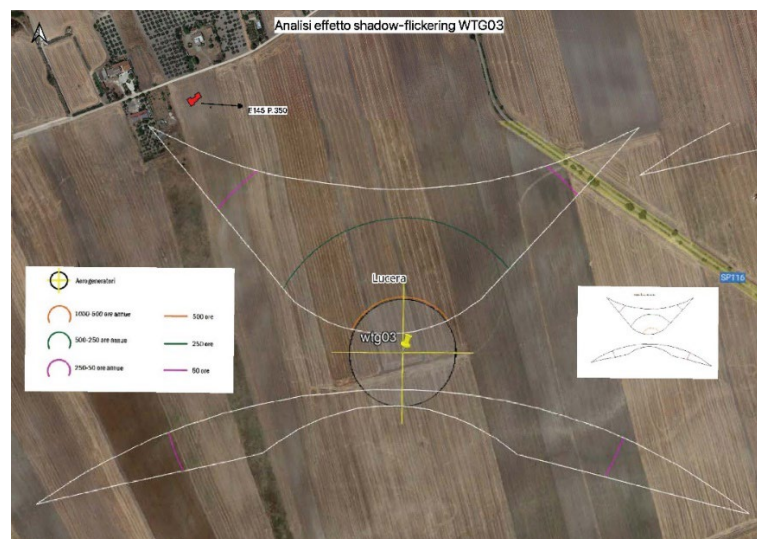
Figura 1 - Analisi Effetto Shadow Flickering WTG03
