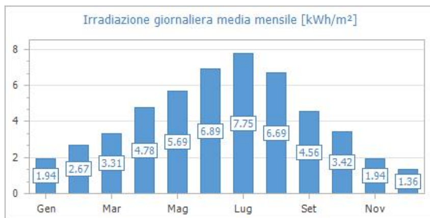
Fig. 1: Irradiazione giornaliera media mensile sul piano orizzontale [kWh/m 2 ]- Fonte dati: UNI 10349:2016 - Stazione di rilevazione: Matera
