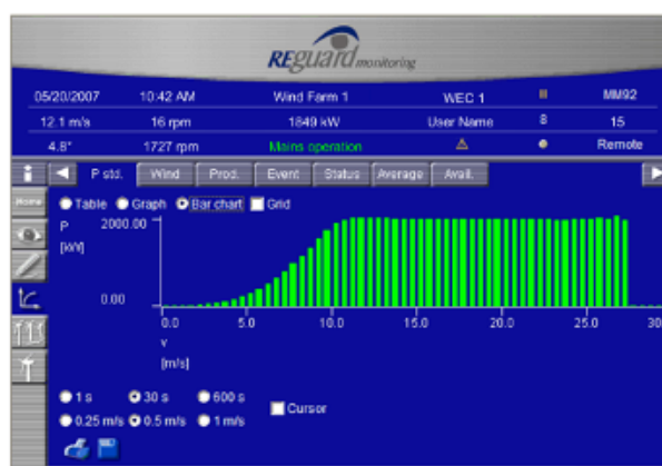
Figura 3 SCADA – Visualizzazione Curva di Potenza – Velocità.
