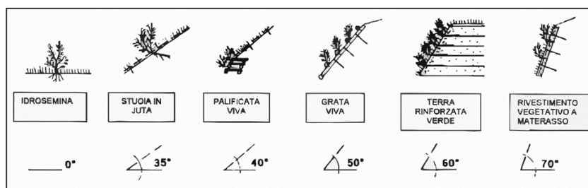
Figura 1 Opere di ingegneria naturalistica distinte per pendenza
