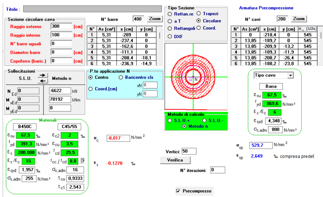
Figura 21 - Fatica massimi
