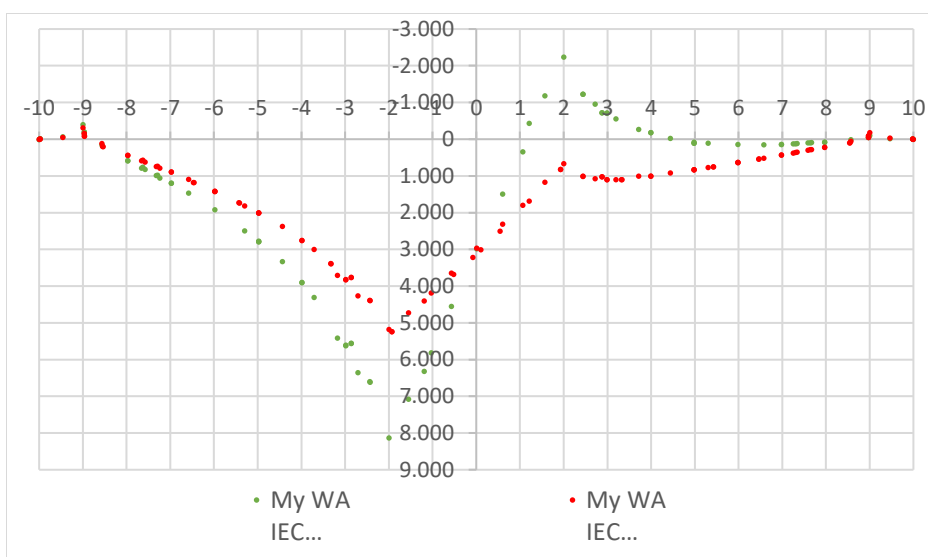
Figura 31 - Momento radiale agente sulla fascia di fondazione (KN m)
