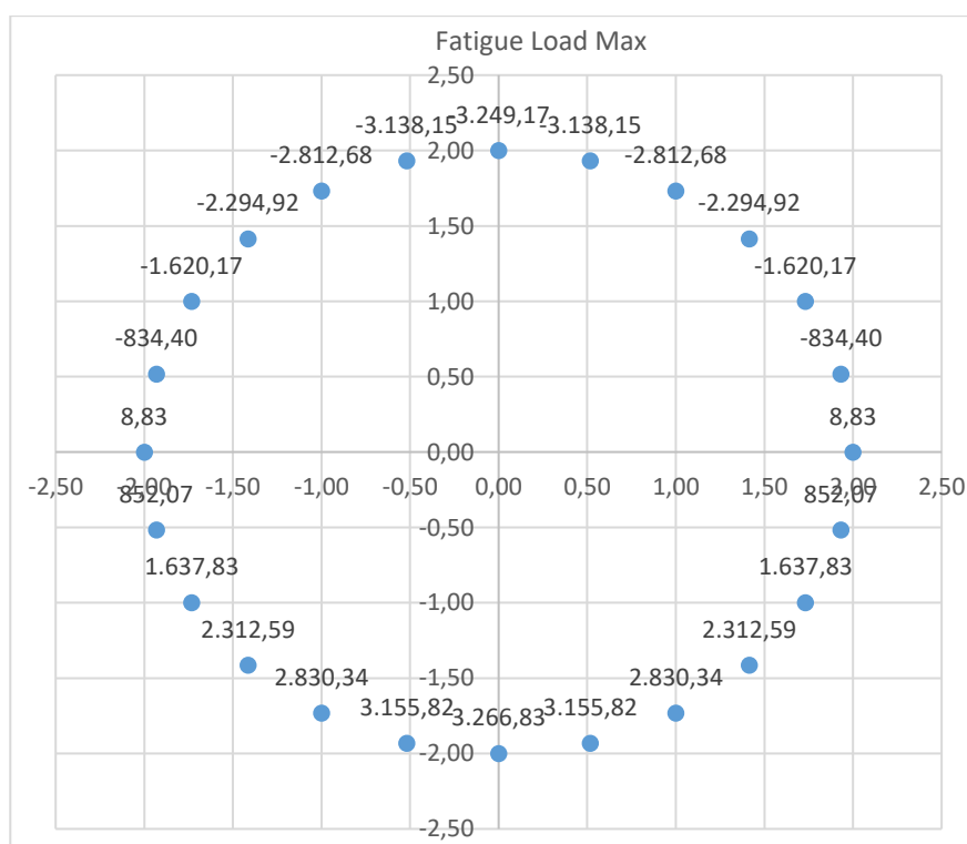
Figura 14 - Distribuzione delle azioni agenti
