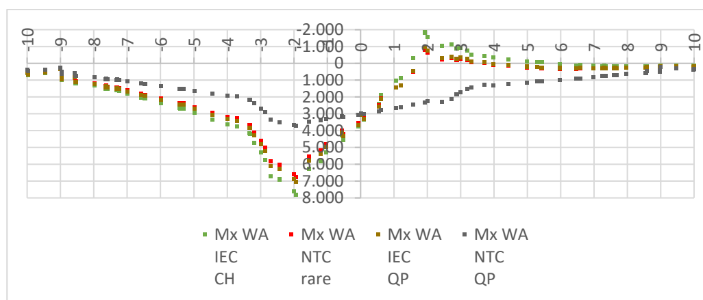
Figura 30 - Involuppo del momento circonferenziale agente sulla fascia di fondazione (KN m)
