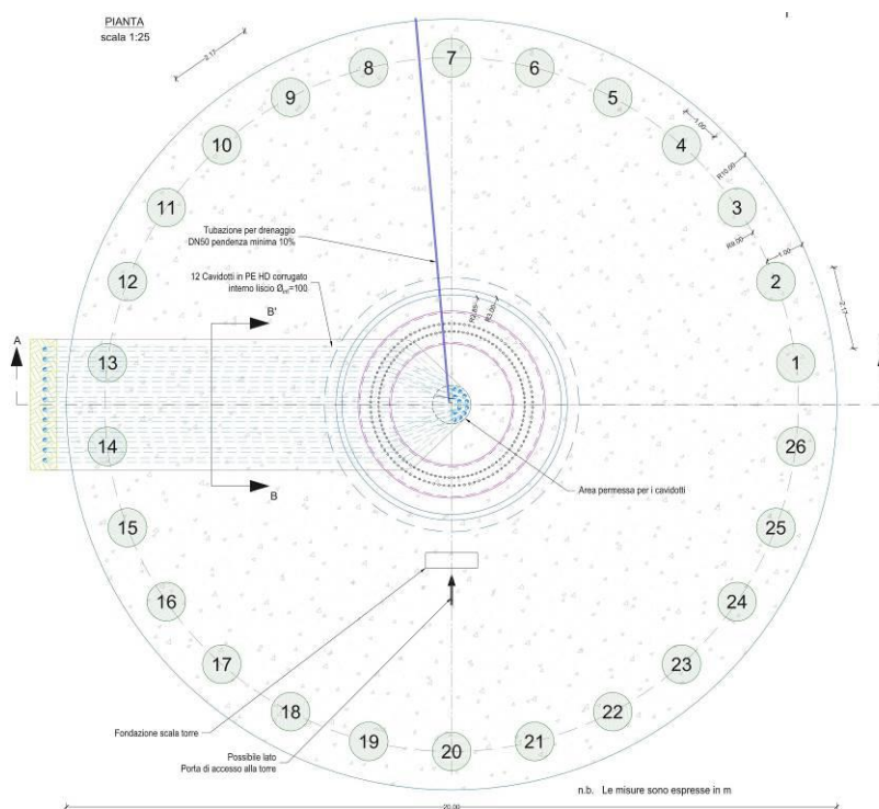
Figura 1 - Pianta del plinto con indicazione dei pali di fondazione (n.26 del diametro 100 cm)
