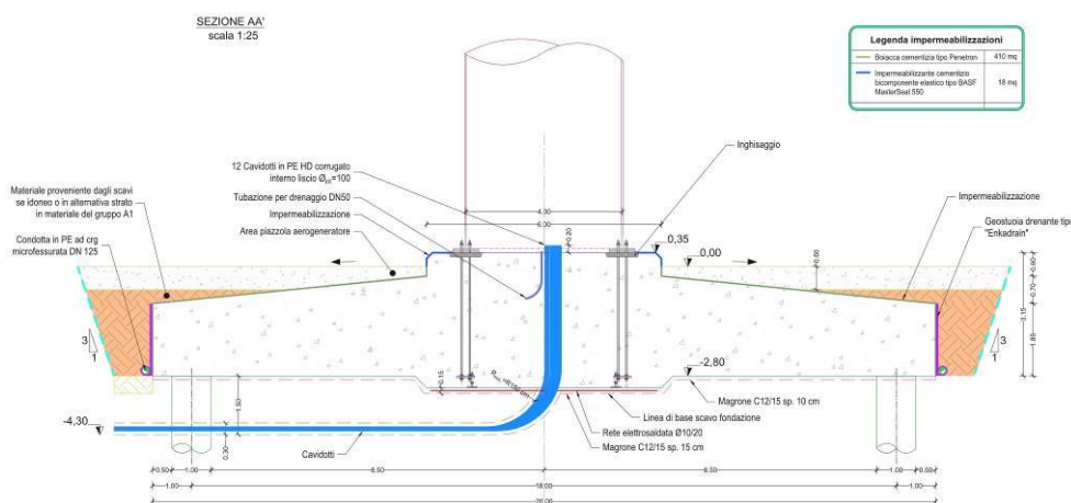
Figura 2 - Sezione del plinto
