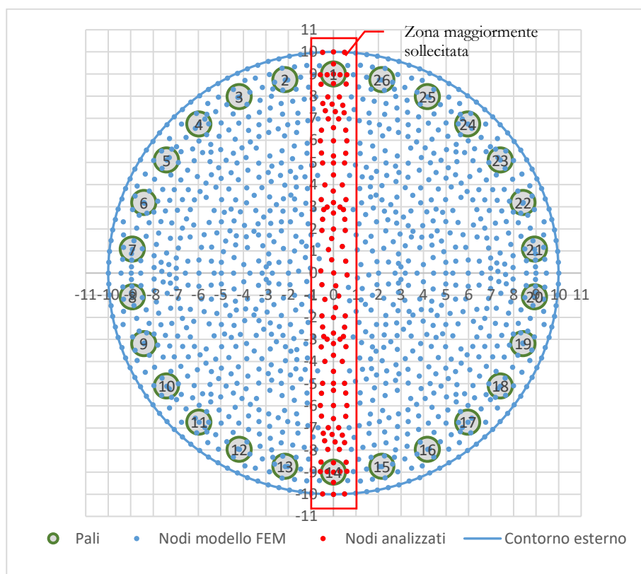
Figura 25 - Individuazione delle zone maggiormente sollecitate
