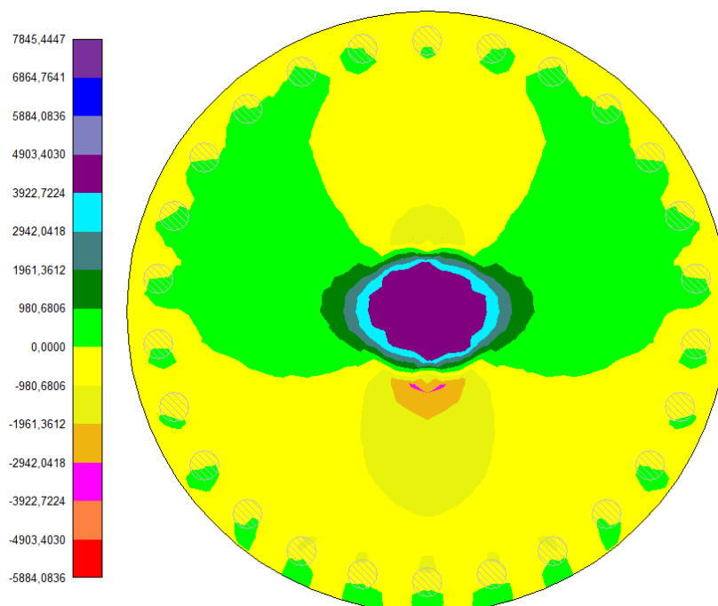
Figura 24 - Distribuzione del taglio T_y (kN) nella piastra di fondazione
