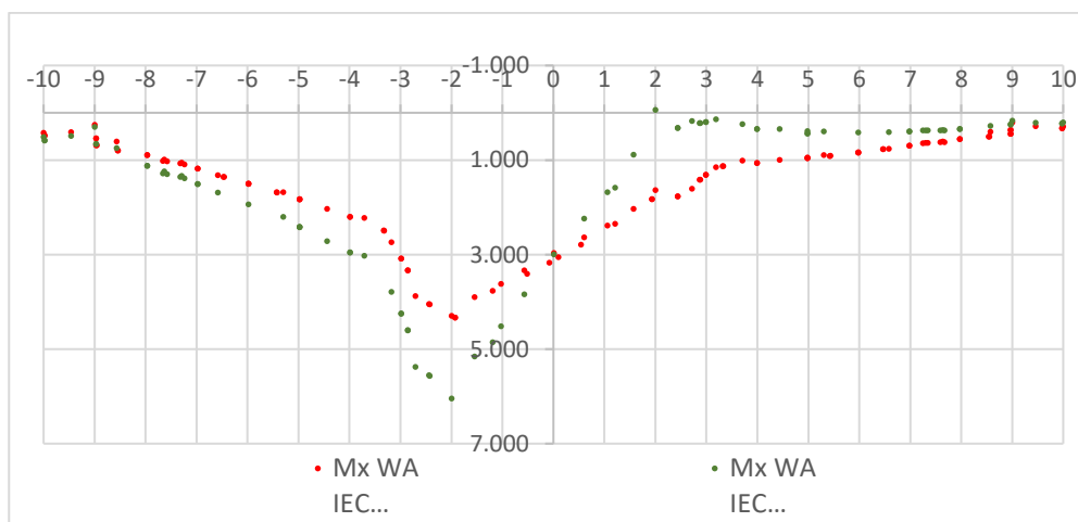
Figura 32 - Momento circonferenziale agente sulla fascia di fondazione (KN m)
