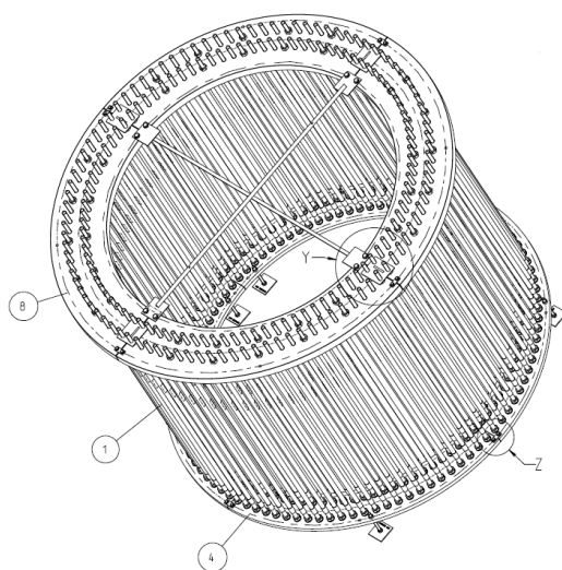
Figura 3 - Vista isometrica d'insieme
