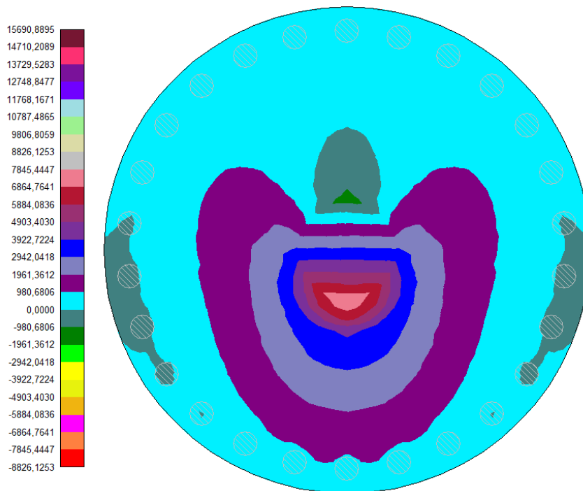
Figura 23 - Distribuzione del momento M_x (kN m) nella piastra di fondazione
