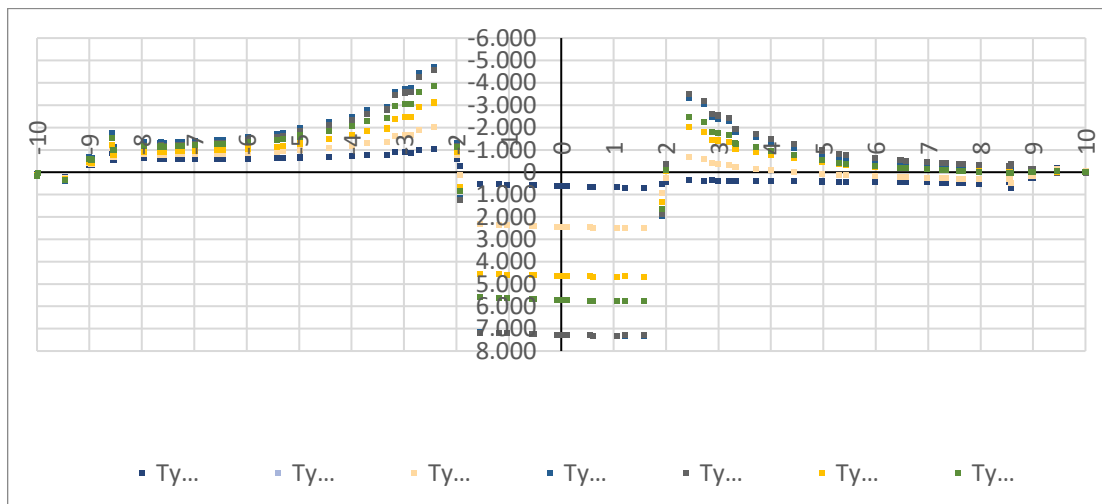
Figura 28 - Inviluppo del taglio agente sulla fascia di fondazione (KN)
