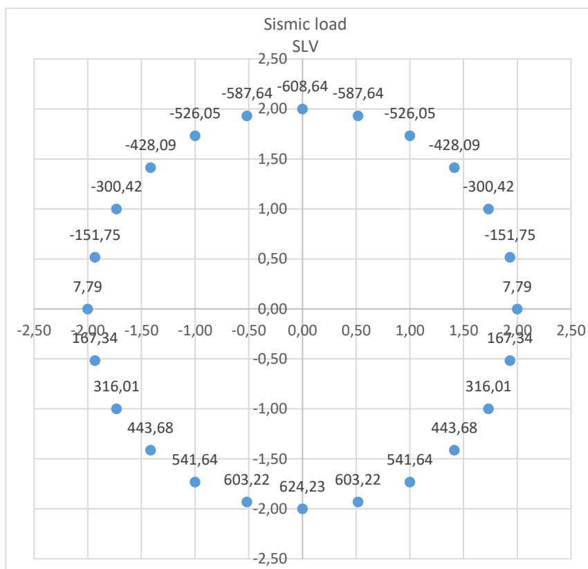
Figura 10 Distribuzione delle azioni agenti
