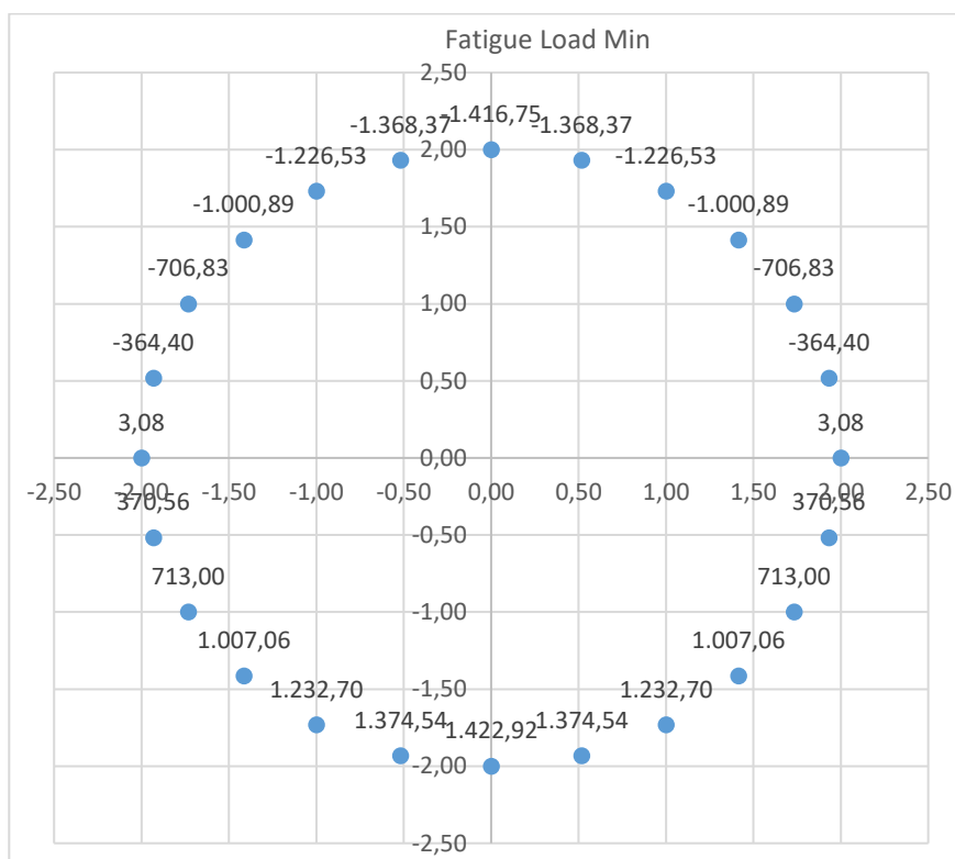
Figura 13 - Distribuzione delle azioni agenti
