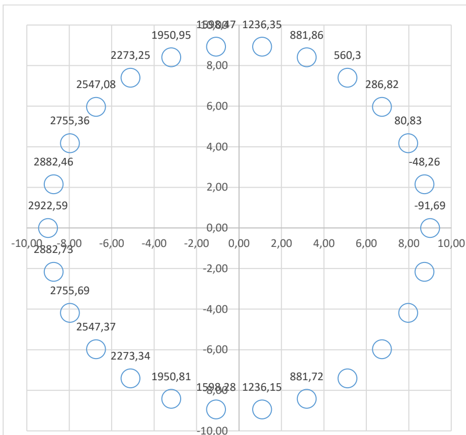
Figura 41 - distribuzione delle azioni agenti
