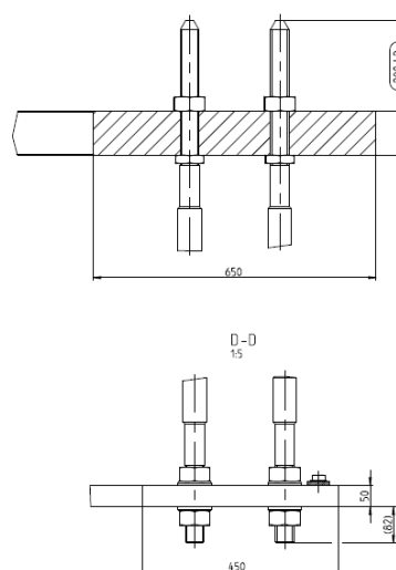
Figura 4 - Sezione verticale
