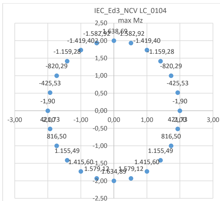
Figura 7 -distribuzione delle azioni agenti
