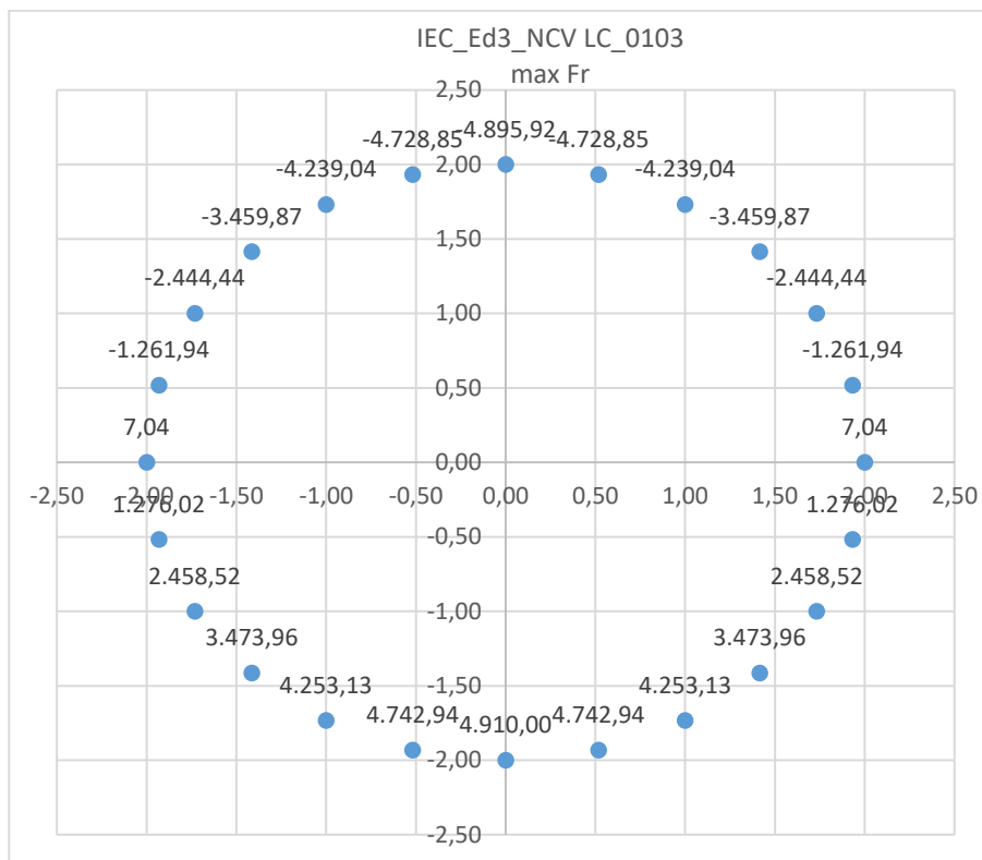
Figura 6-distribuzione delle azioni agenti
