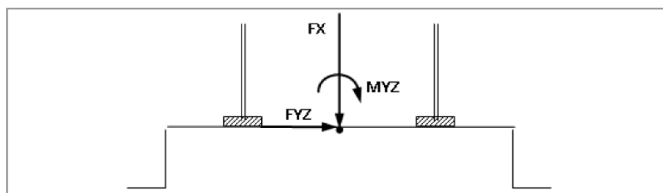
Figura - 5 Sistema di riferimento delle azioni
