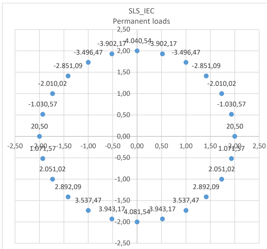
Figura 12 - Distribuzione delle azioni agenti
