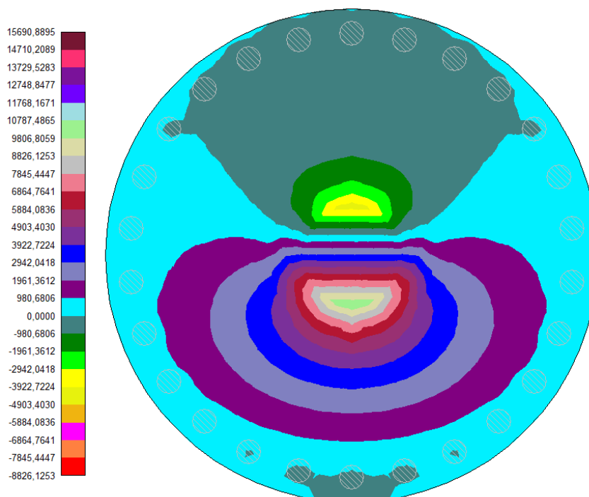
Figura 22 - Distribuzione del momento M_y (KN m) nella piastra di fondazione – COMB 12
