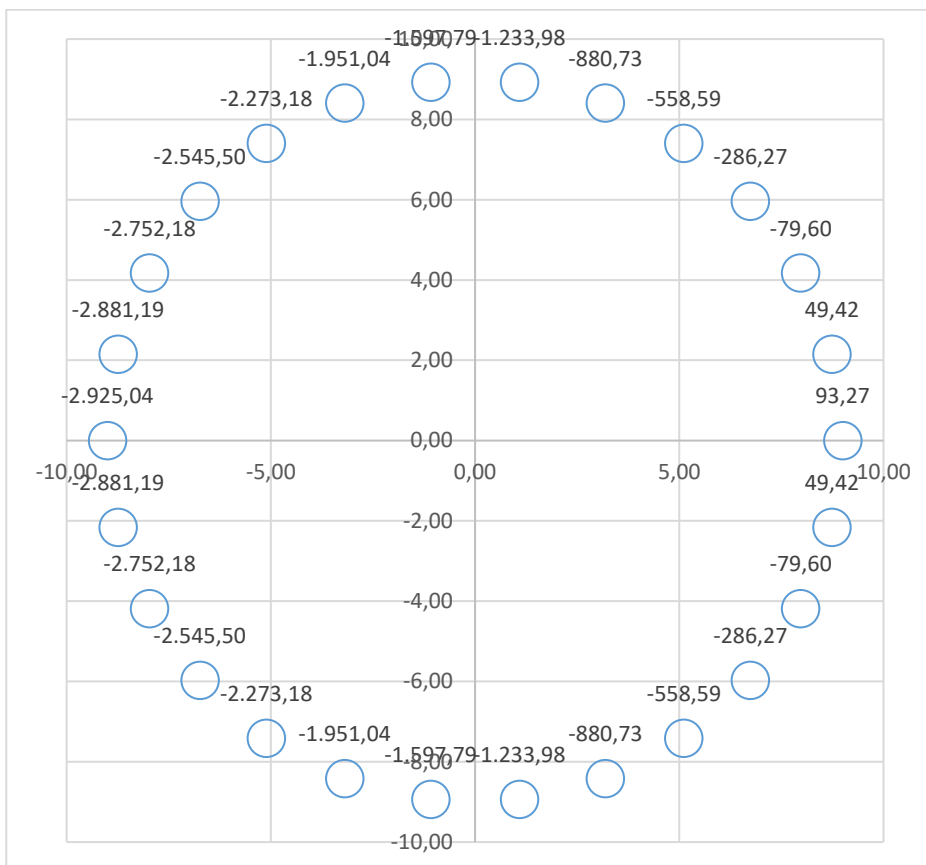
Figura 40 - distribuzione delle azioni agenti
