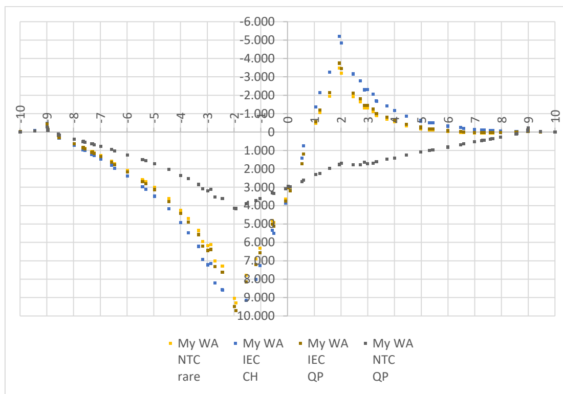
Figura 29 - Involuppo del momento radiale agente sulla fascia di fondazione (KN m)
