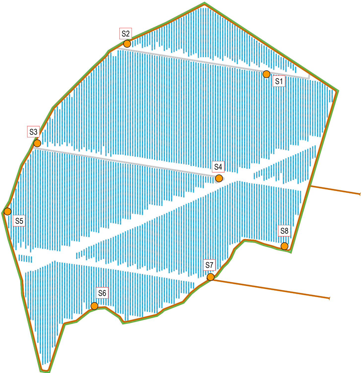
Fig. 3: campo agrivoltaico con posizione delle cabine di trasformazione ●
