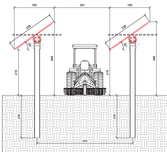
Figura 8 – Sezione tracker con relative posizioni Lotto 1
