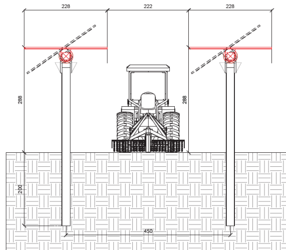
Figura 8 – Sezione tracker con relative posizioni Lotto 1
