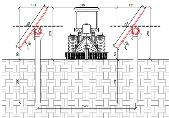
Figura 9 – Sezione tracker con relative posizioni Lotto 2
