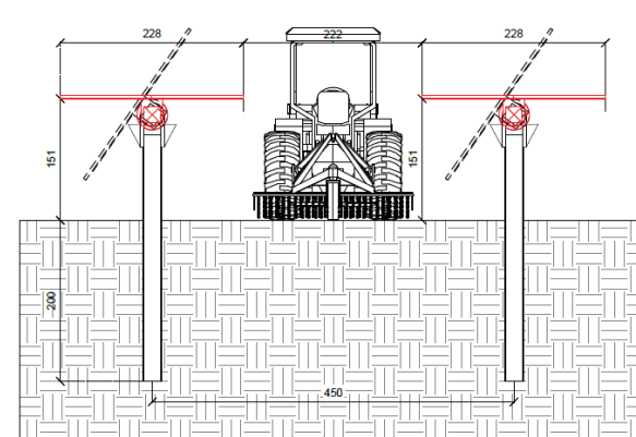
Figura 9 – Sezione tracker con relative posizioni Lotto 2
