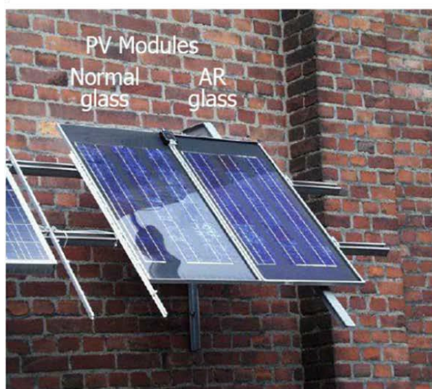
Figura 2. Le due immagini dimostrano come, al contrario di un vetro comune, il vetro anti-riflesso ( Anti-Reflecting glass ) che riveste i moduli fotovoltaici riduca drasticamente la riflessione dei raggi luminosi
