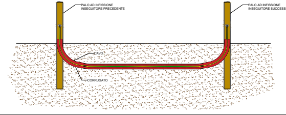
SCHEMA DI COLLEGAMENTO TRA STRUTTURE ADIACENTI
