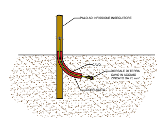
SCHEMA DI COLLEGAMENTO TRA STRUTTURE ADIACENTI
