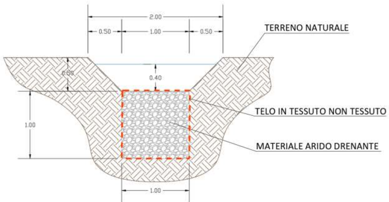
Figura 6.1 - Sezione trasversale sistema fossi + trincee
