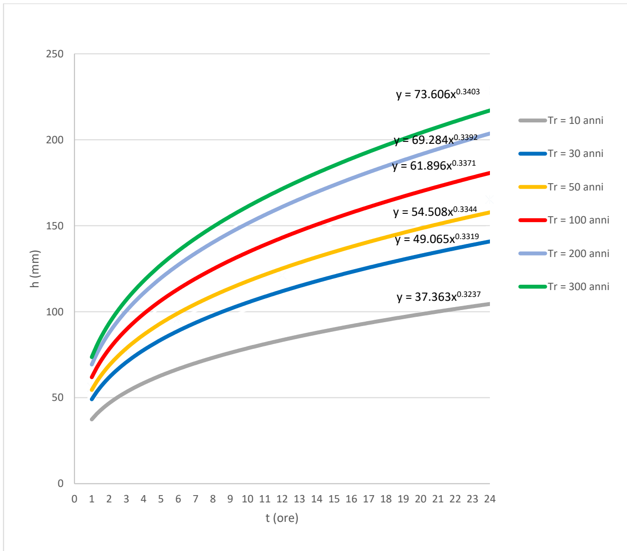
Figura 5.4 – Curve di probabilità pluviometrica (Stazione di Paternò)
