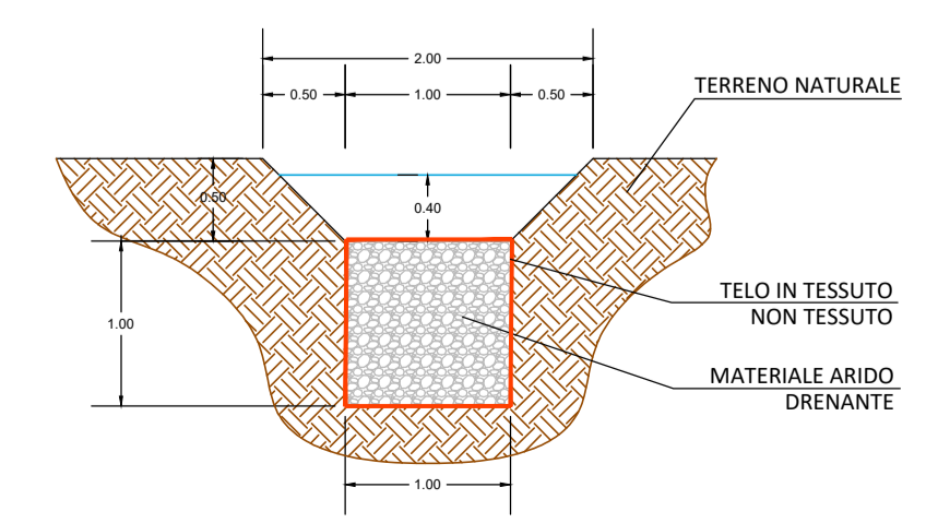
SEZIONE TRASVERSALE SISTEMA FOSSO DI GUARDIA CON TRINCEA DRENANTE Scala 1:50
