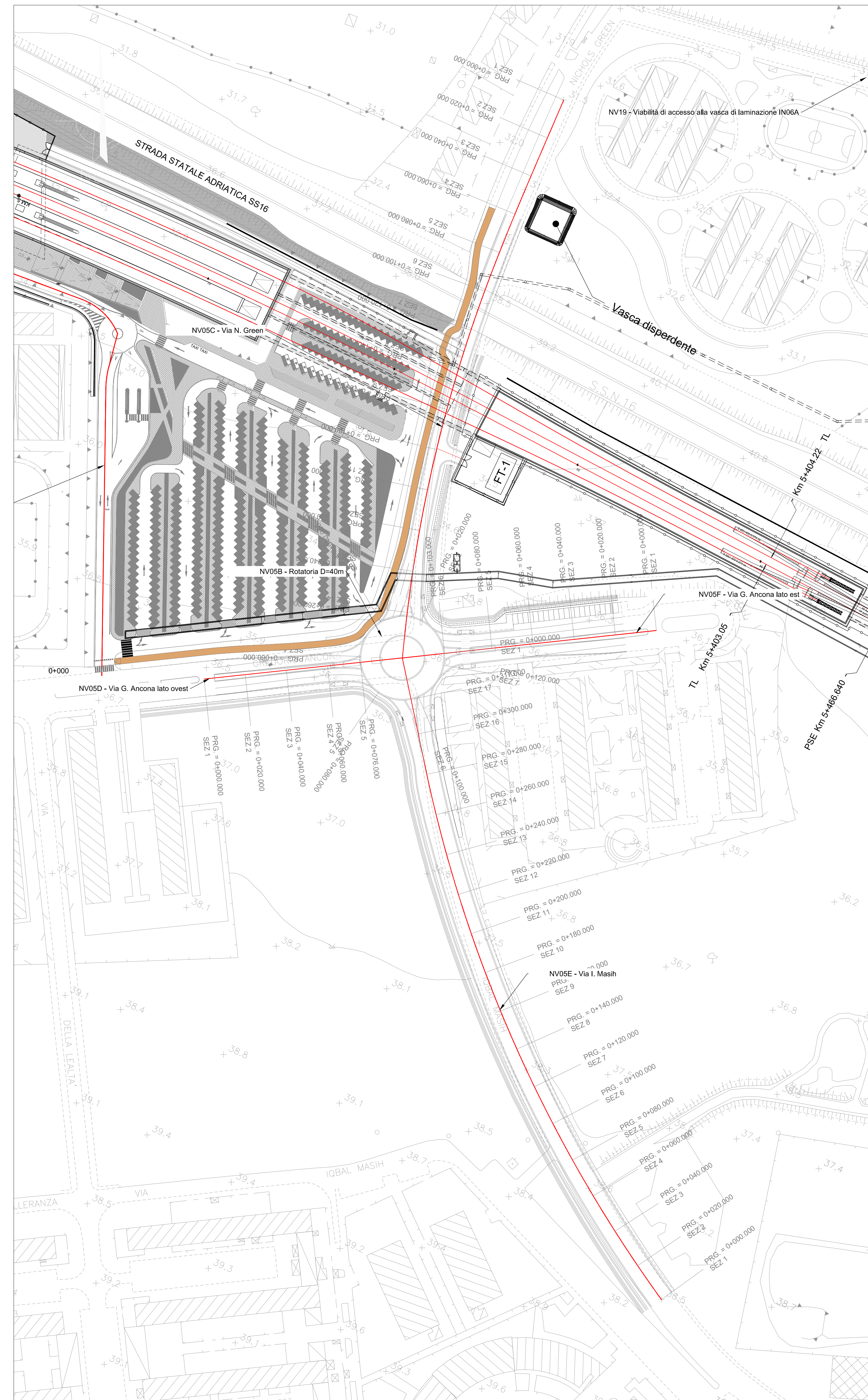
PLANIMETRIA DI PROGETTO SU CARTOGRAFIA
