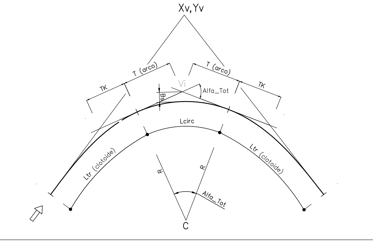
SCHEMA ESPLICATIVO TABELLA CURVE PLANIMETRICHE
