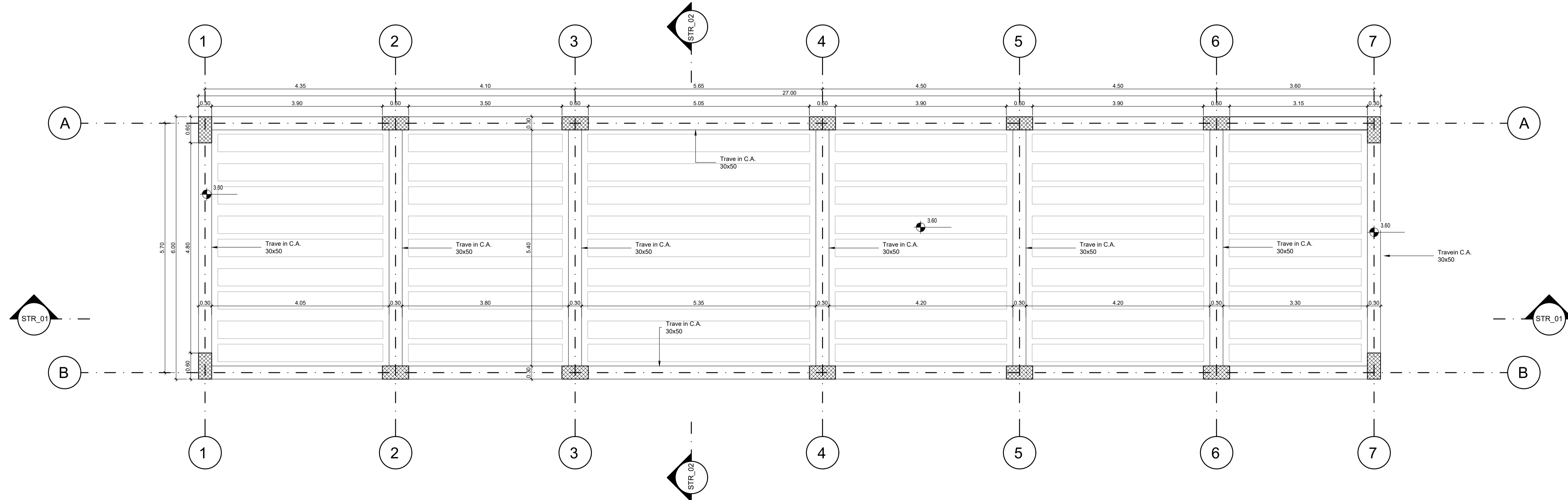
Carpenteria coperture Scala 1:50
