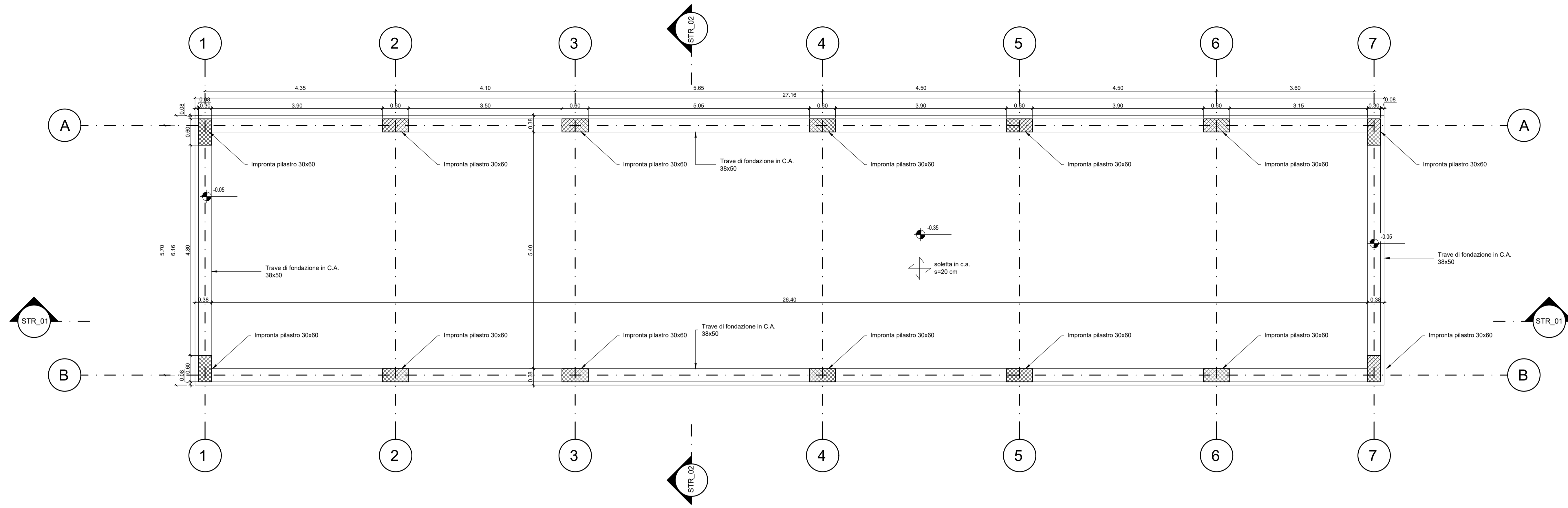
Carpenteria fondazioni Scala 1:50
