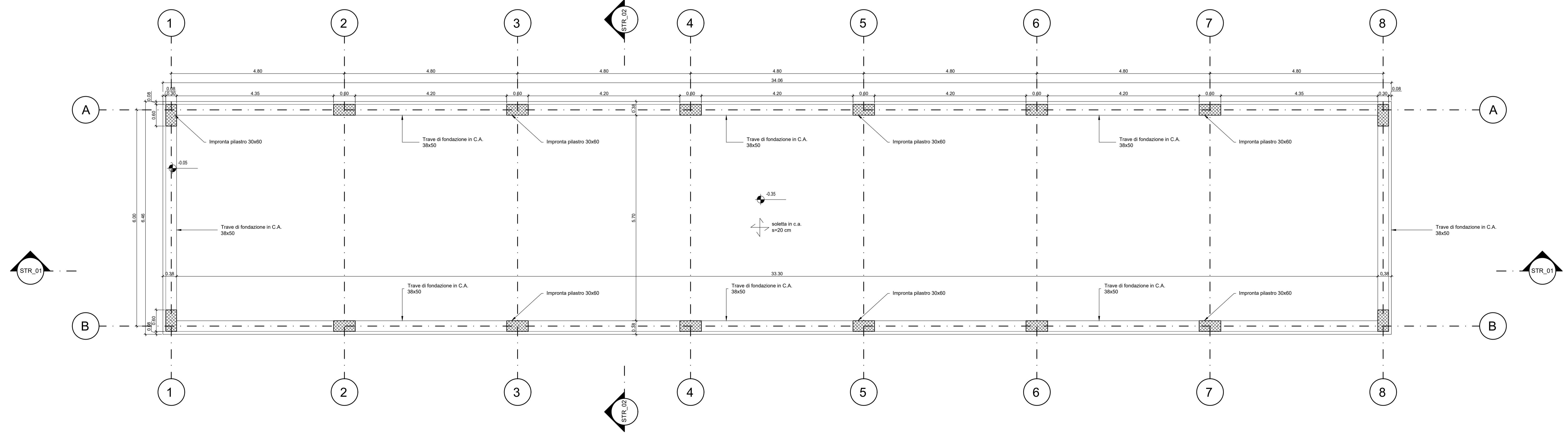
Pianta copertura Scala 1:50
