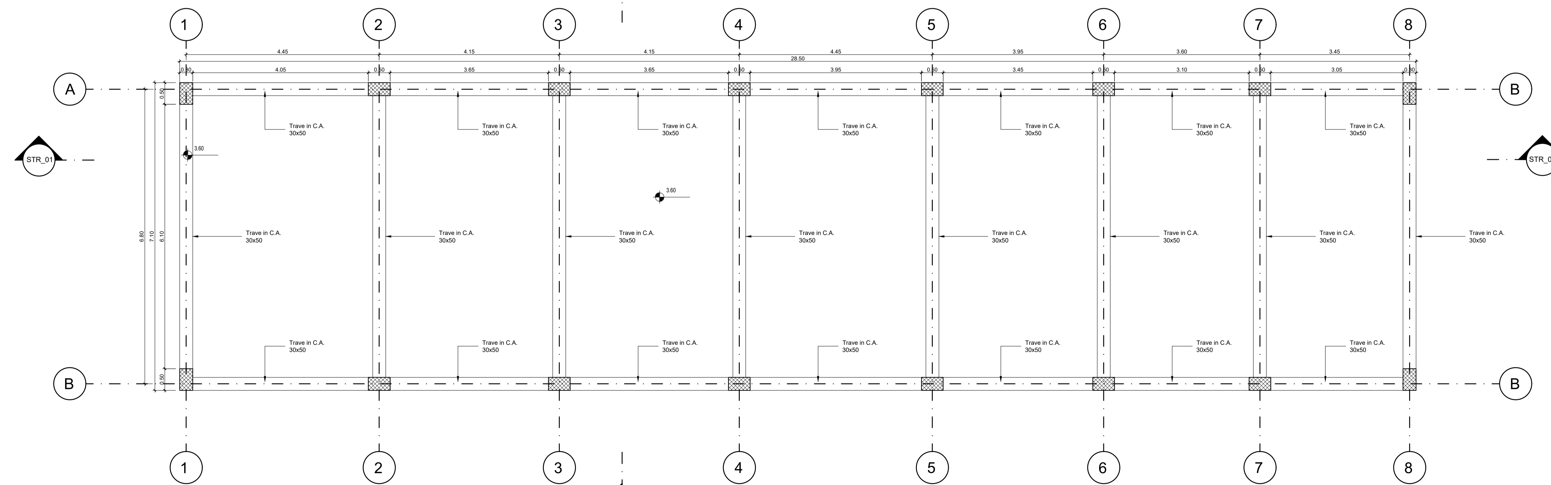
Pianta coperture Scala 1:50
