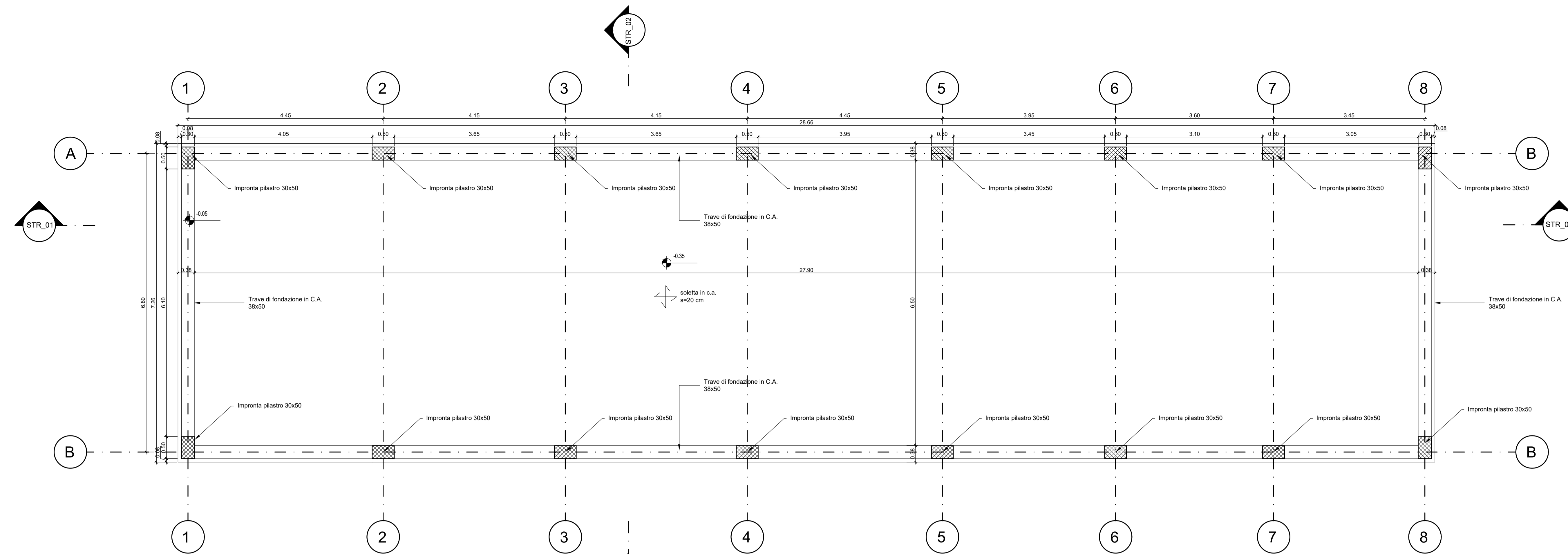
Pianta fondazioni Scala 1:50
