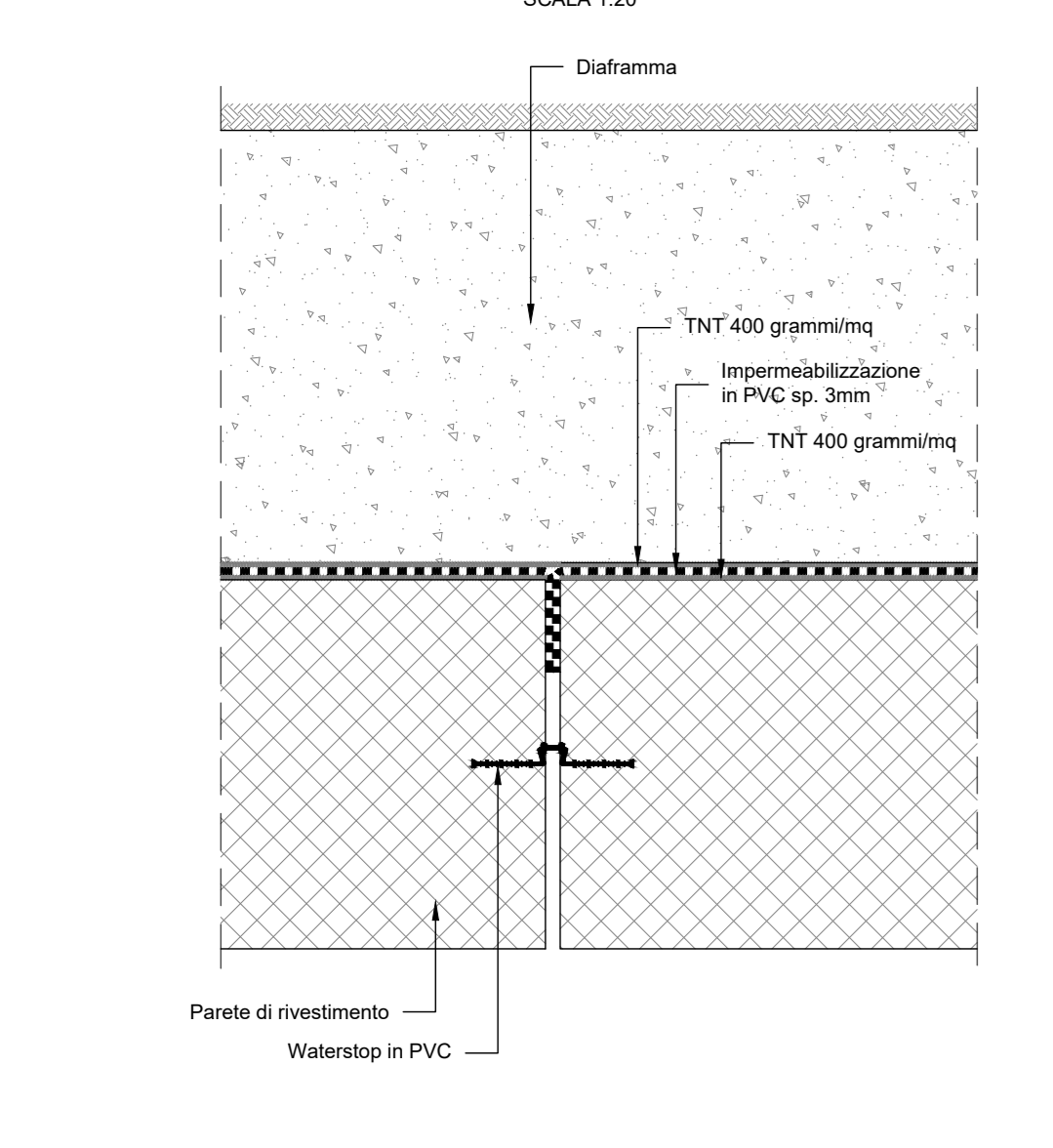
GIUNTO DI PARETE CONTRO DIAFRAMMI SCALA 1:20
