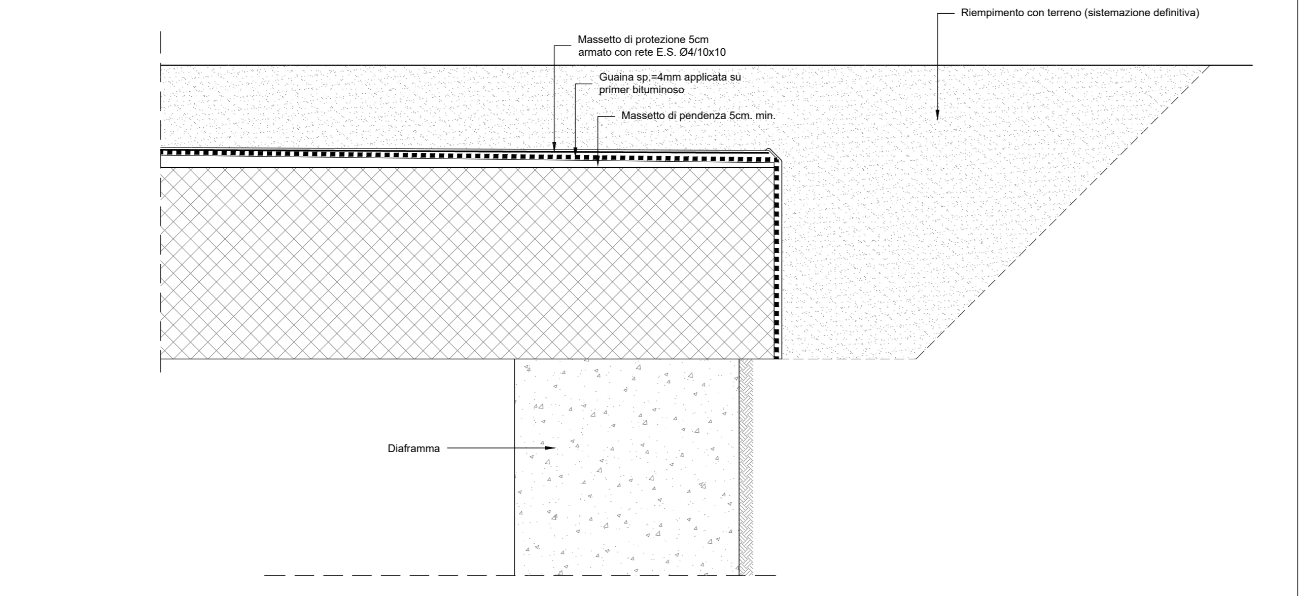
DETTAGLIO IMPERMEABILIZZAZIONE SOLETTA DI COPERTURA E PARETE SCALA 1:20
