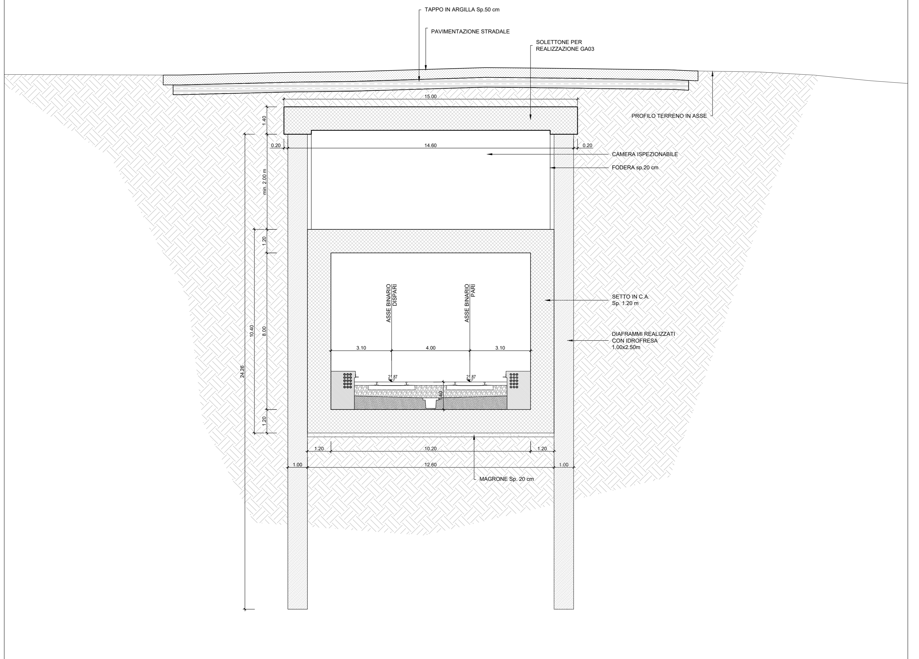
SEZIONE TRASVERSALE A-A SCALA 1:100
