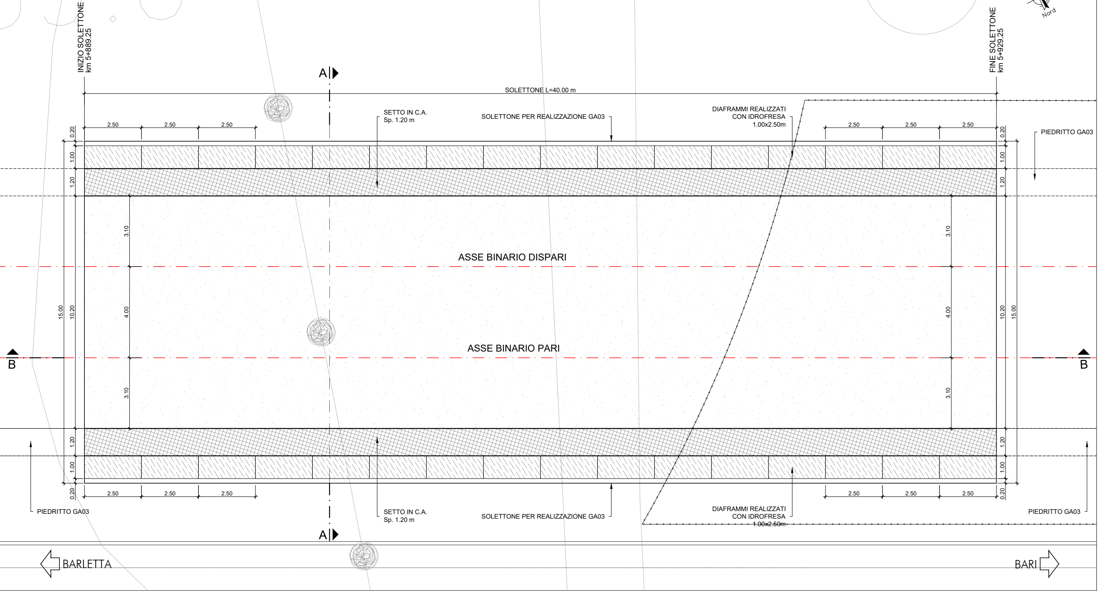
VISTA ESTRADOSSO SOLETTA DI FONDO SCALA 1:100
