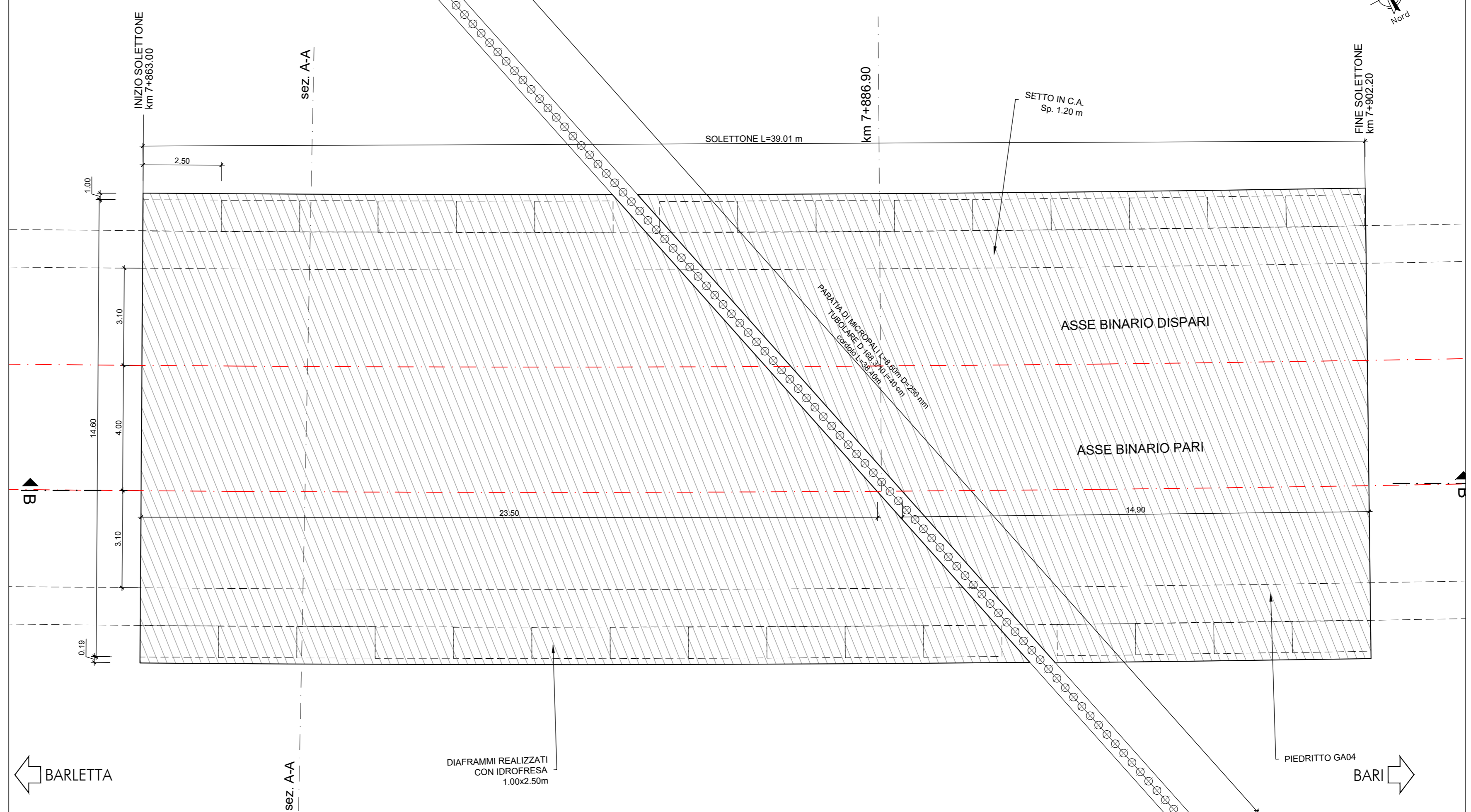
VISTA DALL'ALTO SCALA 1:100
