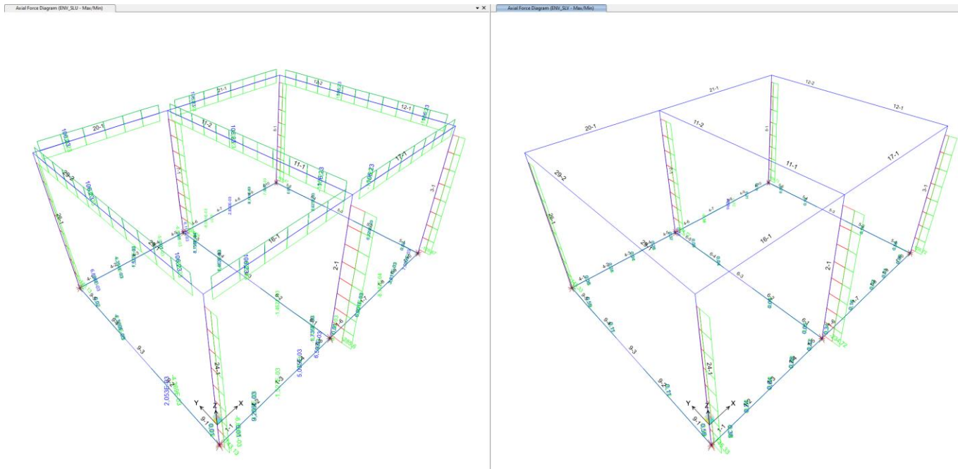
Figura 7-5 -Diagramma N – Combinazione “ENV_SLU” (sx) e “ENV_SLV” (dx)
