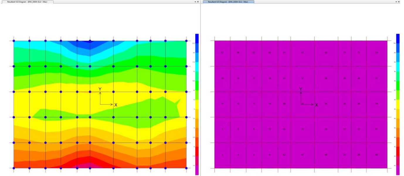
Figura 11: ENV_max_SISM+SLU (sx) e Diagramma di ricoprimento (dx)- V23
