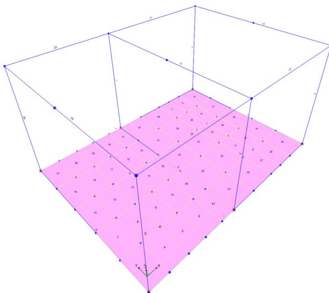
Figura 7-2 - Modello di calcolo – numerazione frames e nodi.
