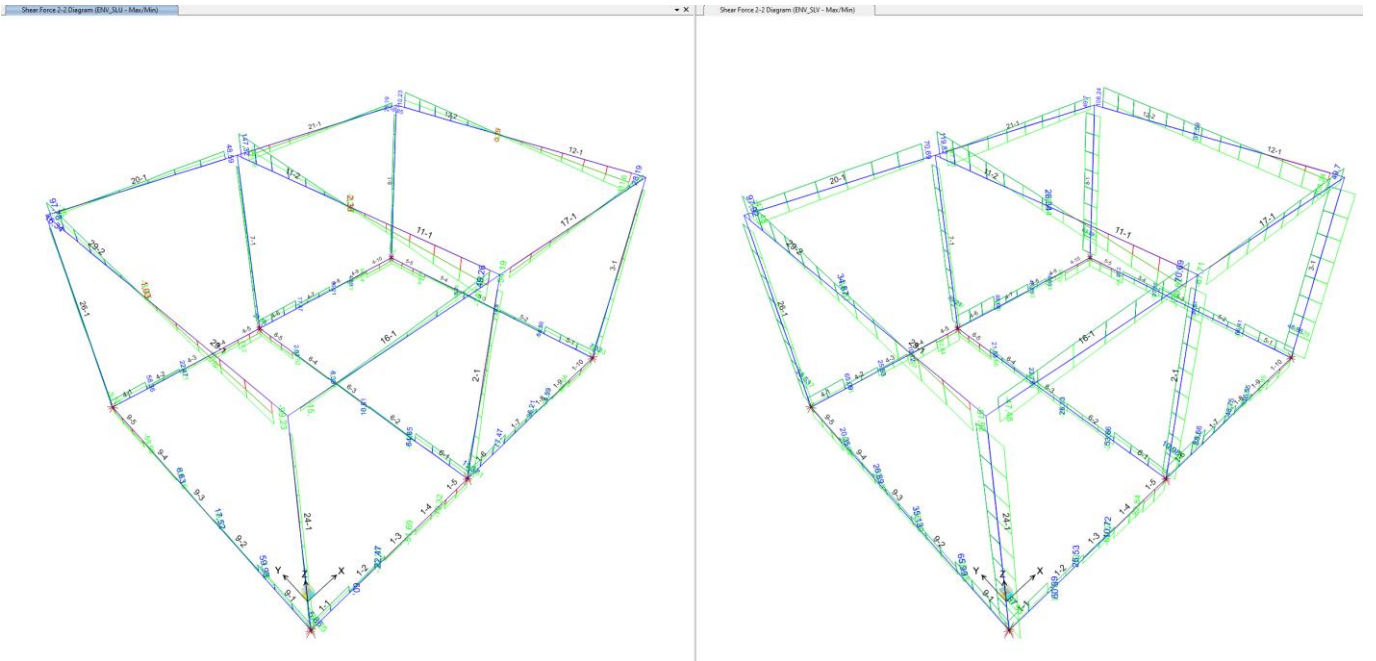
Figura 7-4 - Diagramma V22 – Combinazione “ENV_SLU” (sx) e “ENV_SLV” (dx)
