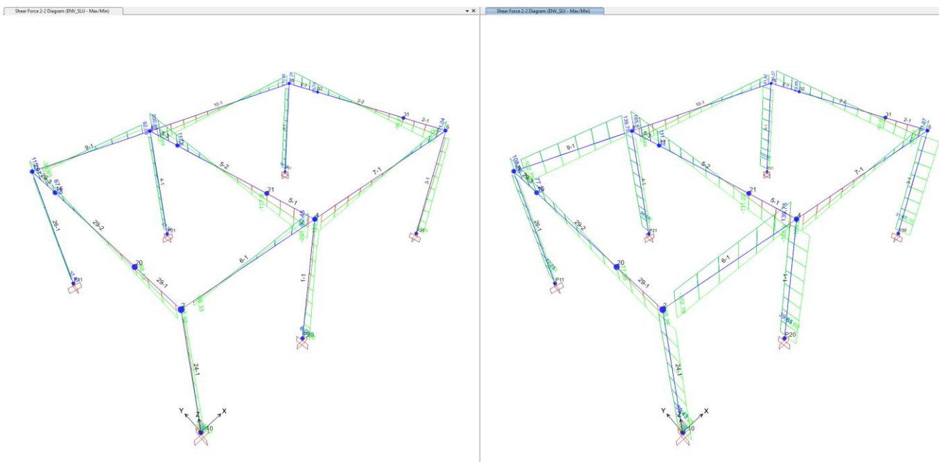
Figura 7-4 - Diagramma V22 – Combinazione “ENV_SLU” (sx) e “ENV_SLV” (dx)
