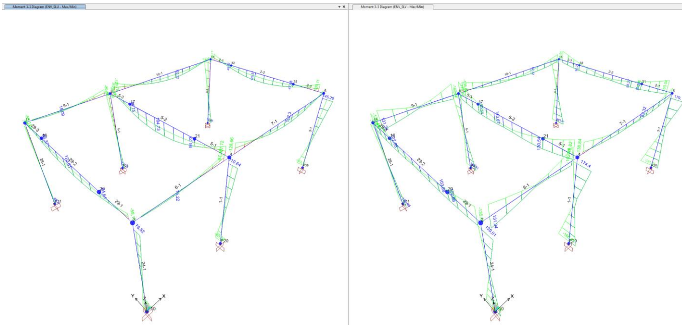
Figura 7-3 - Diagramma M33 – Combinazione “ENV_SLU” (sx) e “ENV_SLV” (dx)
