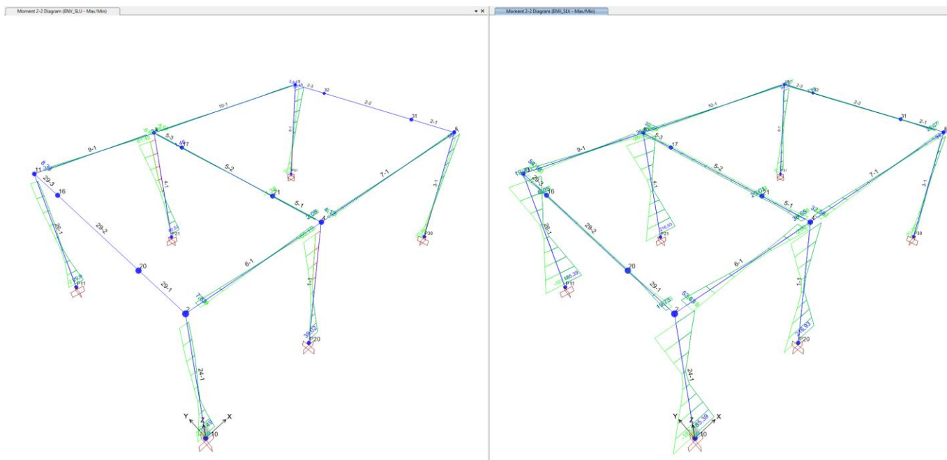
Figura 7-6- Diagramma M22 – Combinazione “ENV_SLU” (sx) e “ENV_SLV” (dx)
