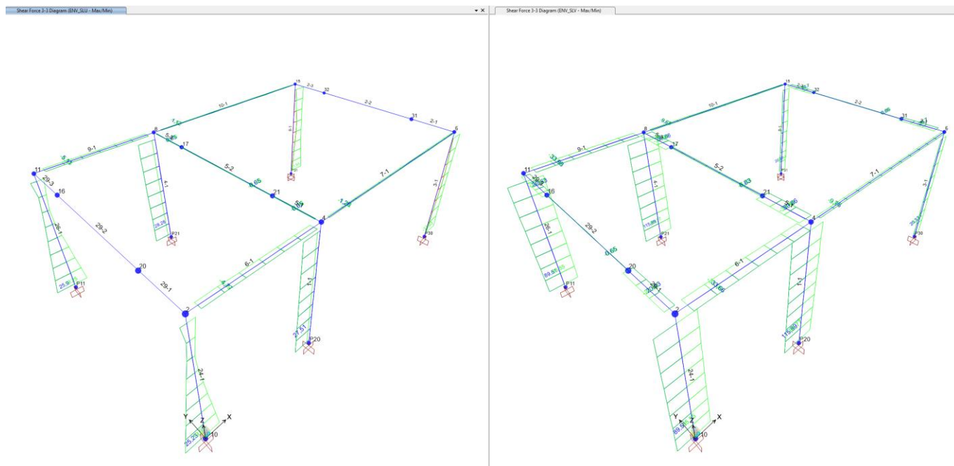
Figura 7-7 Modello di calcolo – Diagramma V33 – Combinazione “ENV_SLU” (sx) e “ENV_SLV” (dx)
