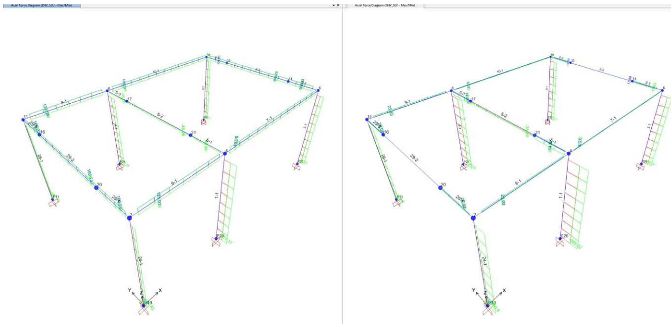
Figura 7-5 -Diagramma N – Combinazione “ENV_SLU” (sx) e “ENV_SLV” (dx)
