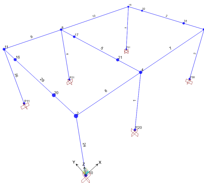
Figura 7-2 - Modello di calcolo – numerazione frames e nodi.
