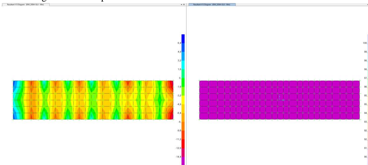
Figura 10: ENV_min_SISM+SLU (sx) e Diagramma di ricoprimento (dx)- V13
