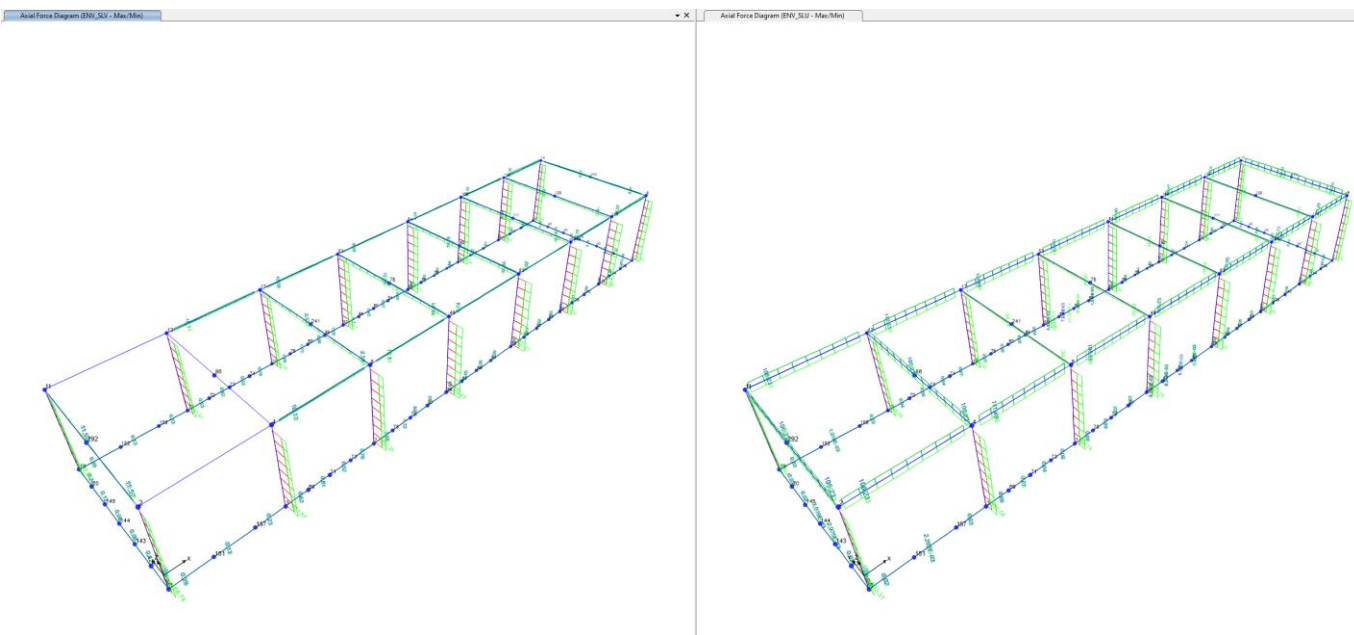
Figura 7-5 -Diagramma N – Combinazione “ENV_SLU” (dx) e “ENV_SLV” (sx)
