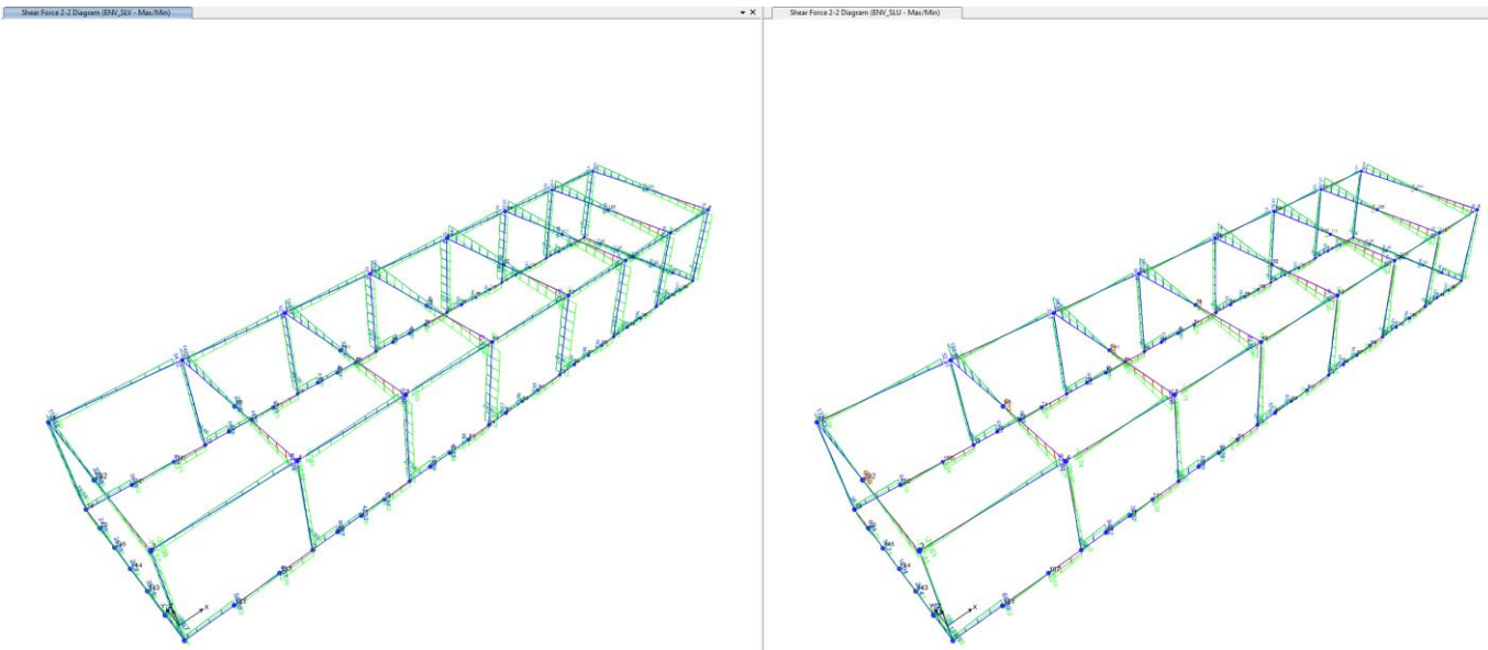
Figura 7-4 -Diagramma V22 – Combinazione “ENV_SLU” (dx) e “ENV_SLV” (sx)
