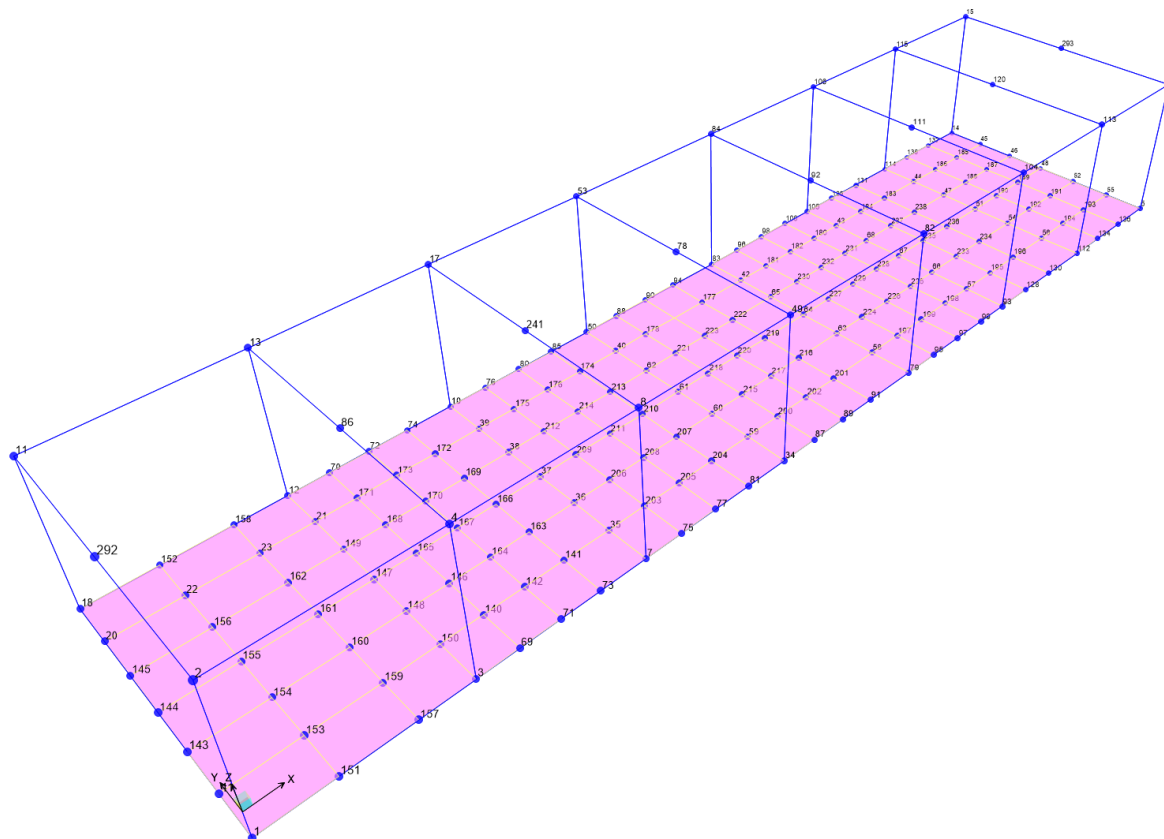
Figura 7-2 - Modello di calcolo – numerazione frames e nodi.
